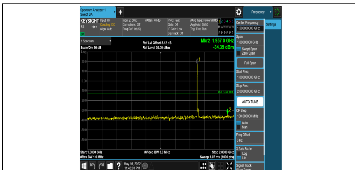
Band4-5MHz-QPSK-20375-1RB#0-Range4:1000~2000MHz
