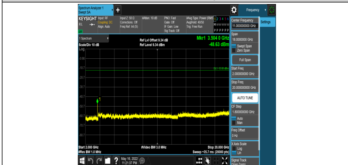
Band4-3MHz-QPSK-20385-1RB#0-Range5:2000~20000MHz
