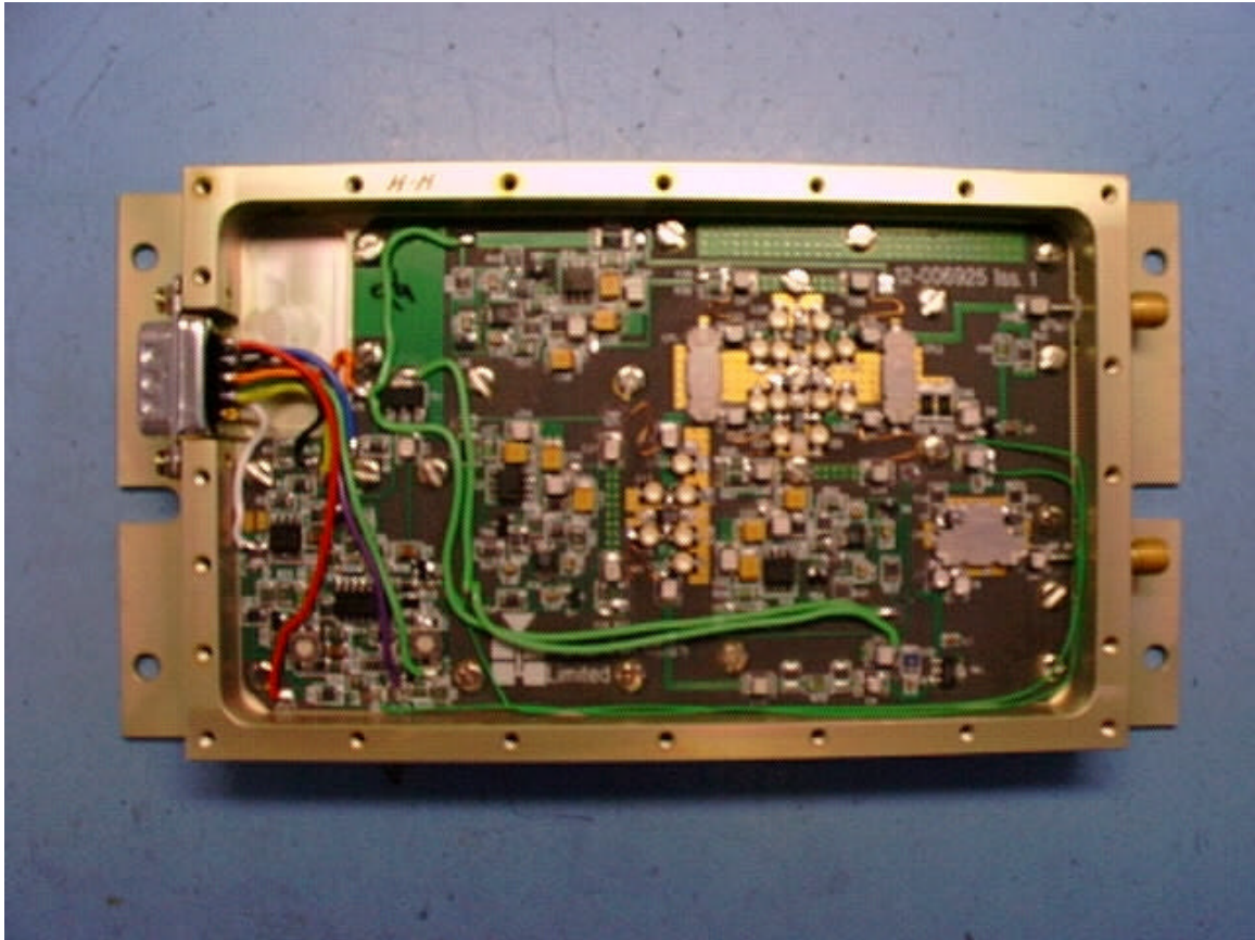
Photo 17 - PA module
