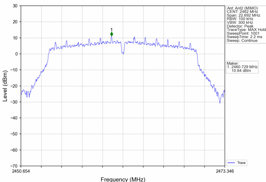
802.11g_HCH_2462MHz_Ant2 (MIMO)_NTNV
