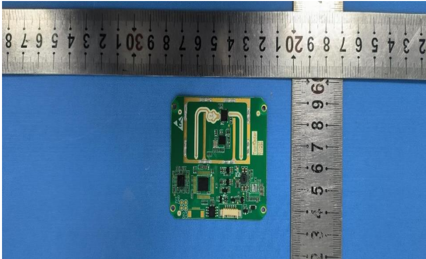
24G Radar Module: TR24DCA100
