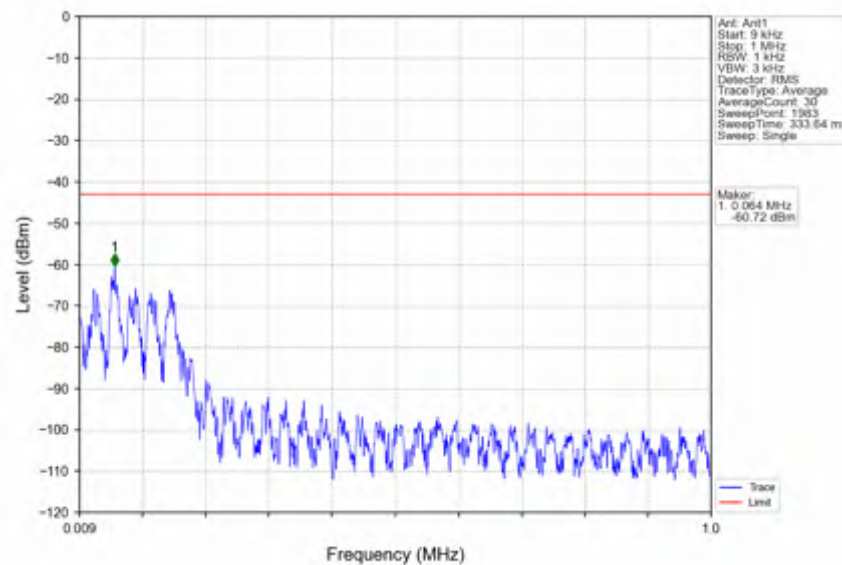
n41_15kHz_SISO_NTNV_20MHz_DFT-s-OFDM QPSK_2506.005MHz_Edge_1RB_Left
