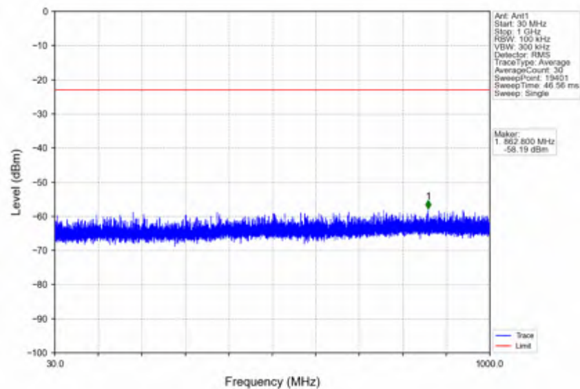
n41_15kHz_SISO_NTNV_30MHz_DFT-s-OFDM QPSK_2511MHz_Edge_1RB_Left
