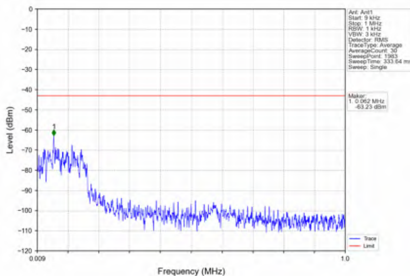
n41_15kHz_SISO_NTNV_40MHz_DFT-s-OFDM_PI/2_BPSK_2516.01MHz_Edge_1RB_Left
