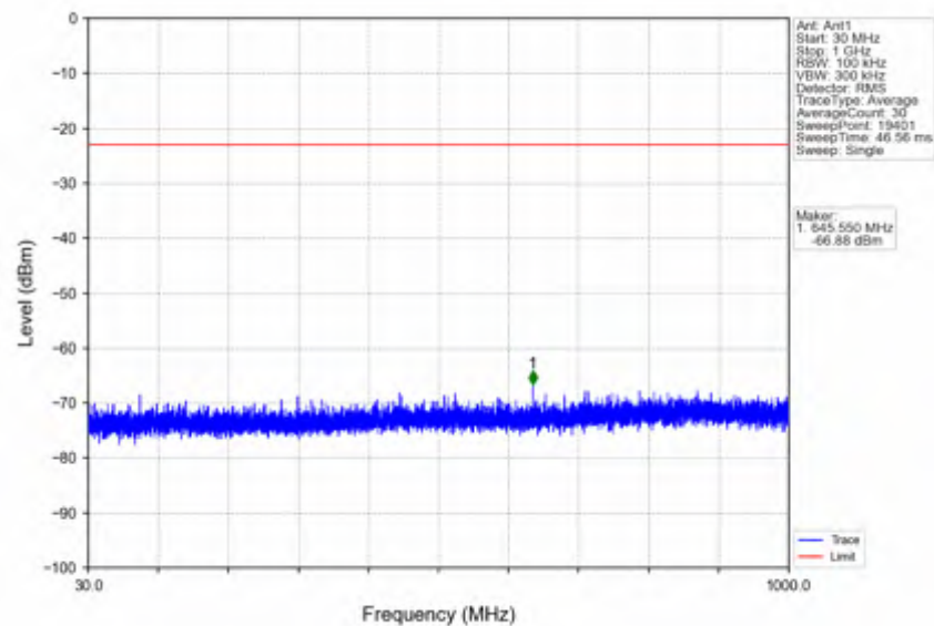
n41_15kHz_SISO_NTV_15MHz_CP-OFDM QPSK_2503.5MHz_Inner_1RB_Left
