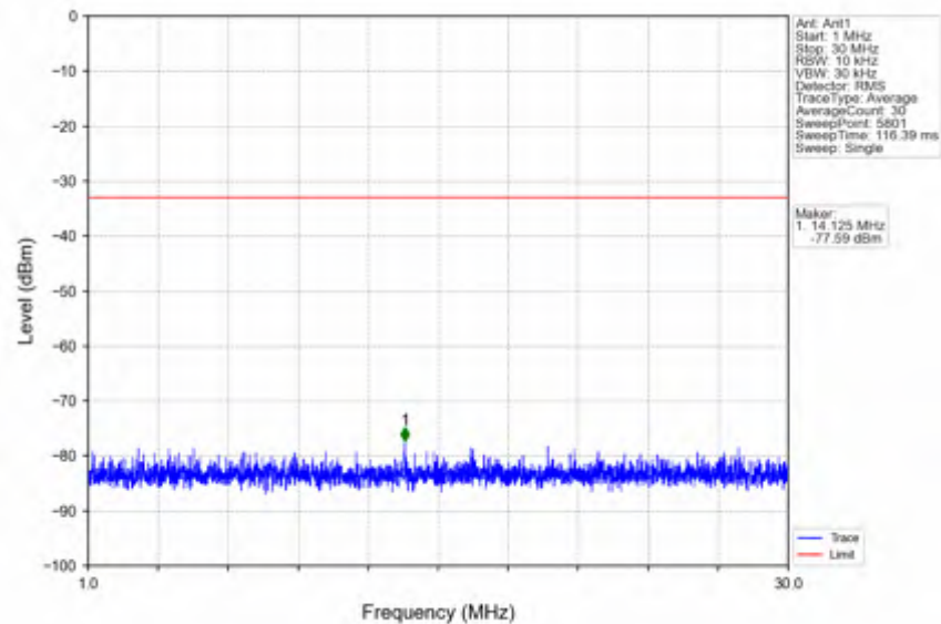
n41_15kHz_SISO_NTNV_30MHz_DFT-s-OFDM_QPSK_2511MHz_Inner_1RB_Left
