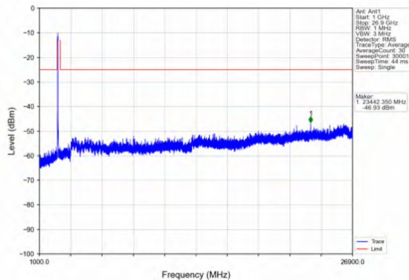
n41_15kHz_SISO_NTNV_30MHz_DFT-s-OFDM QPSK_2511MHz_Inner_1RB_Left
