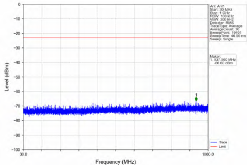
n41_15kHz_SISO_NTNV_20MHz_CP-OFDM QPSK_2506.005MHz_Inner_1RB_Left
