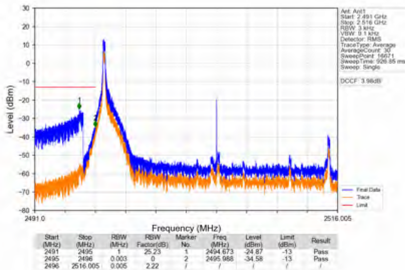
n41_15kHz_SISO_NTNV_20MHz_DFT-s-OFDM QPSK_2506.005MHz_Inner_1RB_Left
