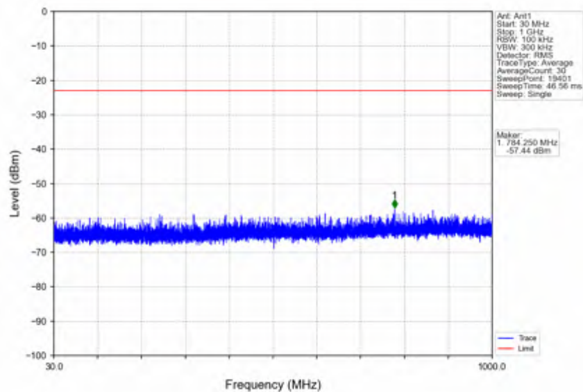
n41_15kHz_SISO_NTNV_20MHz_DFT-s-OFDM_QPSK_2506.005MHz_Edge_1RB_Left
