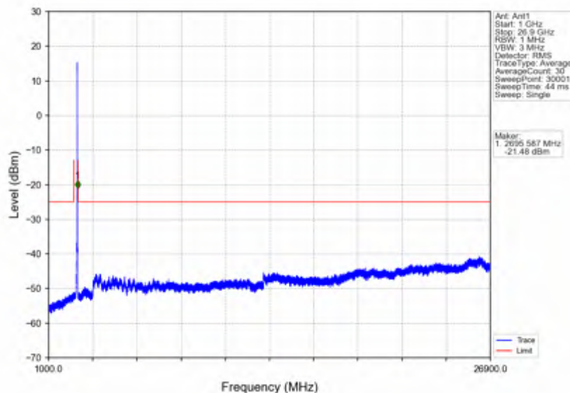
n41_15kHz_SISO_NTNV_20MHz_DFT-s-OFDM QPSK_2679.99MHz_Inner_1RB_Right
