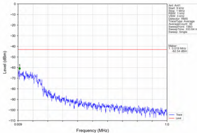
n41_15kHz_SISO_NTNV_20MHz_CP-OFDM QPSK_2506.005MHz_Edge_1RB_Left
