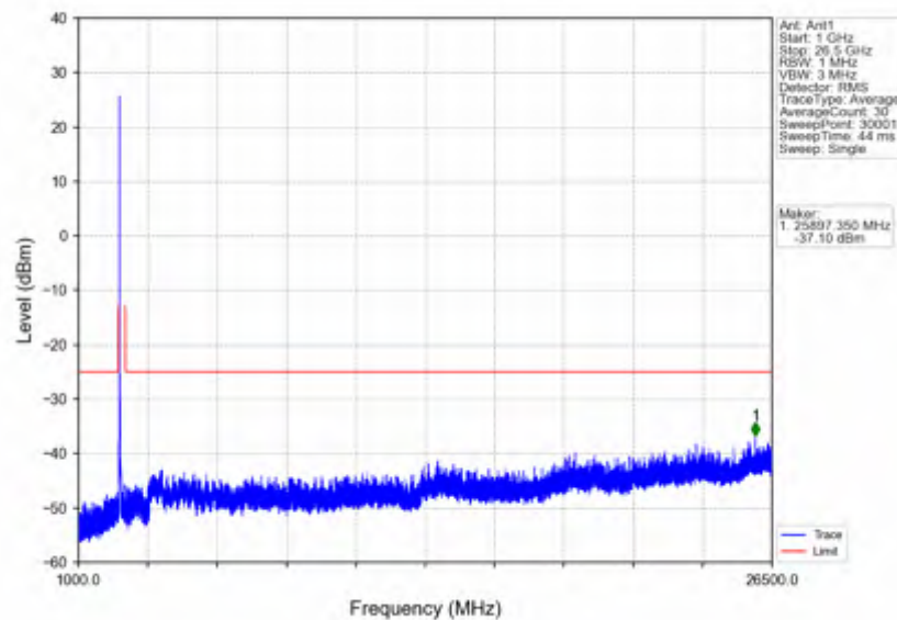
n41_15kHz_SISO_NTNV_30MHz_DFT-s-OFDM QPSK_2511MHz_Edge_1RB_Left
