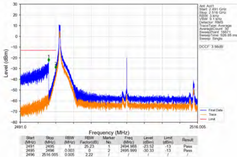
n41_15kHz_SISO_NTNV_20MHz_CP-OFDM QPSK_2506.005MHz_Edge_1RB_Left
