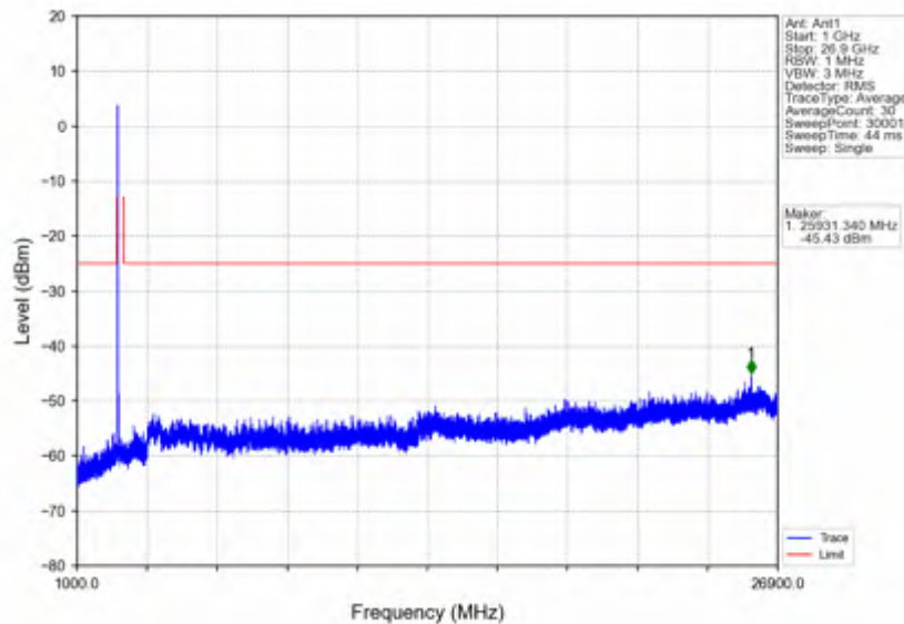
n41_15kHz_SISO_NTNV_30MHz_DFT-s-OFDM_QPSK_2511MHz_Inner_1RB_Left
