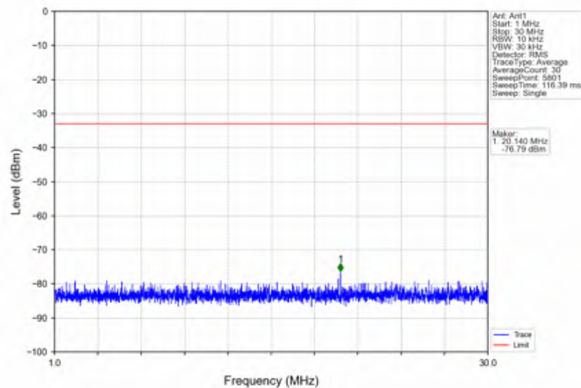
n41_15kHz_SISO_NTNV_30MHz_CP-OFDM_QPSK_2511MHz_Inner_1RB_Left
