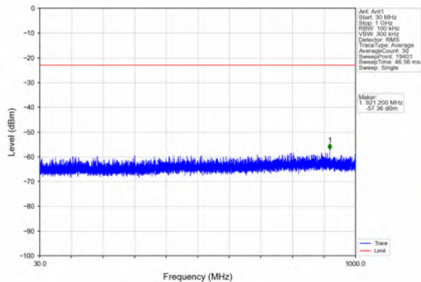
n41_15kHz_SISO_NTNV_30MHz_DFT-s-OFDM PI/2 BPSK_2511MHz_Edge_1RB_Left
