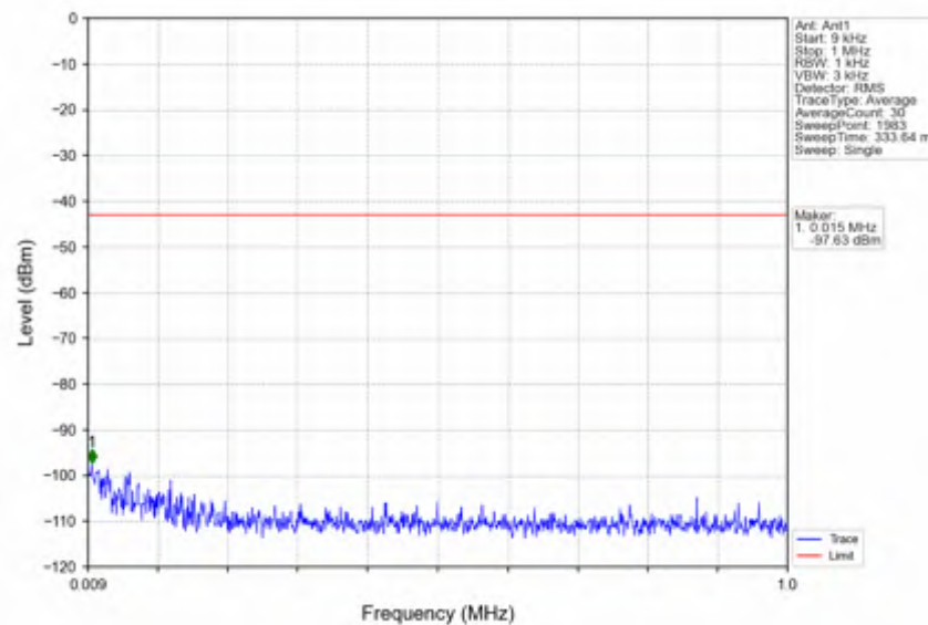
n41_15kHz_SISO_NTNV_10MHz_CP-OFDM QPSK_2685MHz_Inner_1RB_Right
