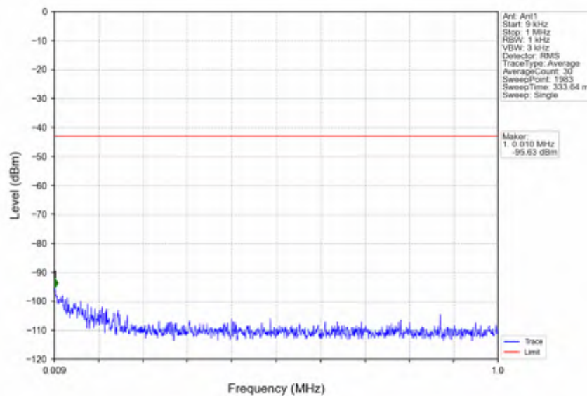
n41_15kHz_SISO_NTNV_30MHz_CP-OFDM_QPSK_2511MHz_Inner_1RB_Left
