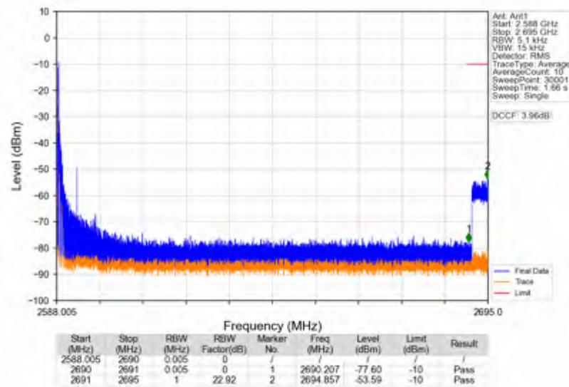
n41 15kHz SISO NTVN 10MHz CP-OFDM QPSK 2593.005MHz Edge 1RB Left
