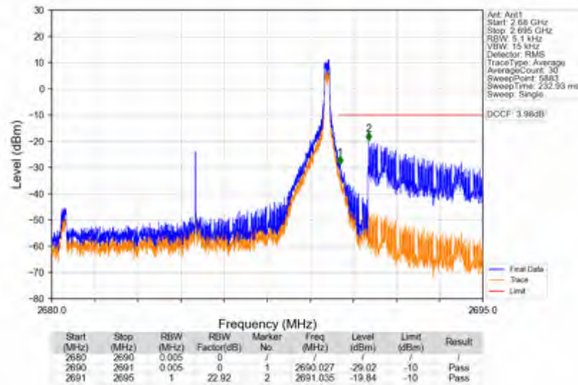
n41_15kHz_SISO_NTNV_10MHz_CP-OFDM_QPSK_2685MHz_Edge_1RB_Right
