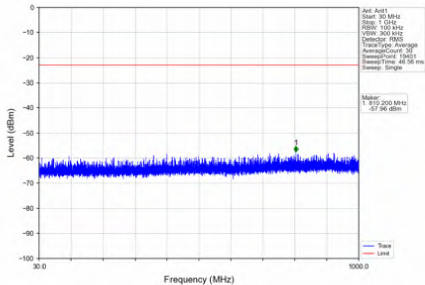
n41_15kHz_SISO_NTNV_10MHz_CP-OFDM QPSK_2593.005MHz_Edge_1RB_Left
