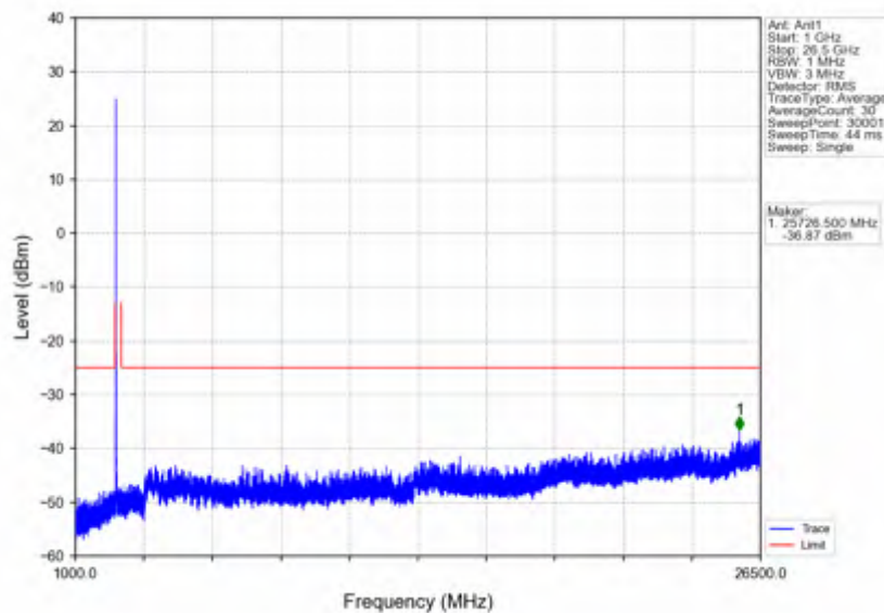
n41_15kHz_SISO_NTNV_20MHz_DFT-s-OFDM_QPSK_2506.005MHz_Edge_1RB_Left
