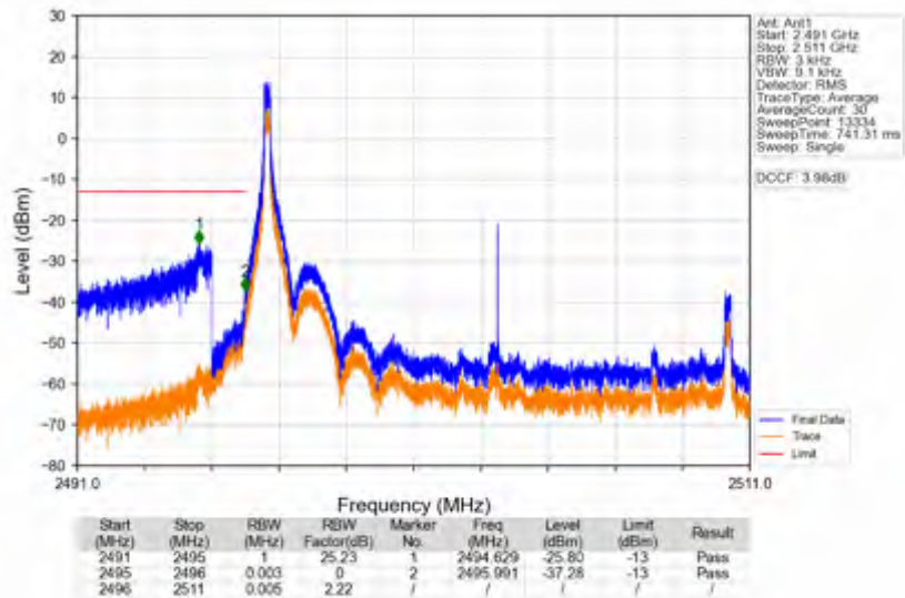
n41_15kHz_SISO_NTNV_15MHz_DFT-s-OFDM_QPSK_2503.5MHz_Inner_1RB_Left
