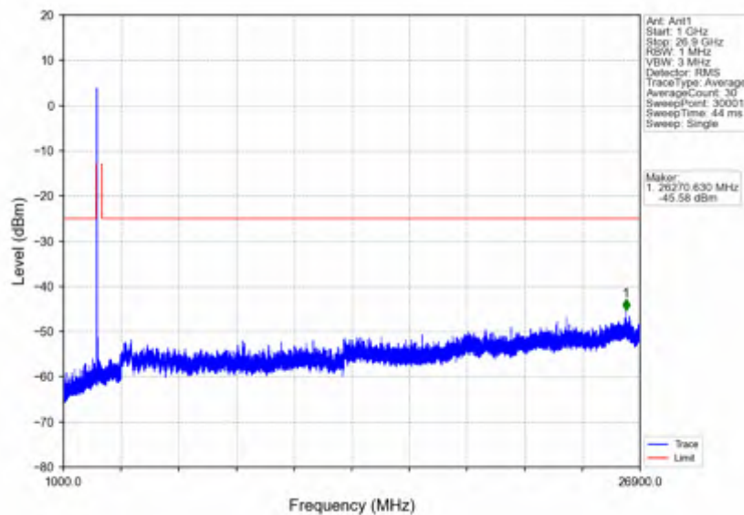
n41_15kHz_SISO_NTNV_30MHz_DFT-s-OFDM PI/2 BPSK_2593.005MHz_Edge_1RB_Left
