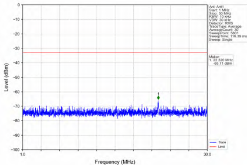
n41_15kHz_SISO_NTNV_20MHz_DFT-s-OFDM QPSK_2593.005MHz_Edge_1RB_Left
