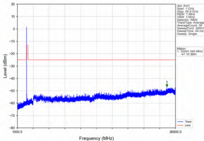
n41_15kHz_SISO_NTNV_30MHz_CP-OFDM QPSK_2593.005MHz_Edge_1RB_Left
