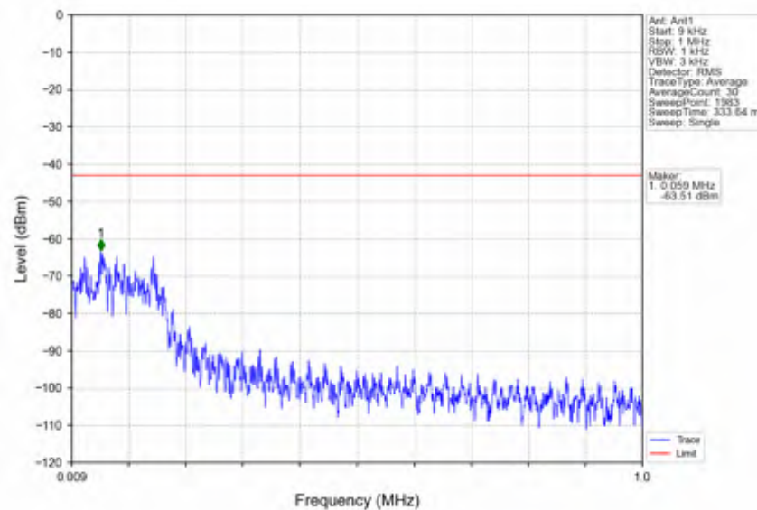
n41_15kHz_SISO_NTNV_20MHz_DFT-s-OFDM QPSK_2593.005MHz_Edge_1RB_Left
