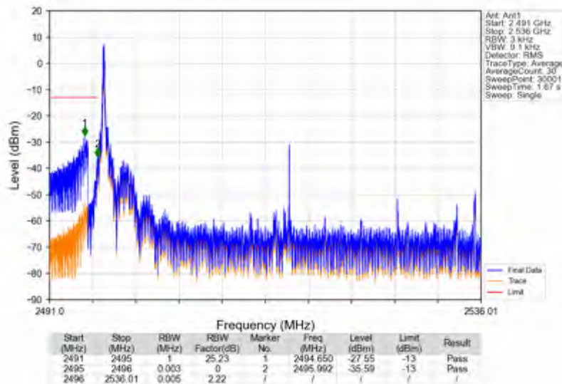
n41_15kHz_SISO_NTNV_40MHz_DFT-s-OFDM_PI/2_BPSK_2516.01MHz_Edge_1RB_Left
