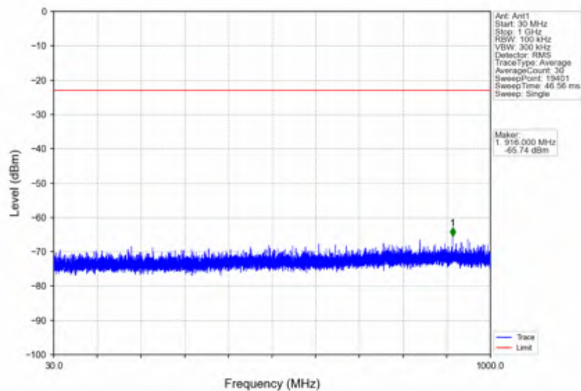
n41_15kHz_SISO_NTNV_20MHz_DFT-s-OFDM QPSK_2506.005MHz_Inner_1RB_Left
