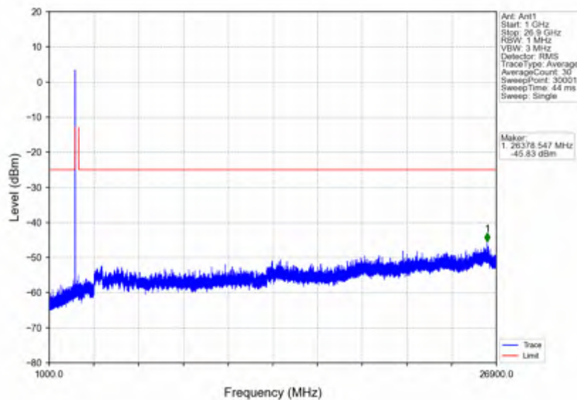
n41 15kHz SISO NTVN 10MHz CP-OFDM QPSK 2593.005MHz Edge 1RB Left
