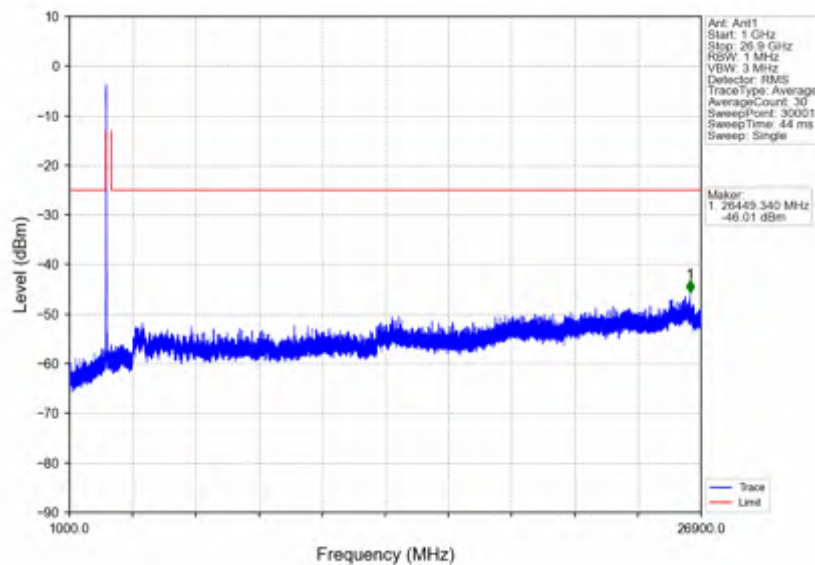
n41_15kHz_SISO_NTNV_15MHz_DFT-s-OFDM_QPSK_2503.5MHz_Inner_1RB_Left
