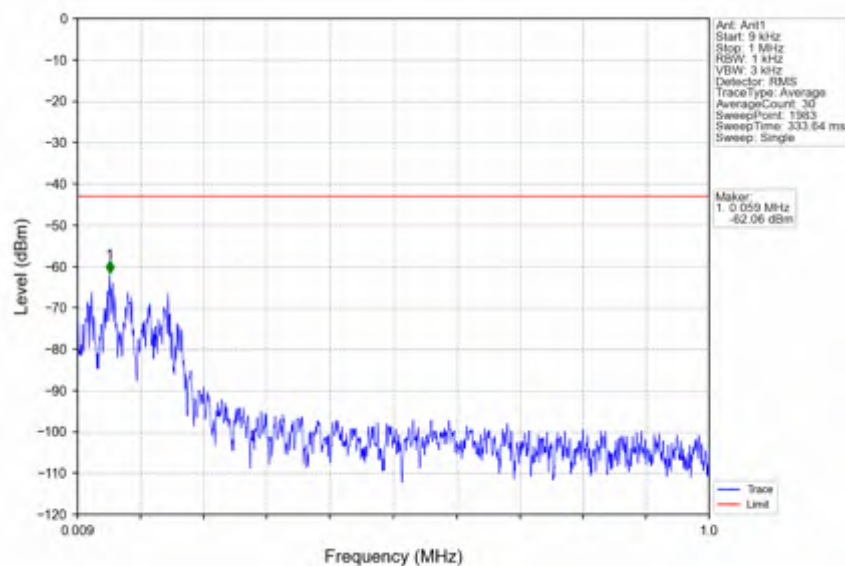
n41_15kHz_SISO_NTNV_20MHz_DFT-s-OFDM_PI/2_BPSK_2506.005MHz_Edge_1RB_Left
