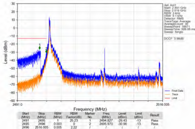
n41_15kHz_SISO_NTNV_20MHz_DFT-s-OFDM_PI/2_BPSK_2506.005MHz_Edge_1RB_Left
