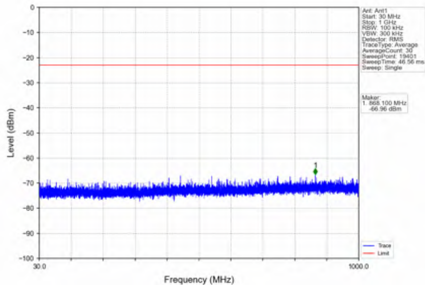
n41_15kHz_SISO_NTNV_30MHz_DFT-s-OFDM_QPSK_2511MHz_Inner_1RB_Left
