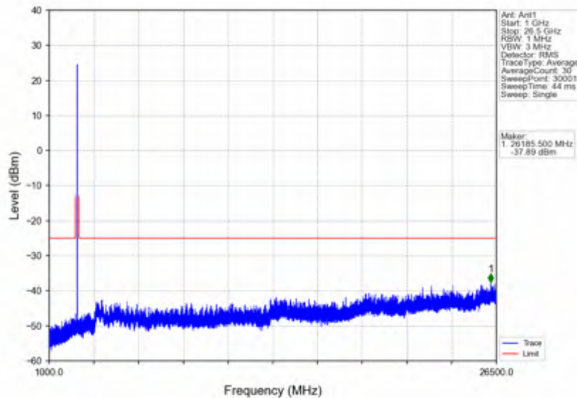
n41_15kHz_SISO_NTNV_10MHz_CP-OFDM QPSK_2593.005MHz_Edge_1RB_Left
