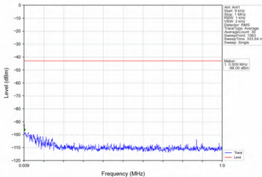
n41_15kHz_SISO_NTV_15MHz_CP-OFDM QPSK_2503.5MHz_Inner_1RB_Left
