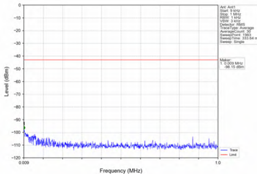
n41_15kHz_SISO_NTNV_15MHz_DFT-s-OFDM PI/2 BPSK_2503.5MHz_Inner_1RB_Left
