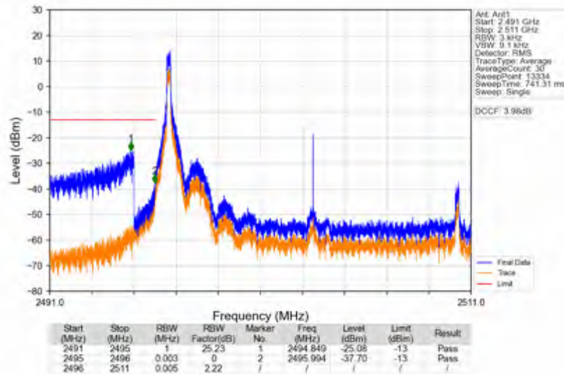
n41_15kHz_SISO_NTV_15MHz_CP-OFDM QPSK_2503.5MHz_Inner_1RB_Left
