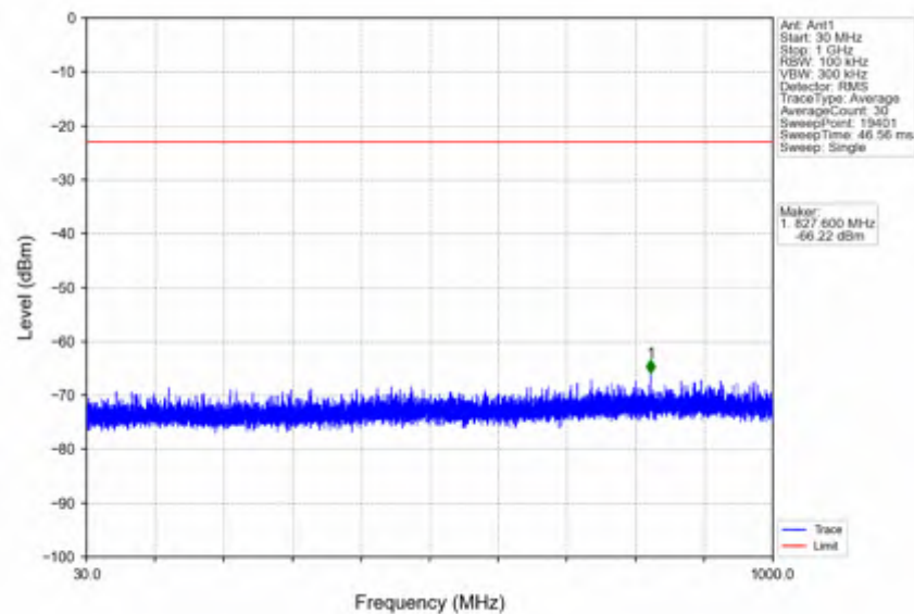
n41_15kHz_SISO_NTNV_20MHz_CP-OFDM QPSK_2679.99MHz_Inner_1RB_Right
