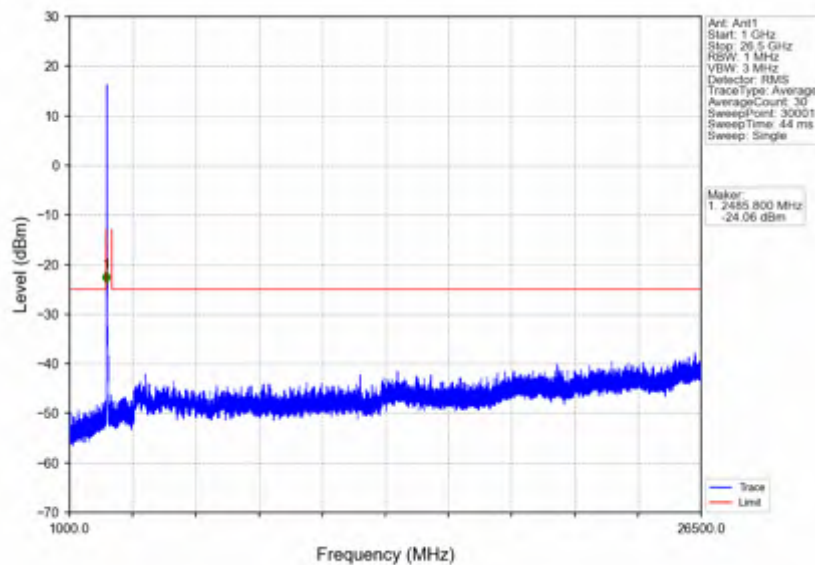
n41_15kHz_SISO_NTNV_20MHz_DFT-s-OFDM QPSK_2506.005MHz_Inner_1RB_Left
