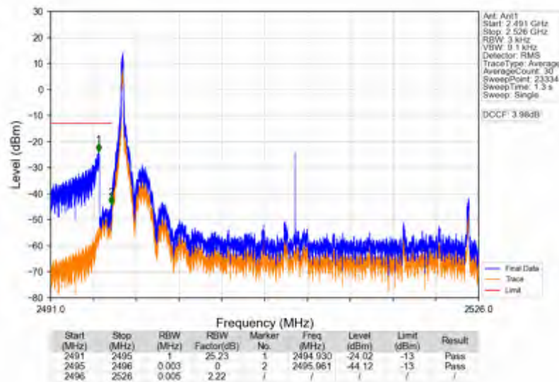
n41_15kHz_SISO_NTNV_30MHz_DFT-s-OFDM QPSK_2511MHz_Inner_1RB_Left
