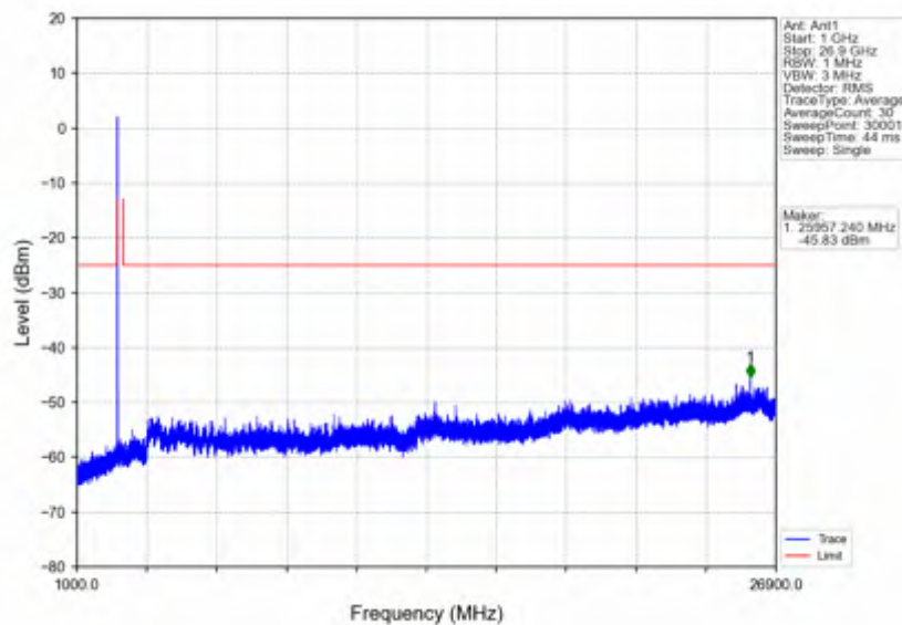
n41_15kHz_SISO_NTNV_15MHz_CP-OFDM_QPSK_2593.005MHz_Edge_1RB_Left
