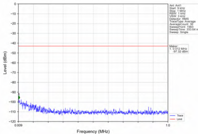
n41_15kHz_SISO_NTNV_10MHz_CP-OFDM_QPSK_2501.01MHz_Inner_1RB_Left
