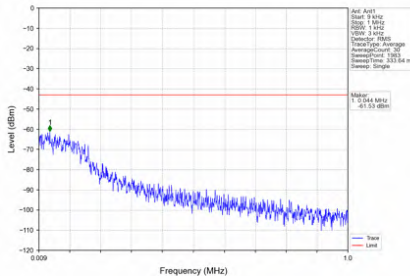
n41_15kHz_SISO_NTNV_10MHz_CP-OFDM_QPSK_2685MHz_Edge_1RB_Right
