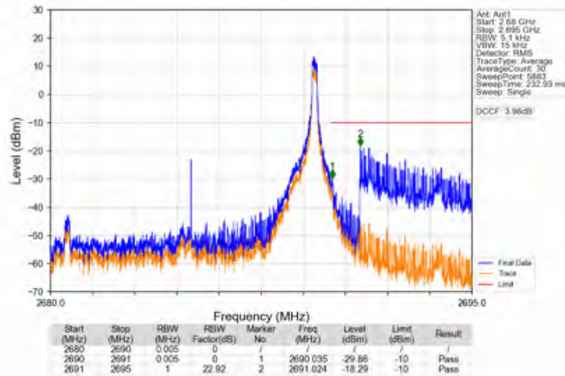
n41_15kHz_SISO_NTNV_10MHz_CP-OFDM QPSK_2685MHz_Inner_1RB_Right
