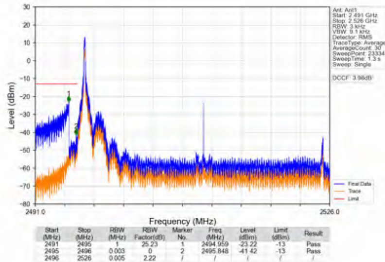
n41_15kHz_SISO_NTNV_30MHz_CP-OFDM_QPSK_2511MHz_Inner_1RB_Left
