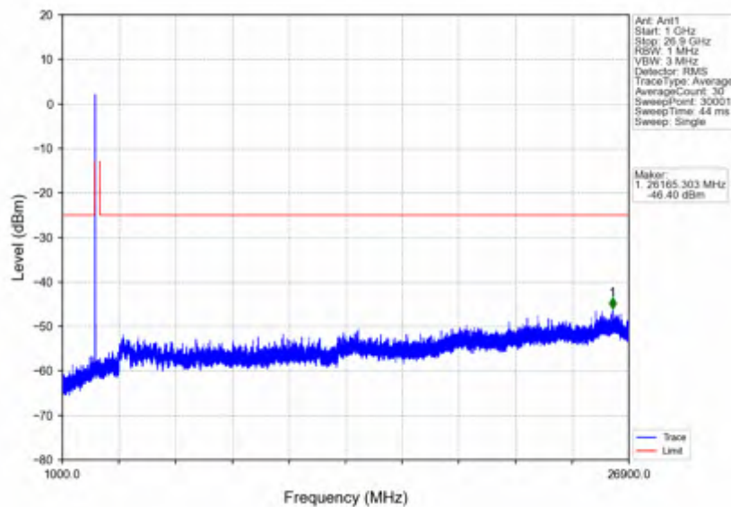
n41_15kHz_SISO_NTNV_20MHz_CP-OFDM QPSK_2593.005MHz_Edge_1RB_Left
