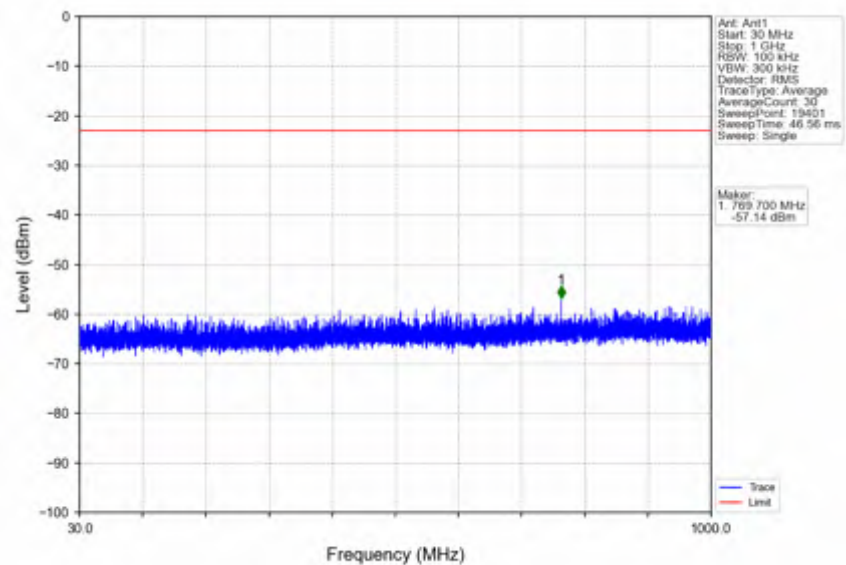
n41_15kHz_SISO_NTNV_10MHz_CP-OFDM QPSK_2685MHz_Edge_1RB_Right
