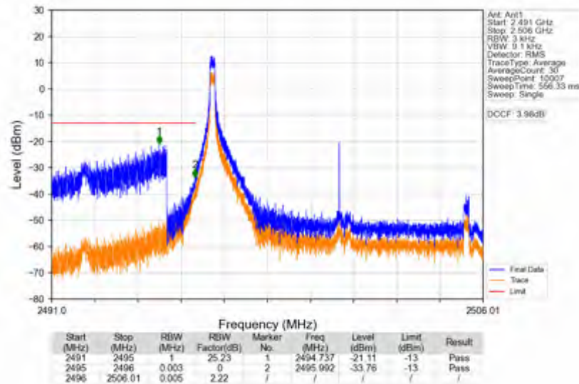
n41_15kHz_SISO_NTNV_10MHz_CP-OFDM_QPSK_2501.01MHz_Inner_1RB_Left
