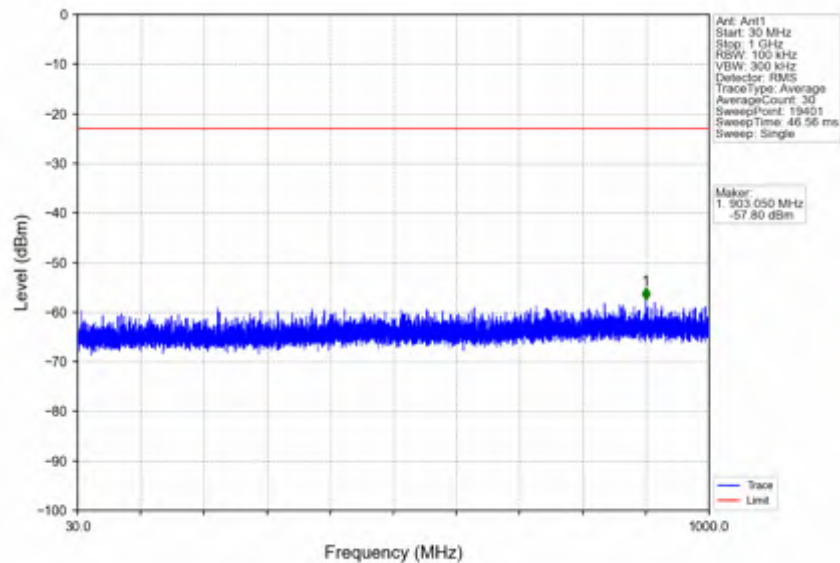
n41_15kHz_SISO_NTNV_20MHz_CP-OFDM_QPSK_2593.005MHz_Edge_1RB_Left
