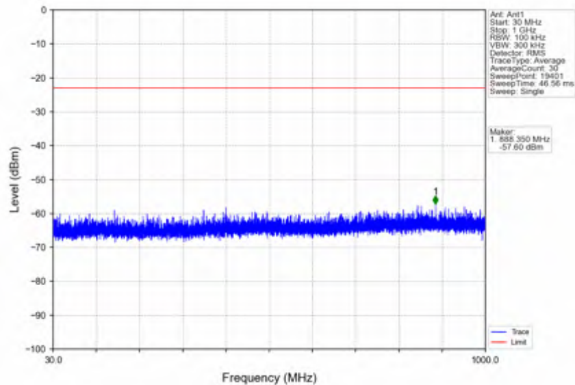
n41_15kHz_SISO_NTNV_15MHz_CP-OFDM_QPSK_2593.005MHz_Edge_1RB_Left
