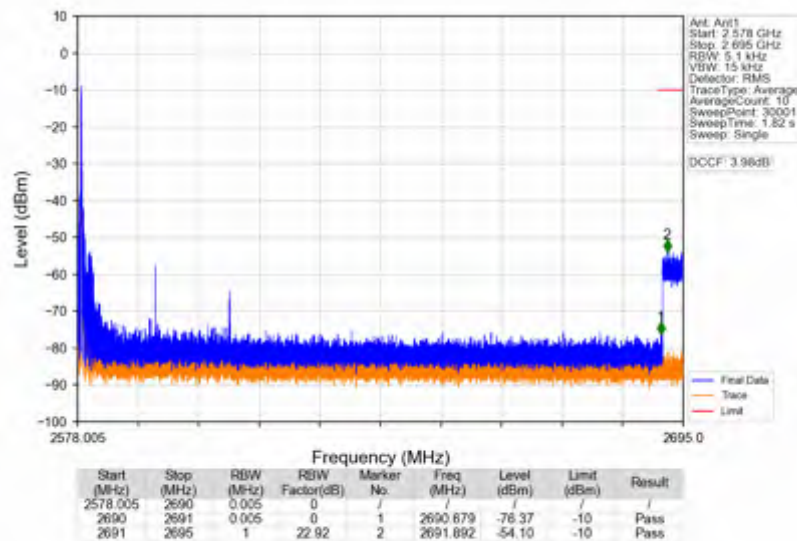
n41_15kHz_SISO_NTNV_30MHz_DFT-s-OFDM PI/2 BPSK_2593.005MHz_Edge_1RB_Left
