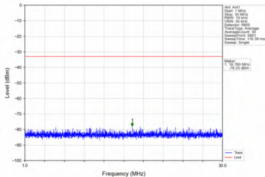
n41_15kHz_SISO_NTV_15MHz_CP-OFDM QPSK_2503.5MHz_Inner_1RB_Left
