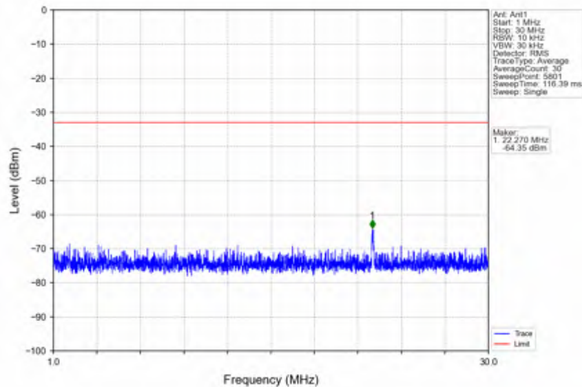
n41_15kHz_SISO_NTNV_20MHz_CP-OFDM QPSK_2593.005MHz_Edge_1RB_Left
