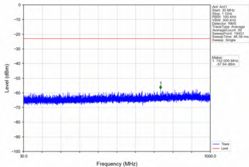
n41_15kHz_SISO_NTNV_10MHz_CP-OFDM QPSK_2501.01MHz_Edge_1RB_Left
