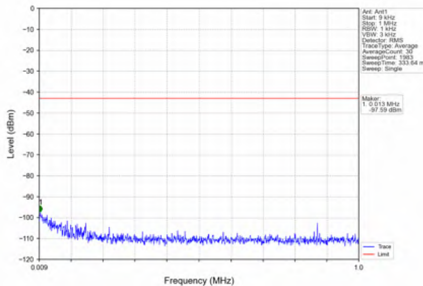
n41_15kHz_SISO_NTNV_20MHz_CP-OFDM QPSK_2679.99MHz_Inner_1RB_Right
