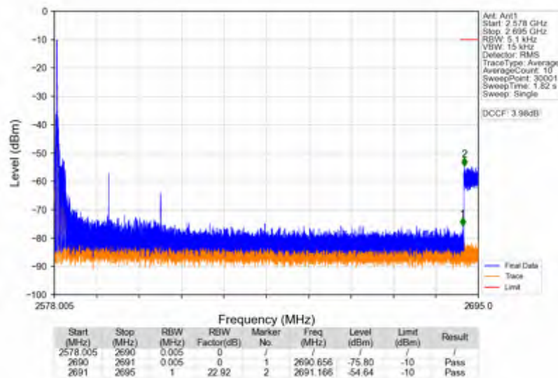
n41_15kHz_SISO_NTNV_30MHz_CP-OFDM QPSK_2593.005MHz_Edge_1RB_Left
