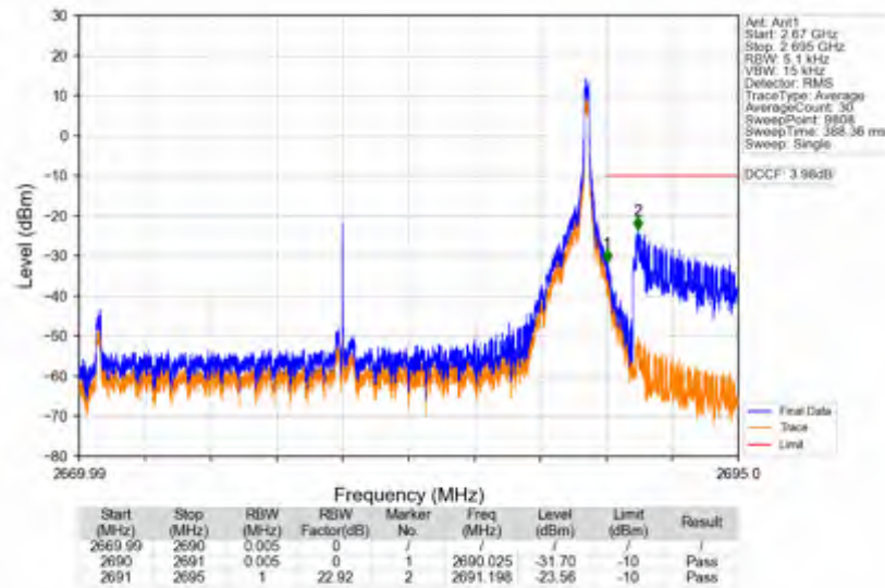
n41_15kHz_SISO_NTNV_20MHz_CP-OFDM QPSK_2679.99MHz_Inner_1RB_Right
