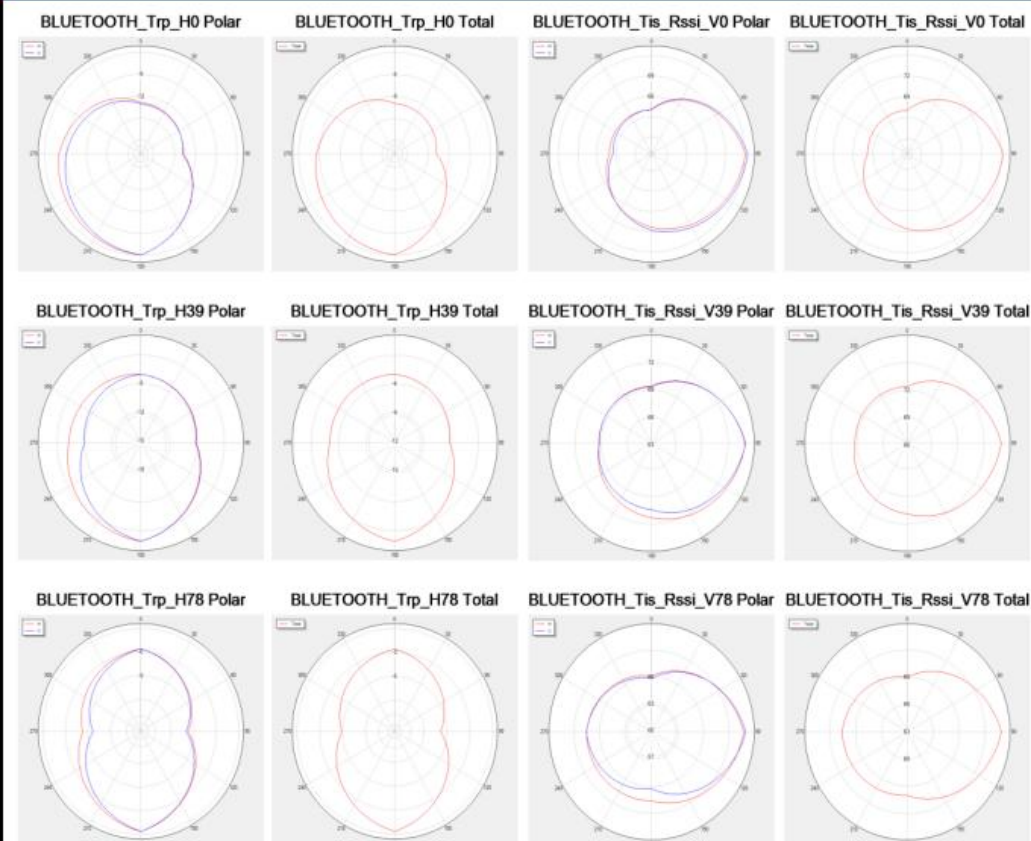
F5-有源方向图-（R自由空间）
