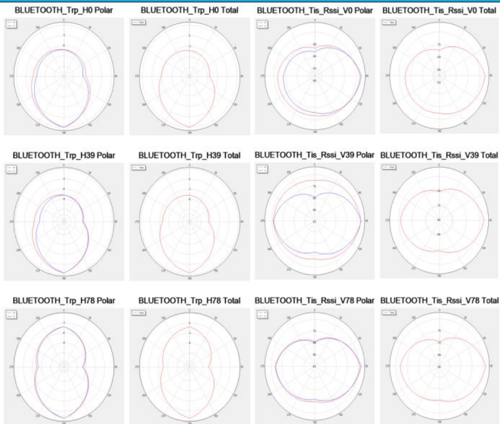
F5-有源方向图-（L自由空间）
