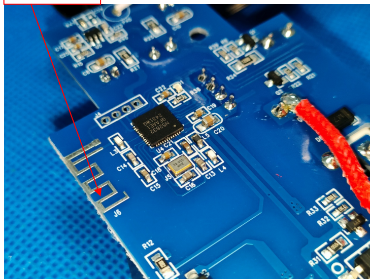
Antenna
