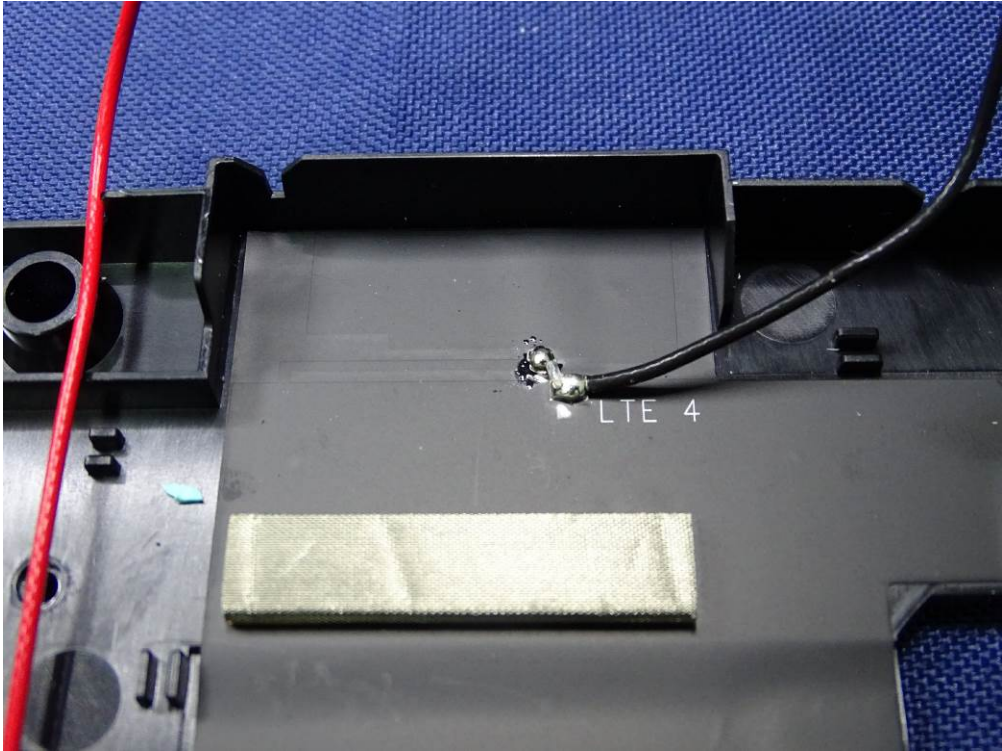
(65) EUT Photo (LTE 1 (ANT_1))
