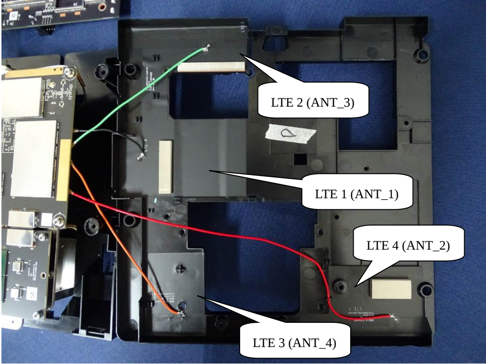
(62) EUT Photo
