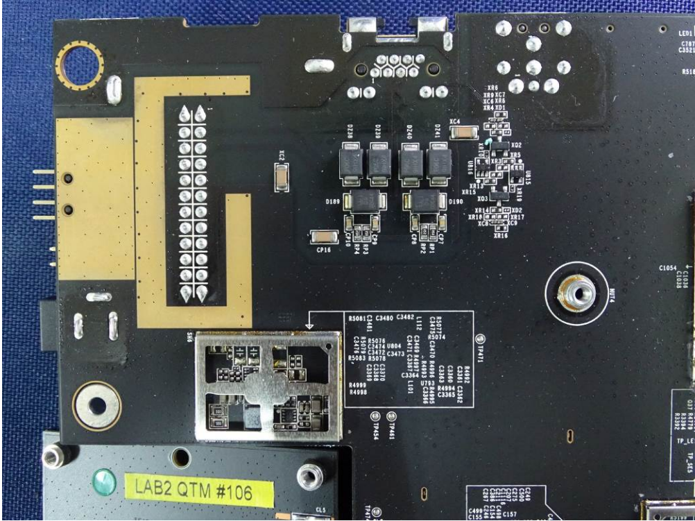
(74) EUT Photo
