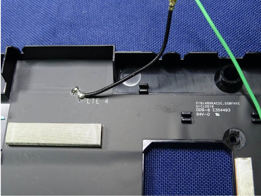
(66) EUT Photo (
