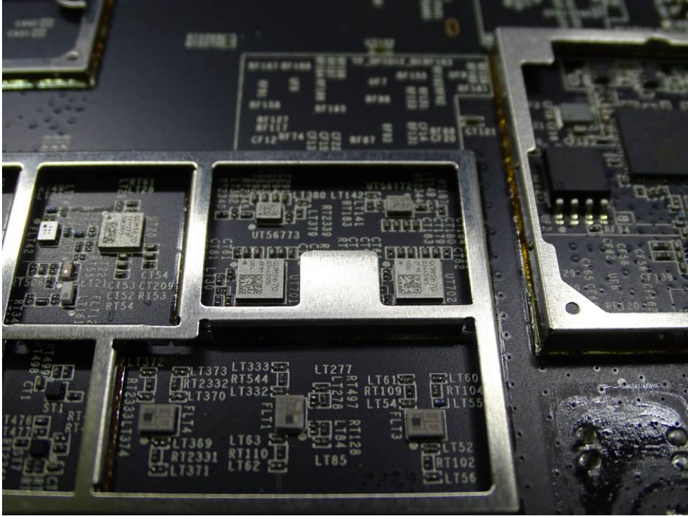
(86) EUT Photo
