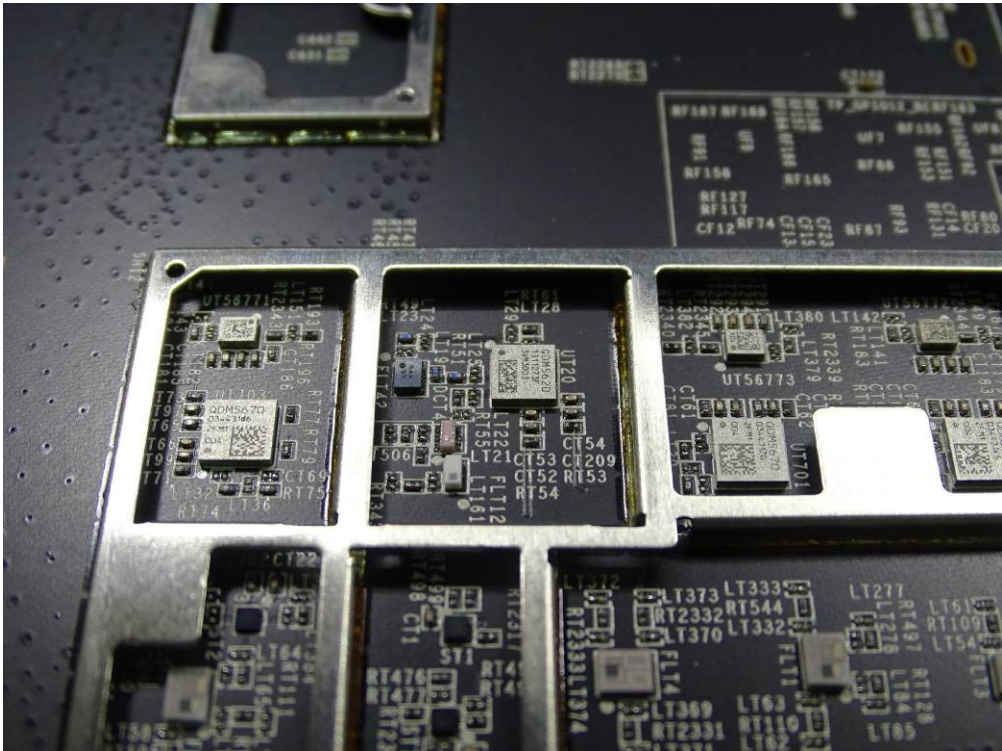
(87) EUT Photo
