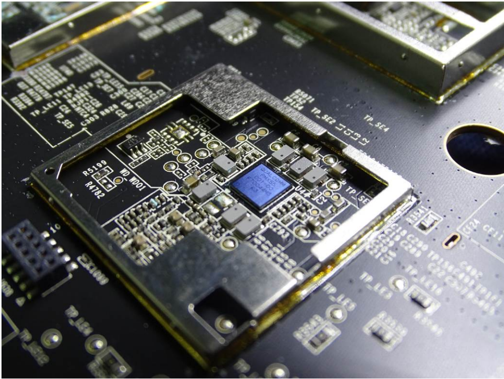
(82) EUT Photo
