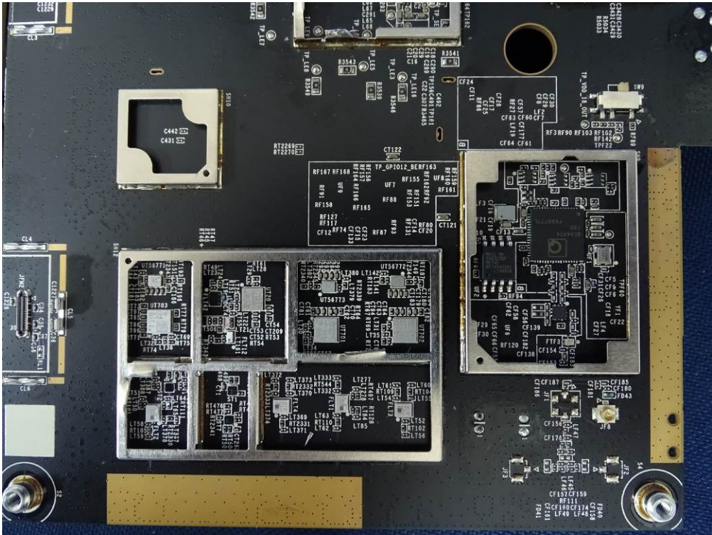
(81) EUT Photo
