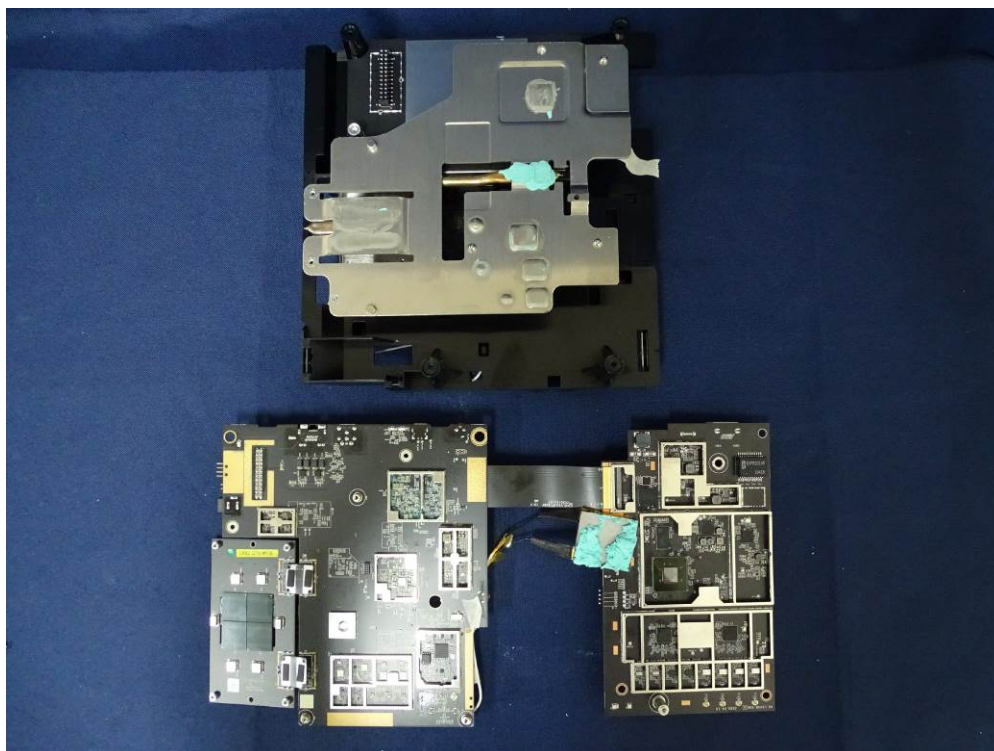
(69) EUT Photo
