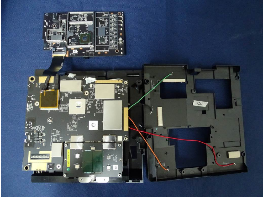
(61) EUT Photo
