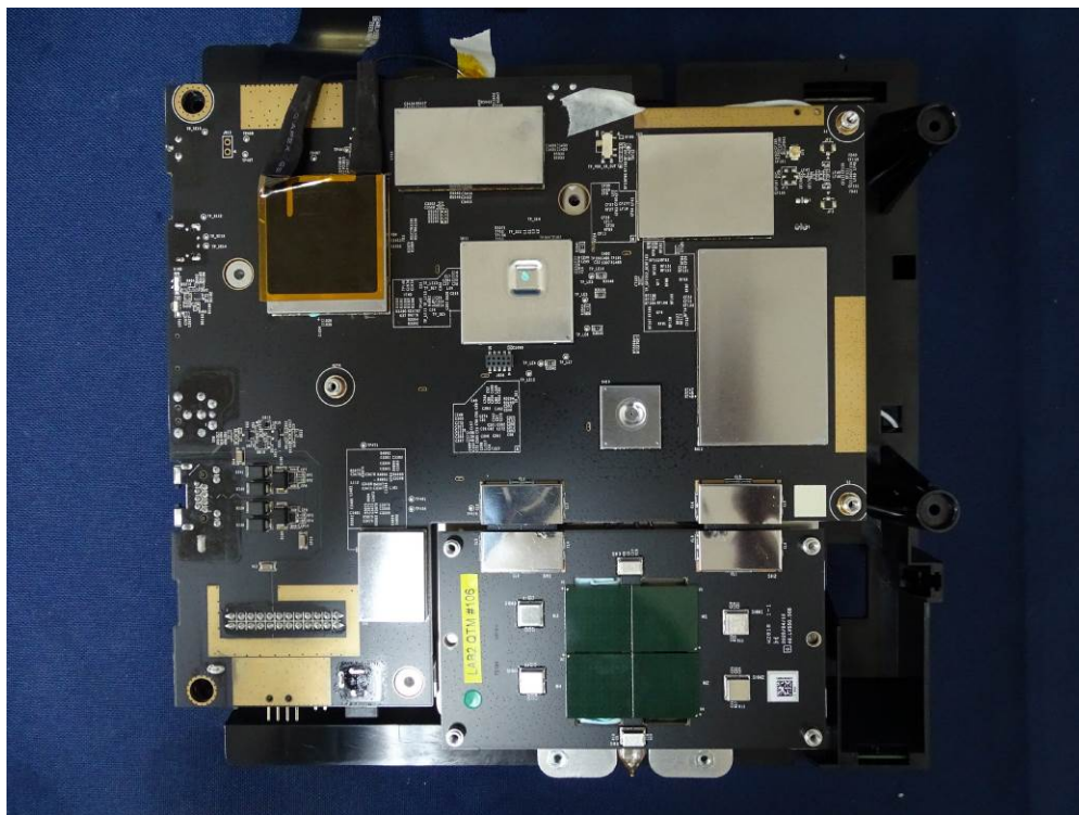
(70) EUT Photo
