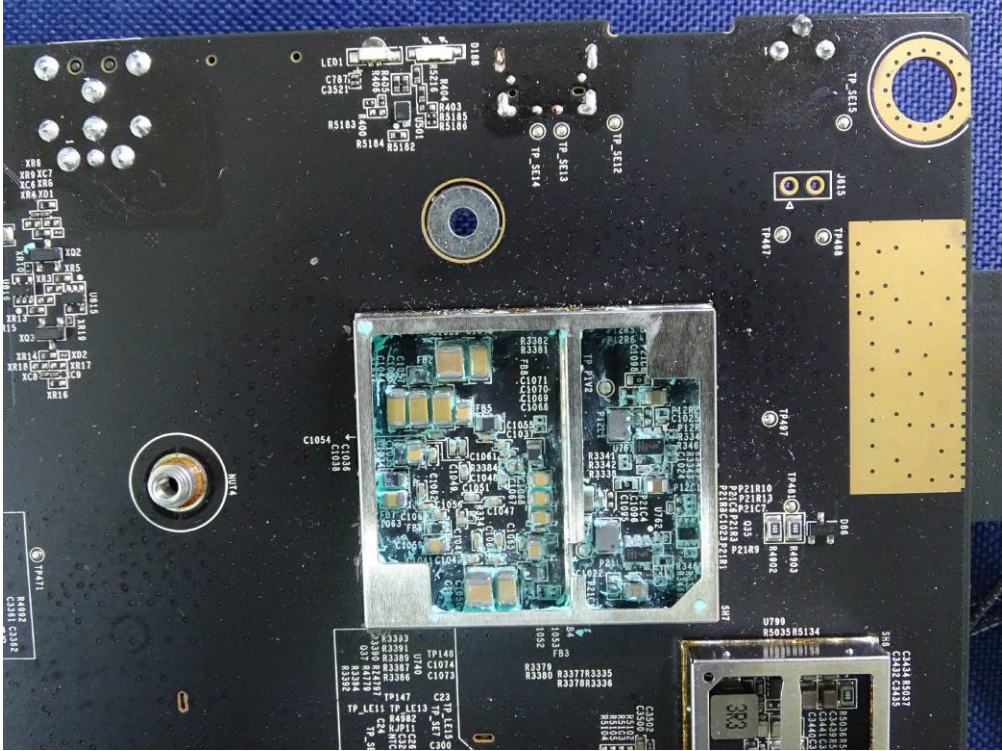
(72) EUT Photo
