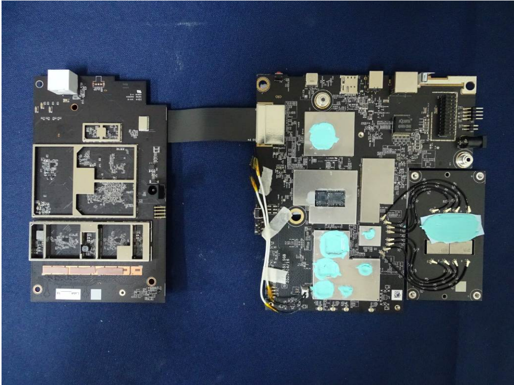
(91) EUT Photo
