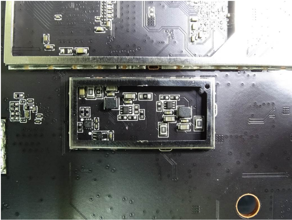
(56) EUT Photo
