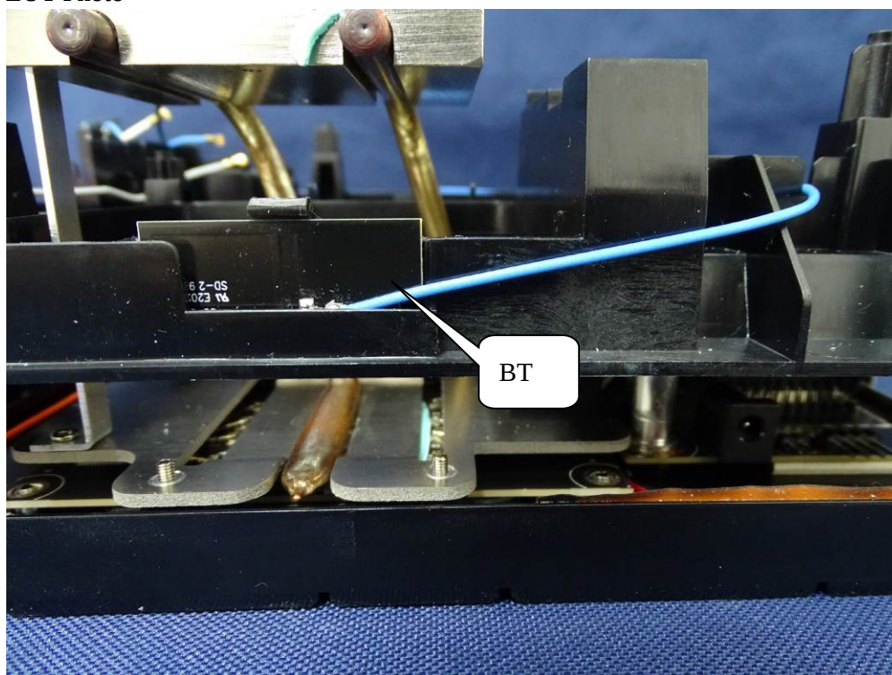
(57) EUT Photo
