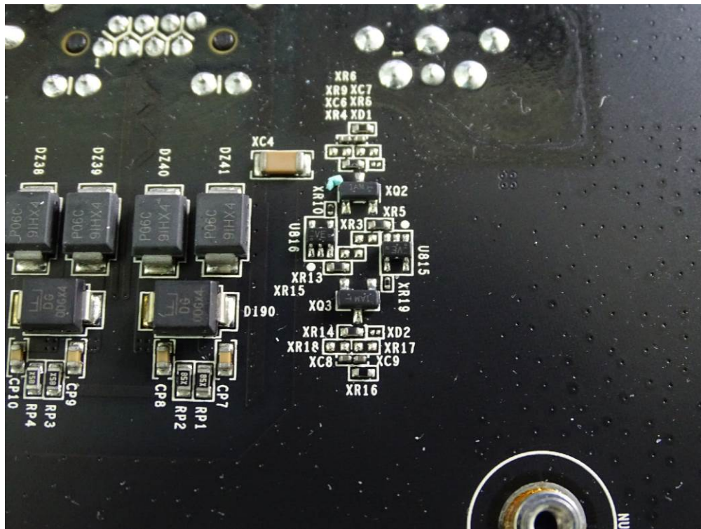
(77) EUT Photo
