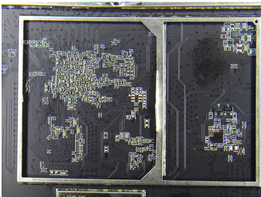
(54) EUT Photo
