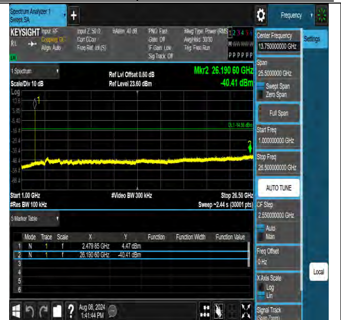
BLE 1M-Ant2-2480-1000~26500-PASS
