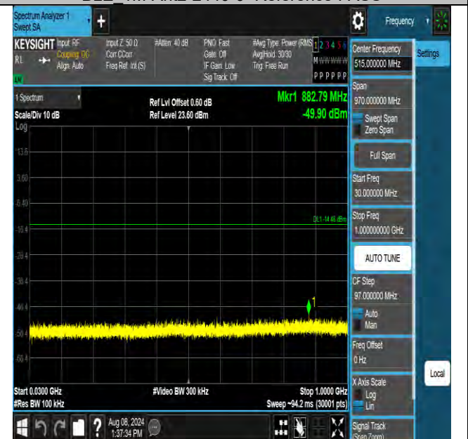
BLE 1M-Ant2-2440-30~1000-PASS
