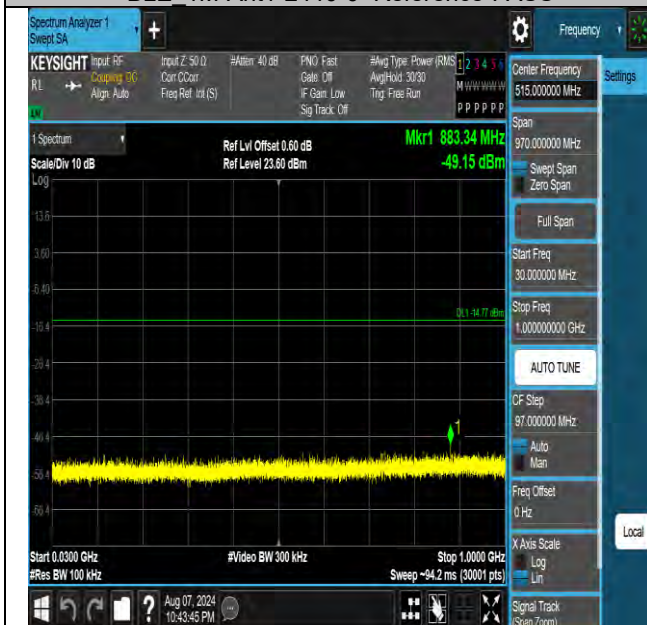
BLE 1M-Ant1-2440-30~1000-PASS
