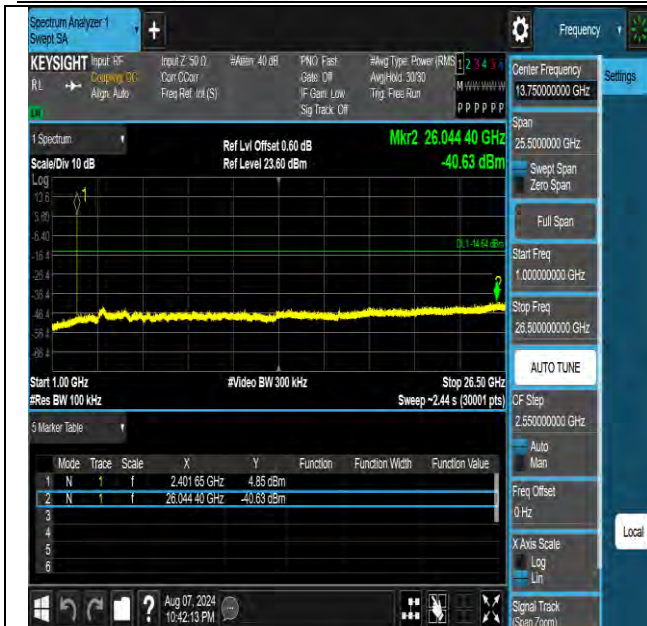
BLE 1M-Ant1-2402-1000~26500-PASS
