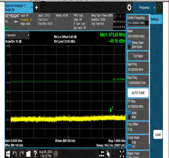
BLE 1M-Ant2-2480-30~1000-PASS
