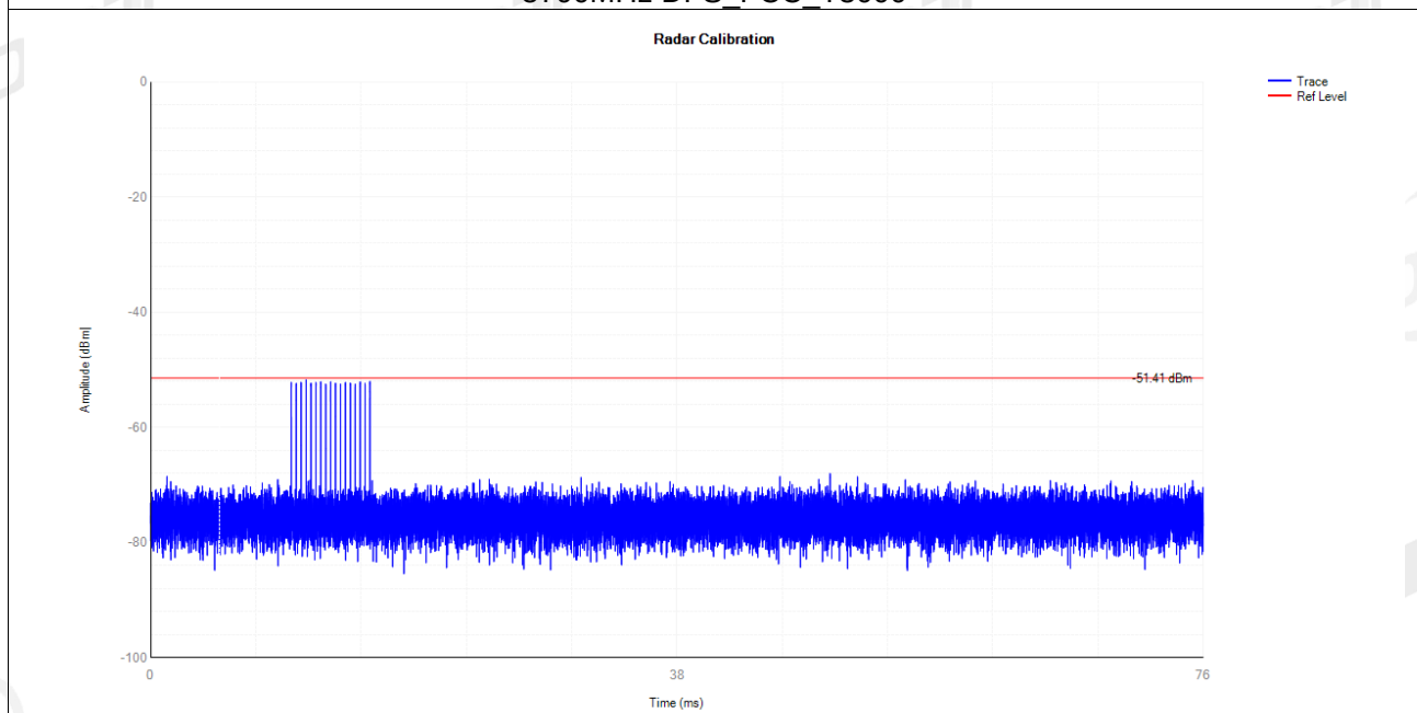
5700MHz DFS_FCC_T4000
