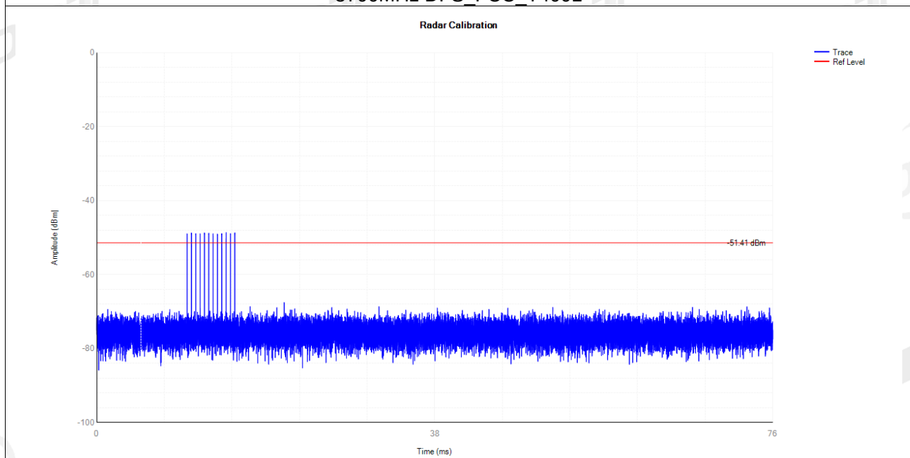
5700MHz DFS_FCC_T5000
