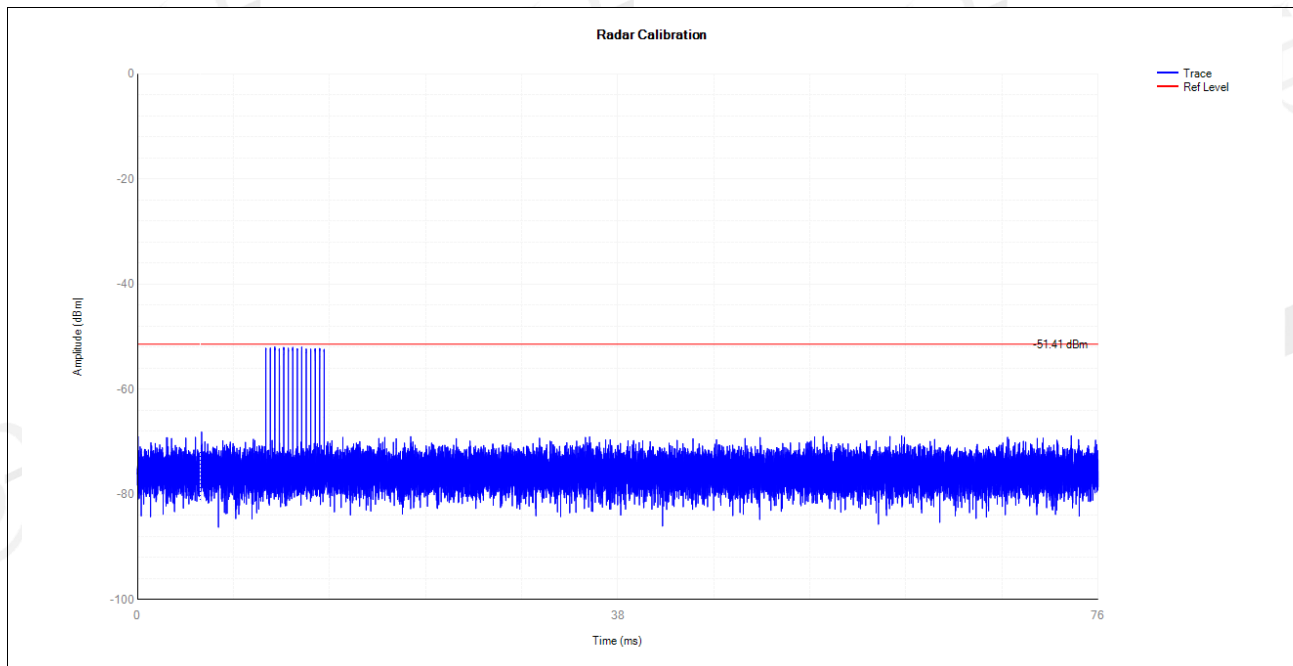
5700MHz DFS_FCC_T4001
