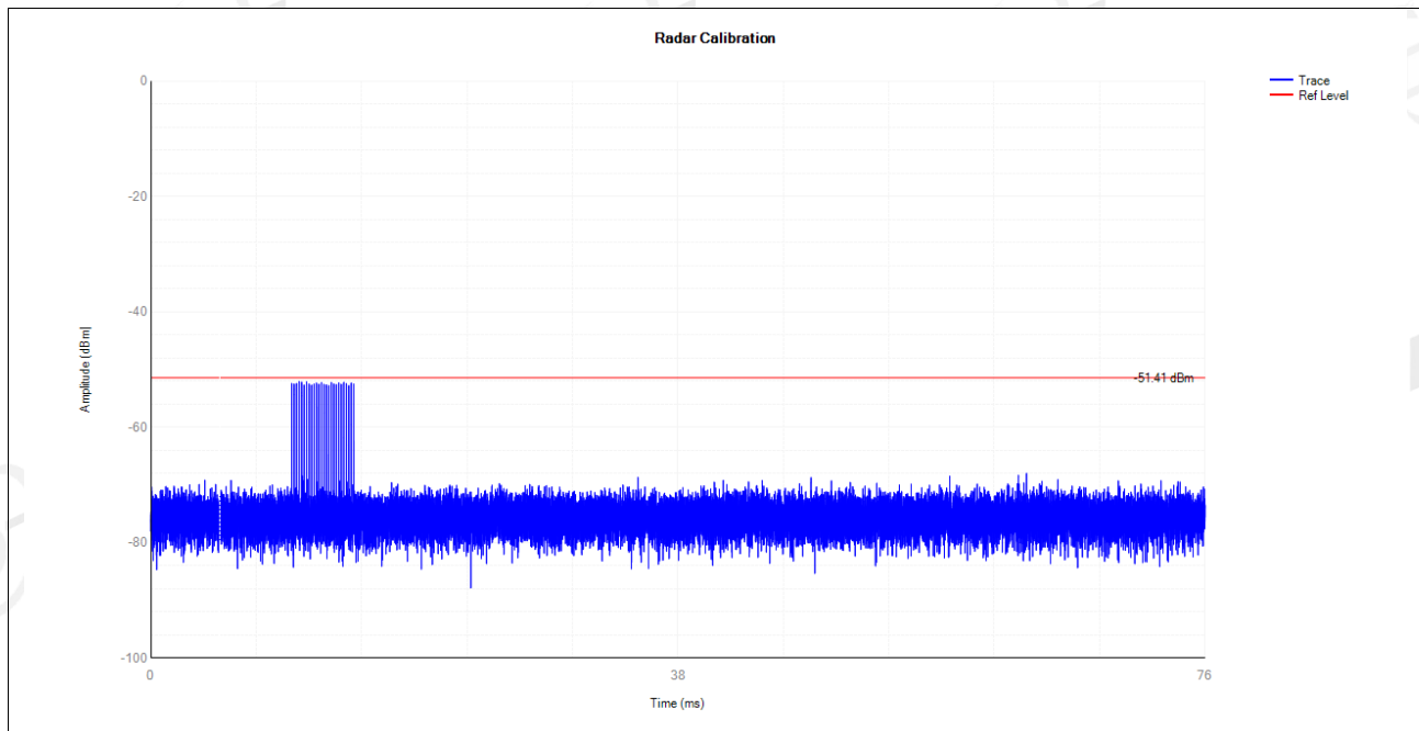
5700MHz DFS_FCC_T3000
