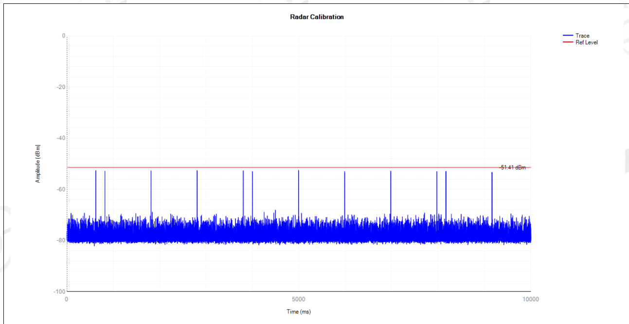
5700MHz DFS_FCC_T6000
