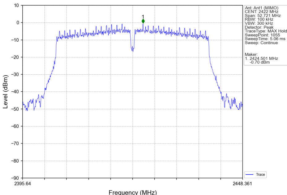
802.11n(HT40)_LCH_2422MHz_Ant1 (MIMO)_NTNV
