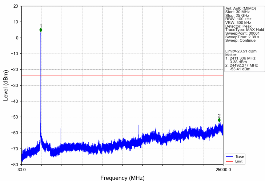
802.11b_LCH_2412MHz_Ant0 (MIMO)_NTNV
