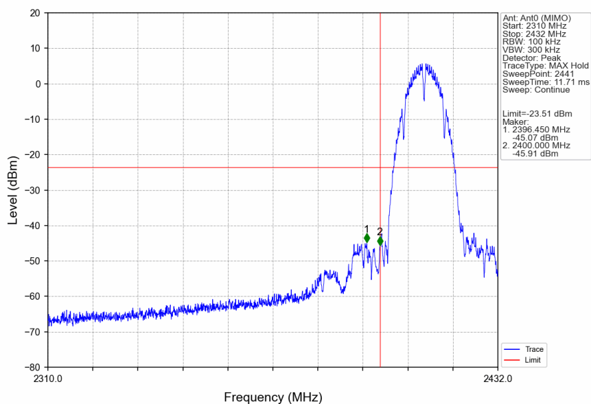
802.11b_LCH_2412MHz_Ant0 (MIMO)_NTNV
