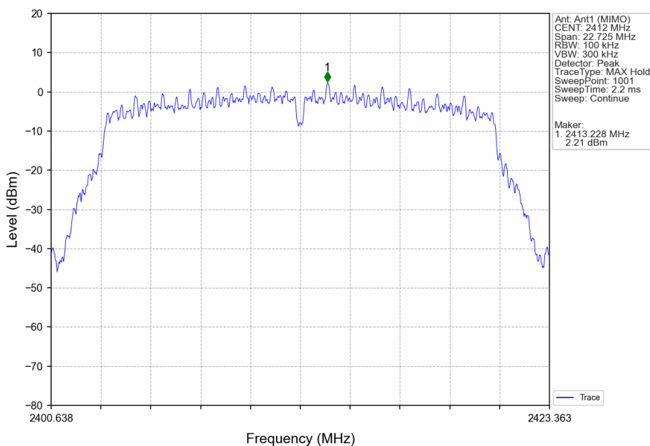
802.11n(HT20)_LCH_2412MHz_Ant1 (MIMO)_NTNV
