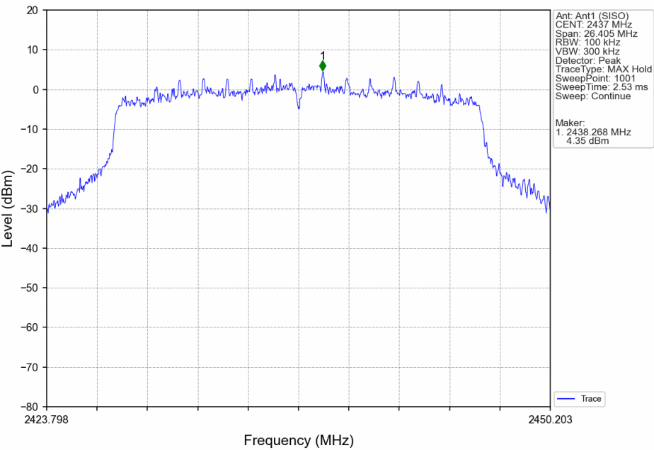
802.11ax(HE20)_MCH_2437MHz_SU_/_Ant1 (SISO)_NTNV
