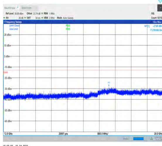
1-N25--15-40-L-1-DFT-PI2BPSK-Inner_1RB_Left-1@ 1-12000-20000-Ant0--27.80--13-PASS
