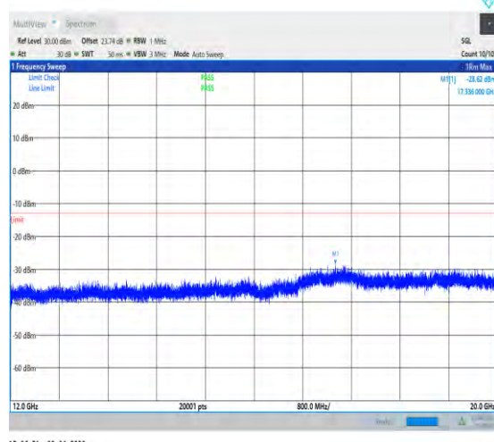
1-N25--15-40-M-1-DFT-PI2BPSK-Inner_1RB_Left-1 @1-12000-20000-Ant0--28.62--13-PASS
