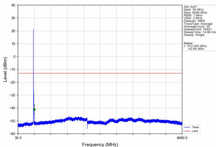
Band5 10MHz QPSK LCH 829MHz RB 50 0 NTN
