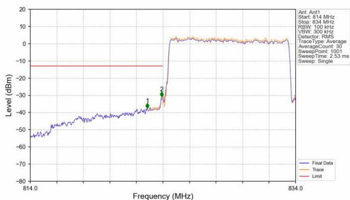
Band5 10MHz QPSK LCH 829MHz RB 50 0 NTN
