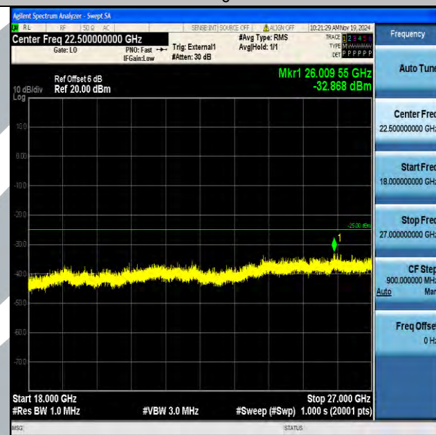
Band38_20MHz_16QAM_38000_1RB#0_18000~27000_18000~27000
