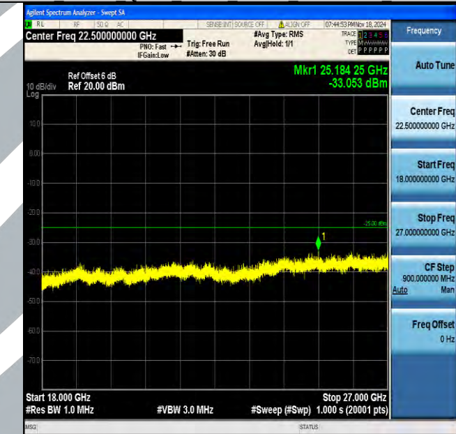
Band7_20MHz_QPSK_21350_1RB#0_18000~27000_18000~27000
