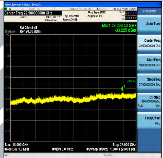
Band38_10MHz_16QAM_38200_1RB#0_18000~27000_18000~27000
