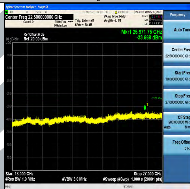
Band38_15MHz_16QAM_38000_1RB#0_18000~27000_18000~27000
