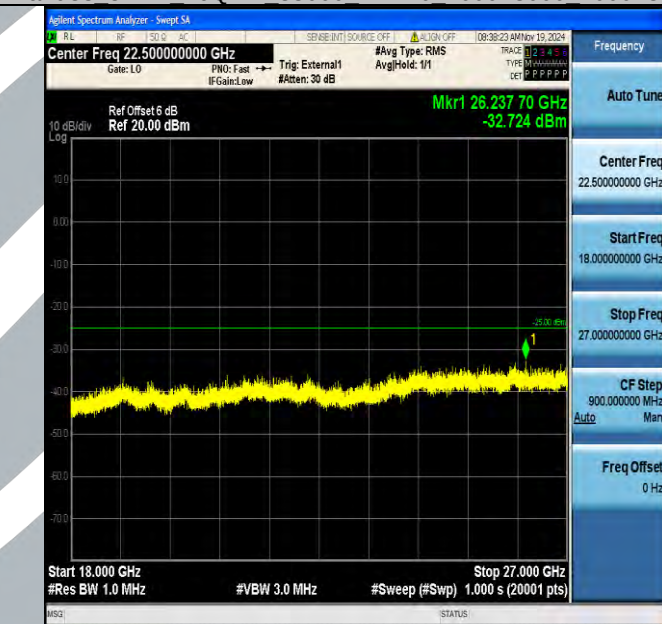
Band38_5MHz_16QAM_38000_1RB#0_18000~27000_18000~27000
