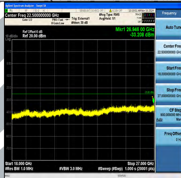
Band38_20MHz_QPSK_38000_1RB#0_18000~27000_18000~27000
