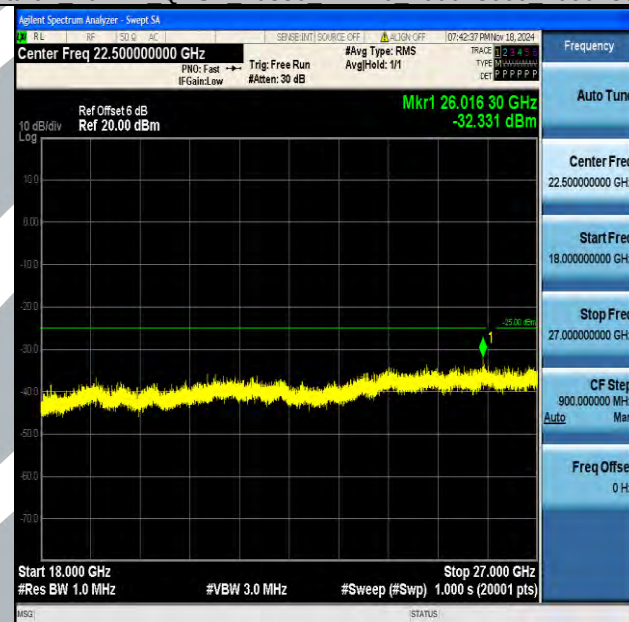
Band7_20MHz_QPSK_20850_1RB#0_18000~27000_18000~27000
