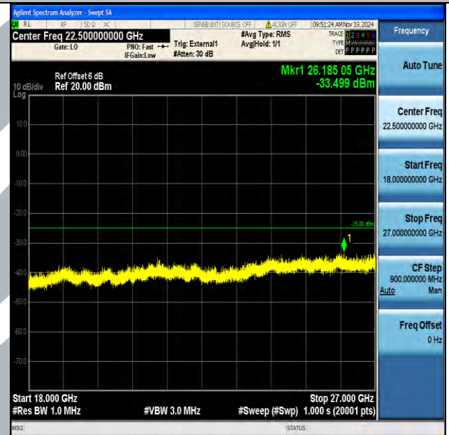
Band38_15MHz_16QAM_38175_1RB#0_18000~27000_18000~27000
