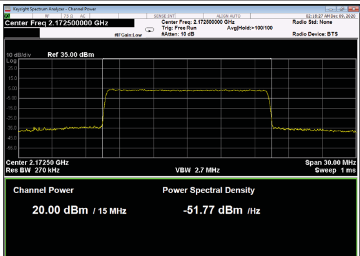
Figure 228: QPSK 15MHz B.W.; 2172.5MHz, 15kHz
