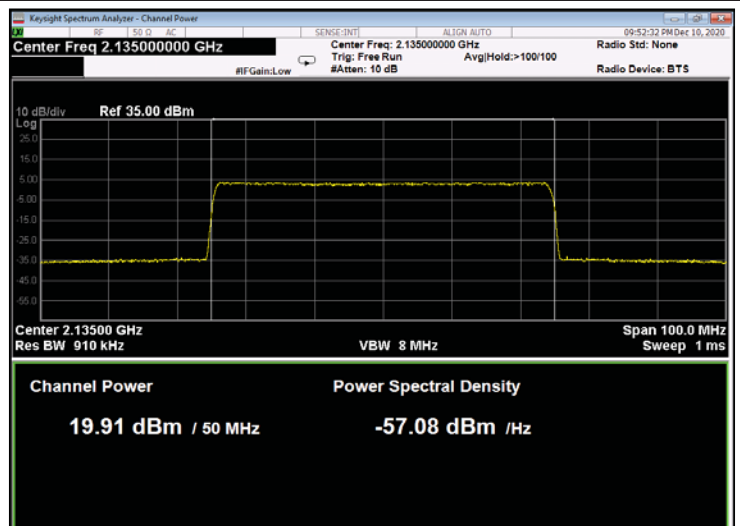
Figure 258: QPSK 50MHz B.W.; 2135.0MHz, 15kHz
