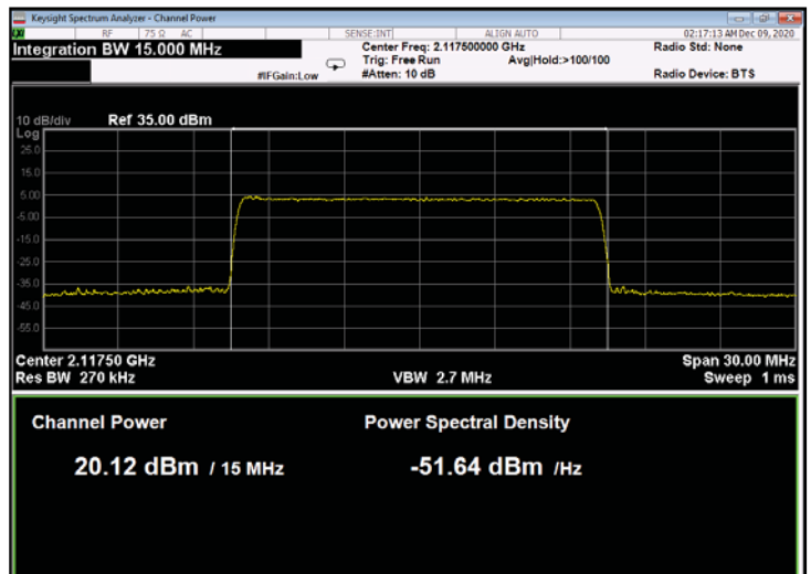
Figure 222: QPSK 15MHz B.W.; 2117.5MHz, 15kHz
