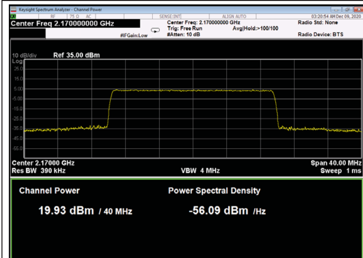
Figure 237: QPSK 20MHz B.W.; 2170.0MHz, 15kHz
