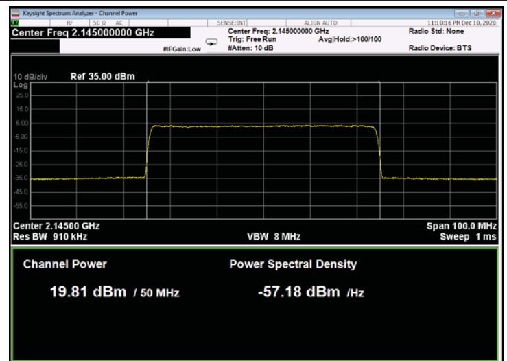
Figure 196: 256QAM 50MHz B.W.; 2145.0MHz, 30kHz
