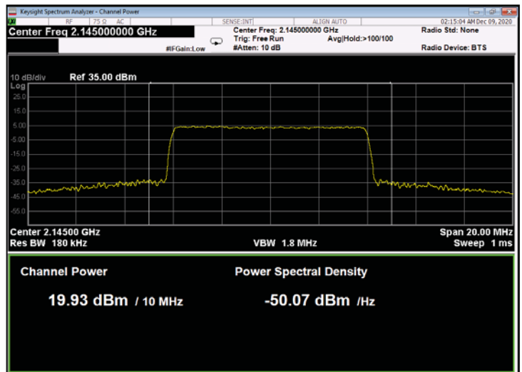
Figure 218: QPSK 10MHz B.W.; 2145.0MHz, 60kHz
