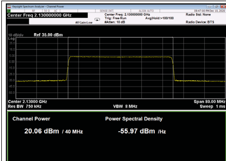
Figure 249: QPSK 40MHz B.W.; 2130.0MHz, 15kHz
