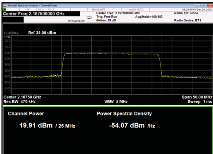
Figure 247: QPSK 25MHz B.W.; 2167.5MHz, 30kHz
