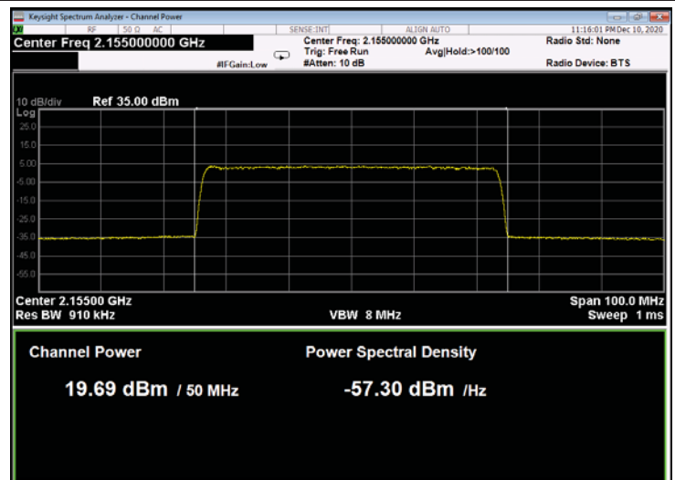
Figure 200: 256QAM 50MHz B.W.; 2155.0MHz, 60kHz
