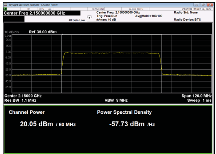
Figure 272: QPSK 60MHz B.W.; 2150.0MHz, 60kHz
