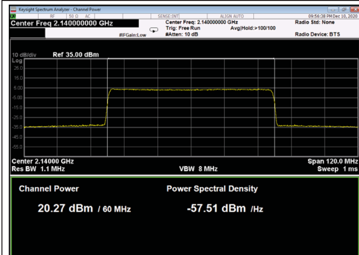
Figure 267: QPSK 60MHz B.W.; 2140.0MHz, 30kHz
