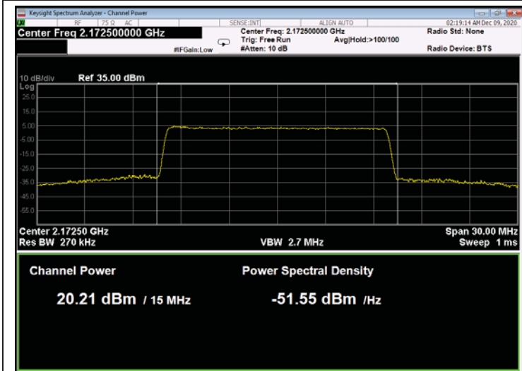
Figure 229: QPSK 15MHz B.W.; 2172.5MHz, 30kHz
