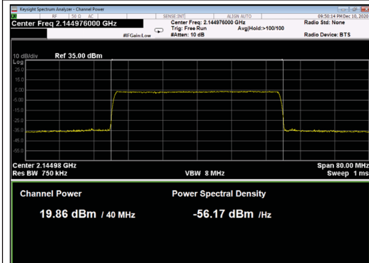
Figure 253: QPSK 40MHz B.W.; 2145.0MHz, 30kHz
