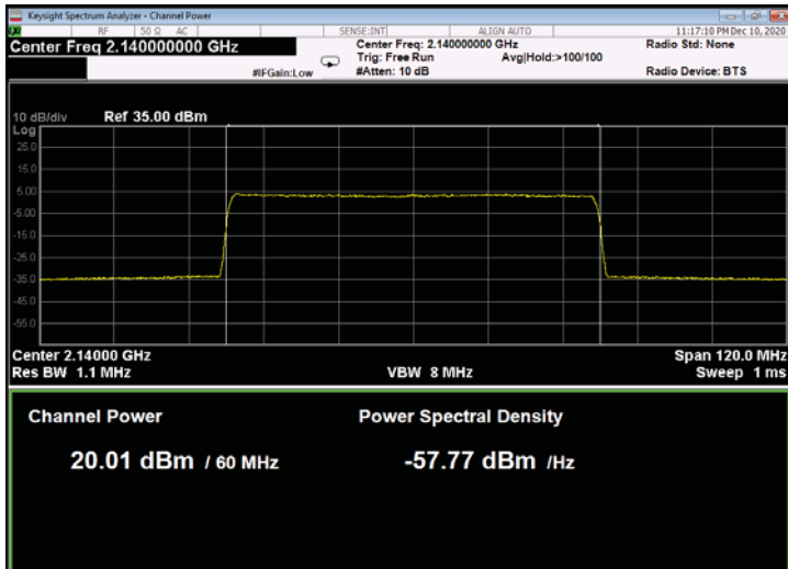
Figure 201: 256QAM 60MHz B.W.; 2140.0MHz, 30kHz
