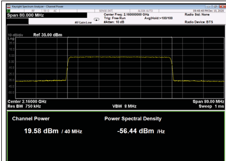
Figure 255: QPSK 40MHz B.W.; 2160.0MHz, 15kHz
