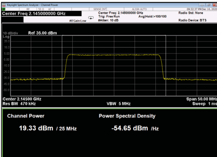
Figure 245: QPSK 25MHz B.W.; 2145.0MHz, 60kHz
