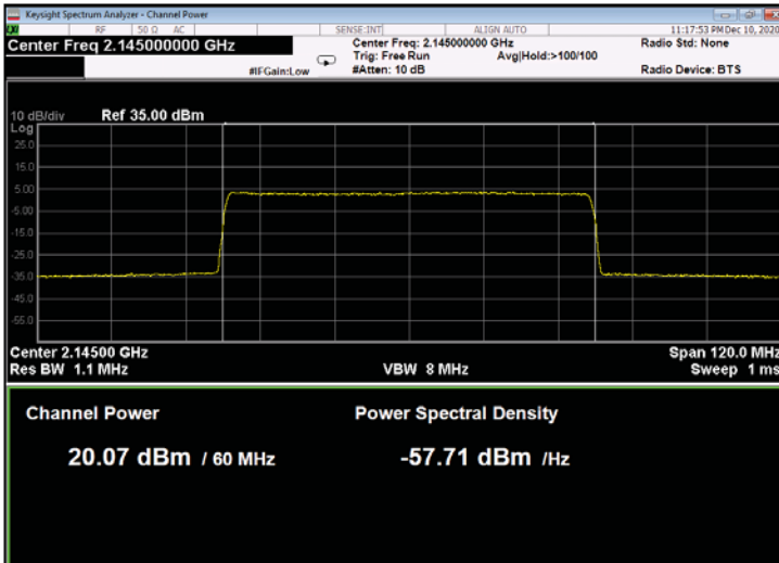
Figure 203: 256QAM 60MHz B.W.; 2145.0MHz, 30kHz
