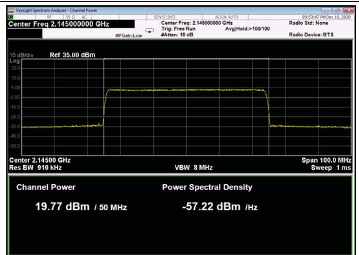
Figure 262: QPSK 50MHz B.W.; 2145.0MHz, 30kHz
