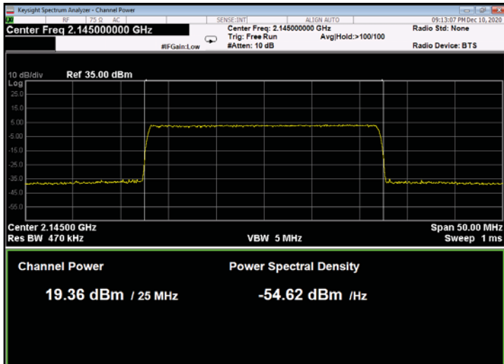
Figure 243: QPSK 25MHz B.W.; 2145.0MHz, 15kHz
