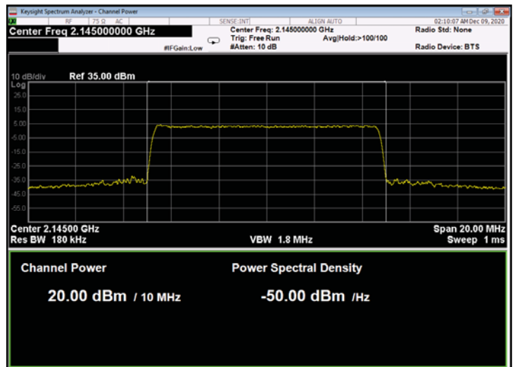
Figure 216: QPSK 10MHz B.W.; 2145.0MHz, 15kHz
