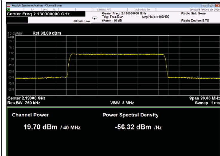
Figure 251: QPSK 40MHz B.W.; 2130.0MHz, 60kHz
