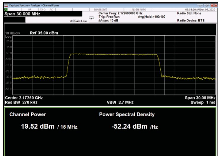
Figure 230: QPSK 15MHz B.W.; 2172.5MHz, 60kHz
