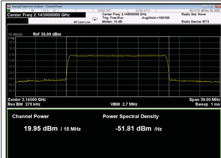
Figure 225: QPSK 15MHz B.W.; 2145.0MHz, 15kHz
