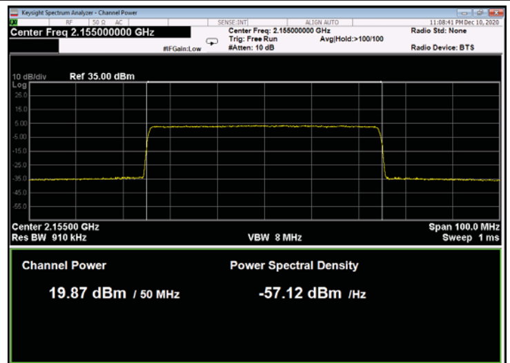
Figure 198: 256QAM 50MHz B.W.; 2155.0MHz, 15kHz
