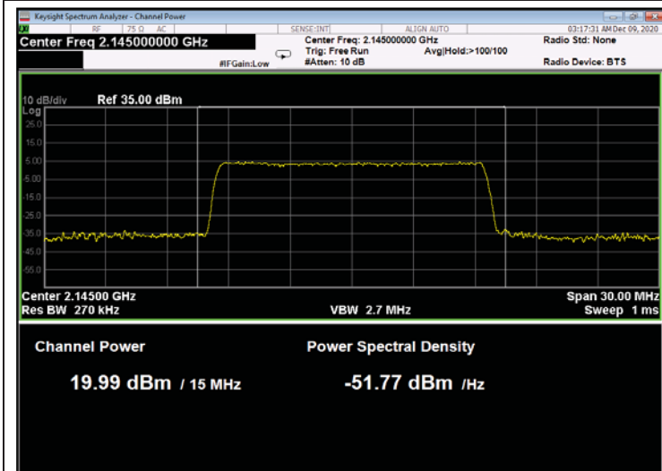
Figure 227: QPSK 15MHz B.W.; 2145.0MHz, 60kHz
