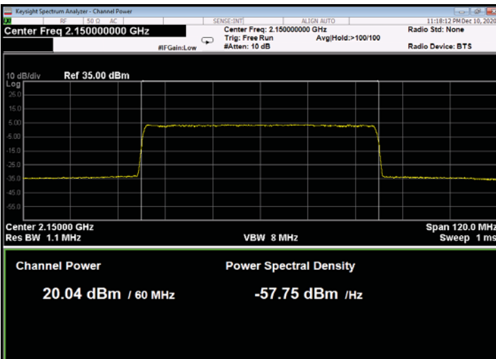
Figure 205: 256QAM 60MHz B.W.; 2150.0MHz, 30kHz
