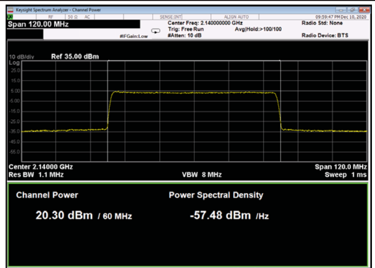
Figure 268: QPSK 60MHz B.W.; 2140.0MHz, 60kHz
