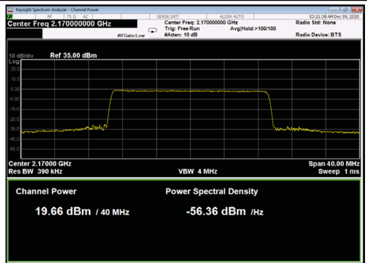
Figure 238: QPSK 20MHz B.W.; 2170.0MHz, 30kHz
