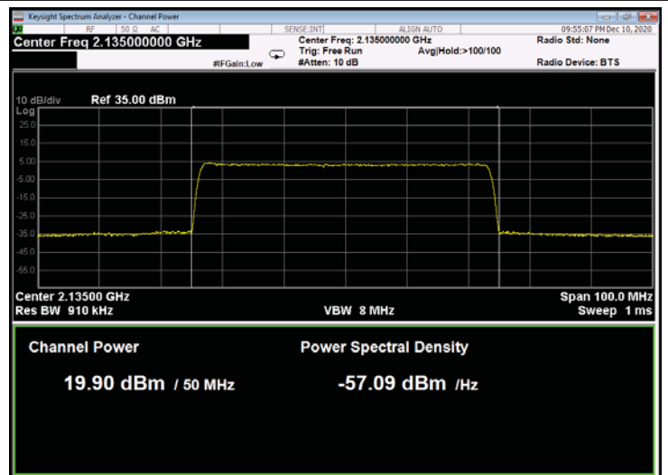
Figure 260: QPSK 50MHz B.W.; 2135.0MHz, 60kHz
