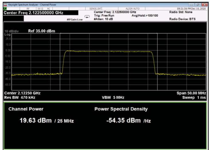
Figure 242: QPSK 25MHz B.W.; 2122.5MHz, 60kHz
