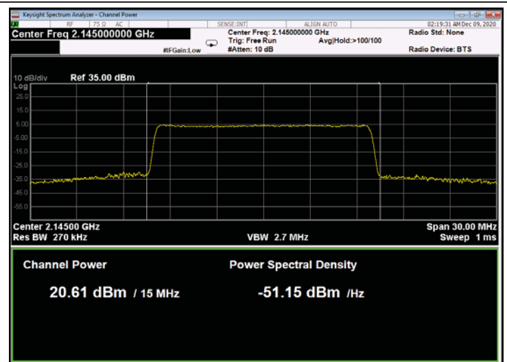
Figure 226: QPSK 15MHz B.W.; 2145.0MHz, 30kHz
