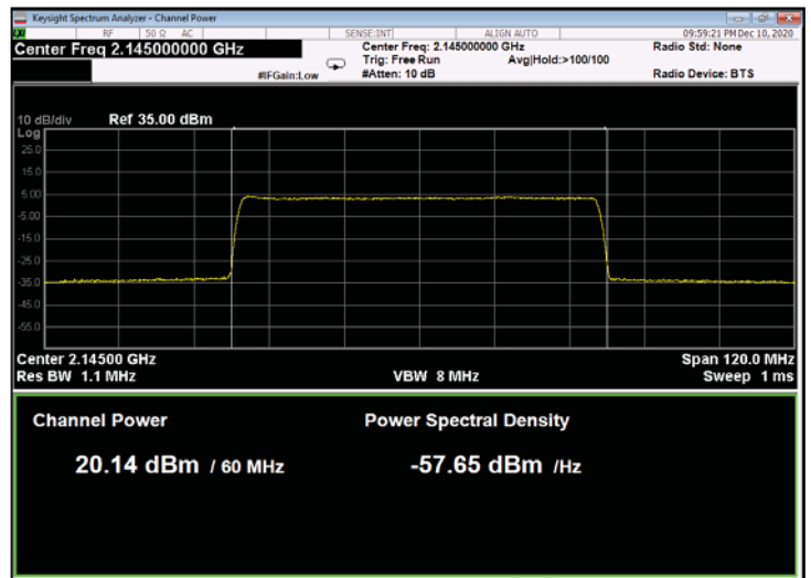
Figure 270: QPSK 60MHz B.W.; 2145MHz, 60kHz
