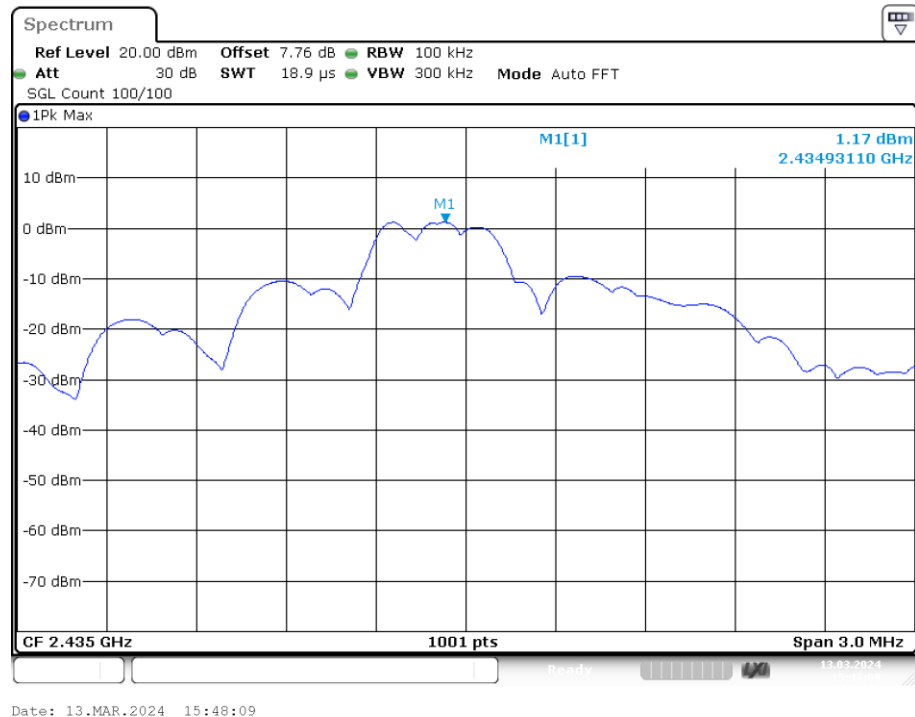
PSD NVNT GFSK 2435MHz Ant1
