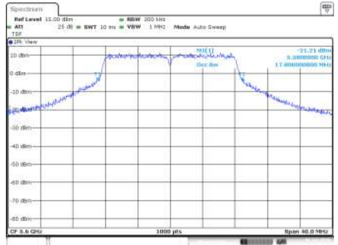
SISO A, CH120, 802.11a, 6Mbps, 99%
