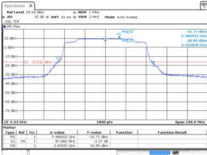
MIMO A, CH106, 802.11ac80, VHT0, 26dB
