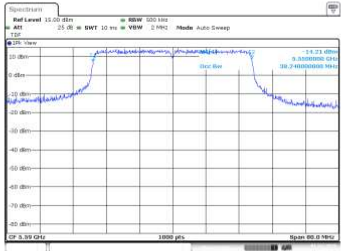
SISO A, CH118, 802.11ax40, HE0, 99%
