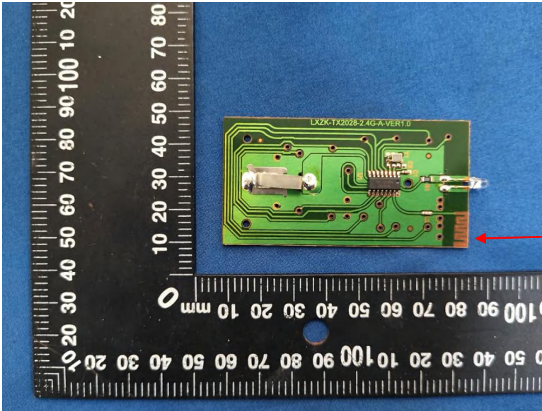
2.4G Antenna
