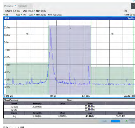
42(3550-3600)-20MHz-QPSK-43190-1RB#0-PASS
