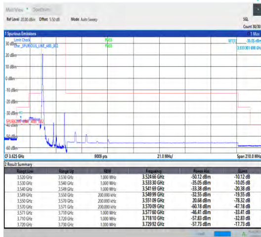
Band22_20MHz_QPSK_43190_1RB#0
