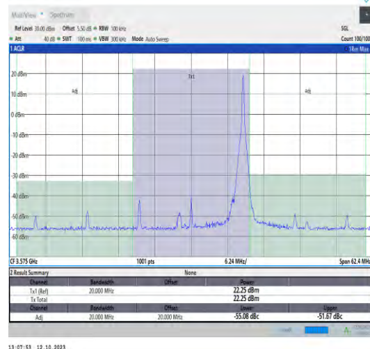
42(3550-3600)-20MHz-QPSK-43340-1RB#99-PASS
