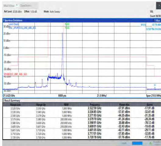
Band22_20MHz_QPSK_43490_1RB#99
