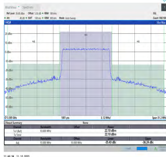
42(3550-3600)-10MHz-QPSK-43540-50RB#0-PASS
