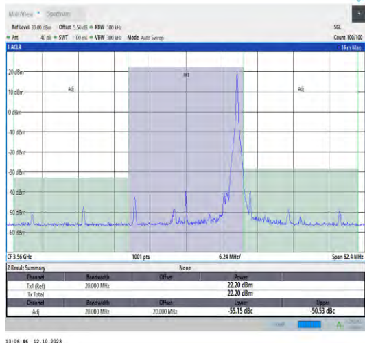
42(3550-3600)-20MHz-QPSK-43190-1RB#99-PASS
