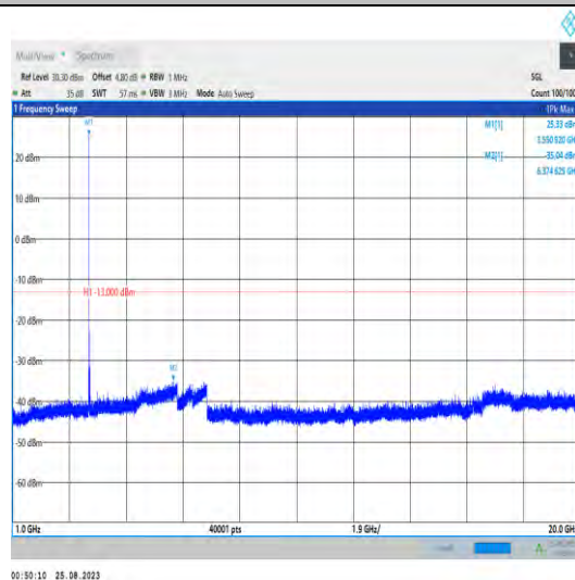
Band42_20MHz_QPSK_43190_1RB#0_1000~20000_1000~20000 000~20000
