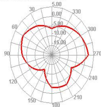
5500.000MHz E2
