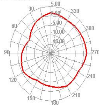
5500.000MHz H
