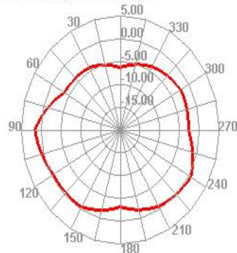
5500.000MHz E1
