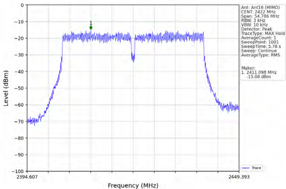
802.11n(HT40)_LCH_2422MHz_Ant16 (MIMO)_NTNV
