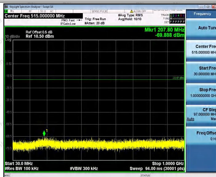
11N20_Ant1_2412_30~1000
