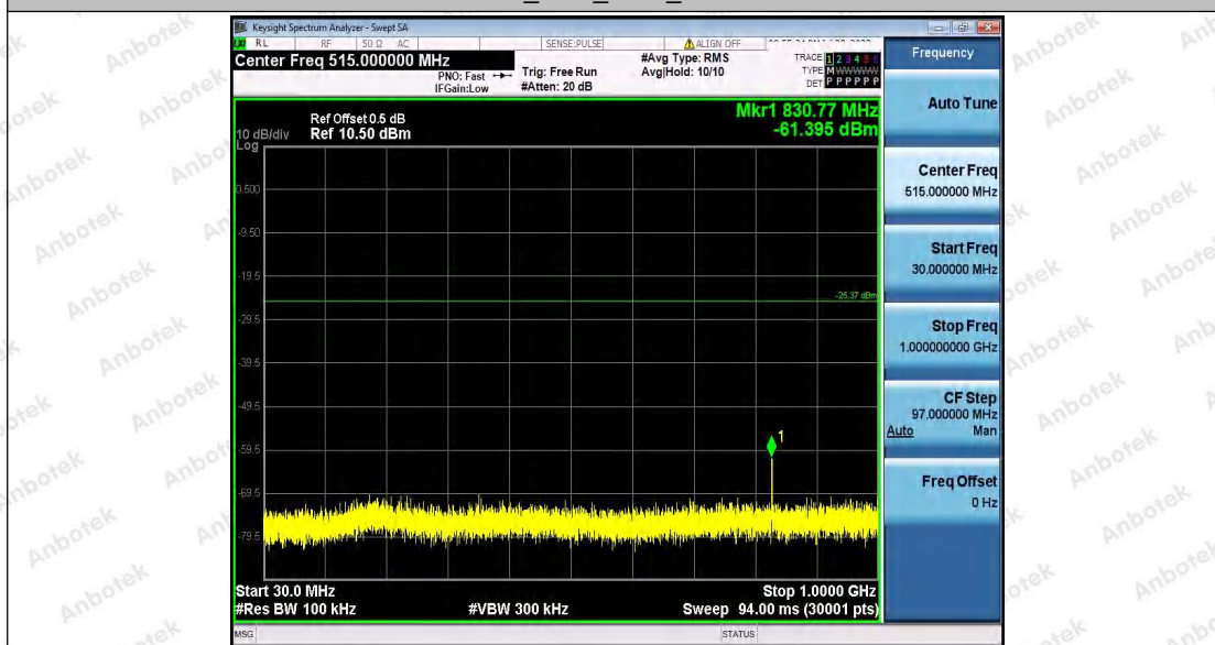
11N40_Ant1_2452_30~1000
