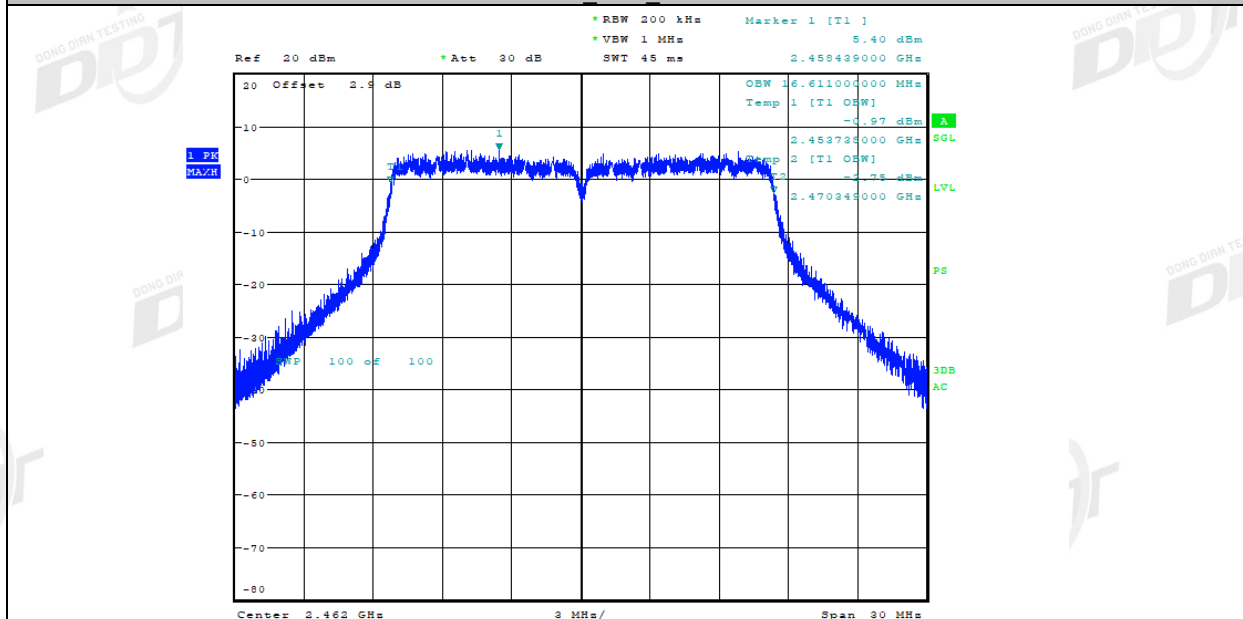
11G_Ant1_2462
