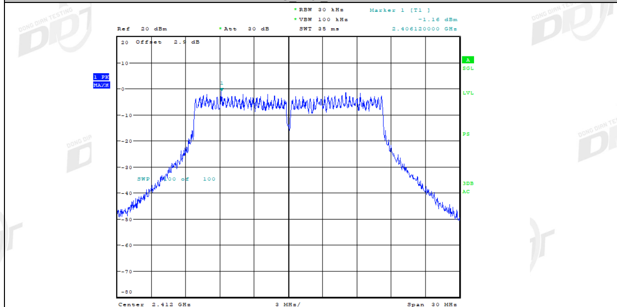
11G Ant1 2412
