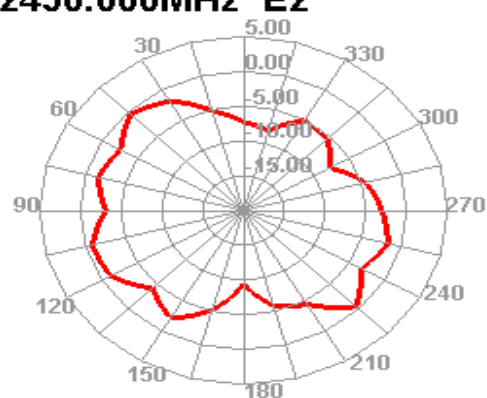
2450.000MHz E2
