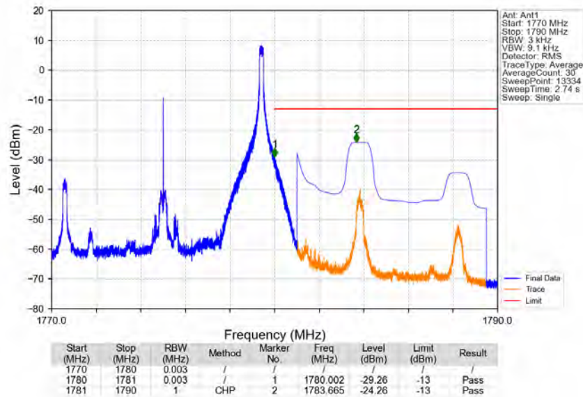
Band66_10MHz_QPSK_HCH_1775MHz_RB_1_49_NTNV
