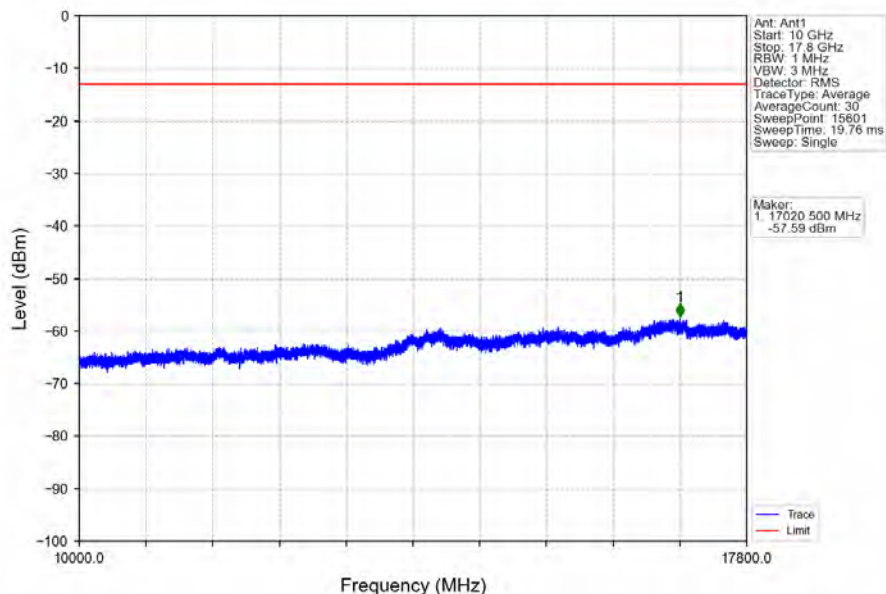
Band66_20MHz_QPSK_MCH_1745MHz_RB_1_0_NTNV
