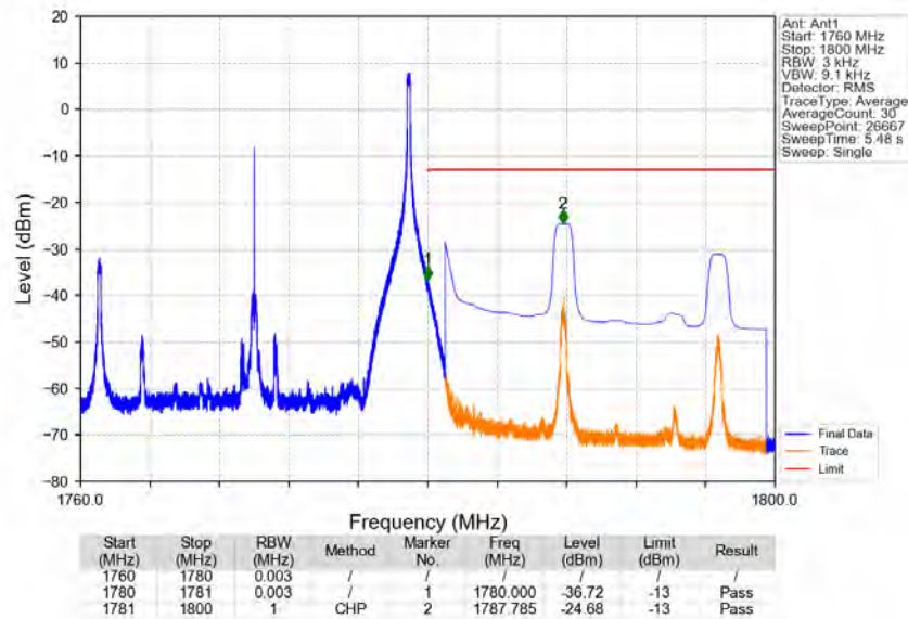
Band66_20MHz_QPSK_HCH_1770MHz_RB_1_99_NTNV
