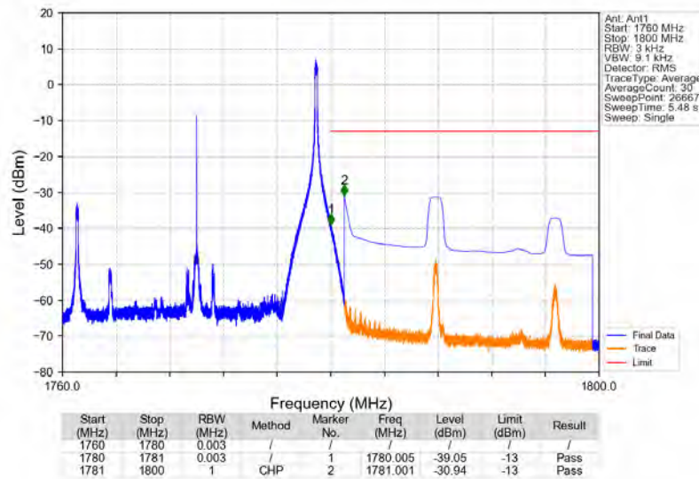
Band66 20MHz 64QAM HCH 1770MHz RB 1 99 NTNV
