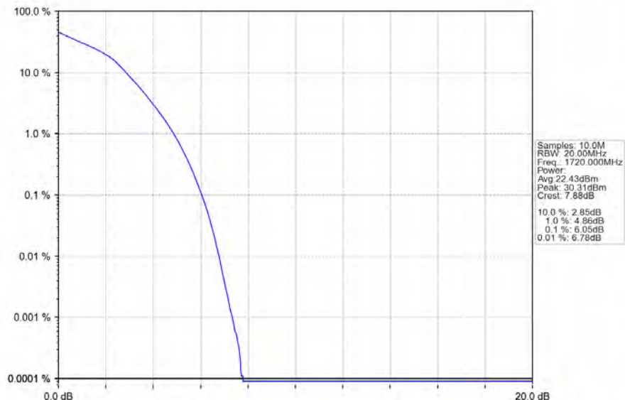
Band66_20MHz_16QAM_LCH_1720MHz_RB_100_0_NTNV
