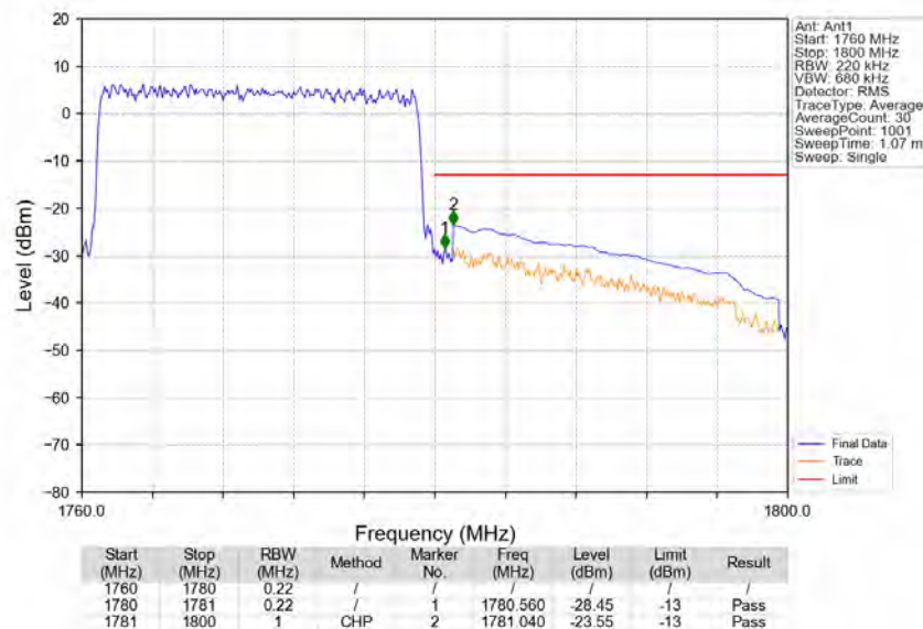
Band66_20MHz_QPSK_HCH_1770MHz_RB_100_0_NTNV
