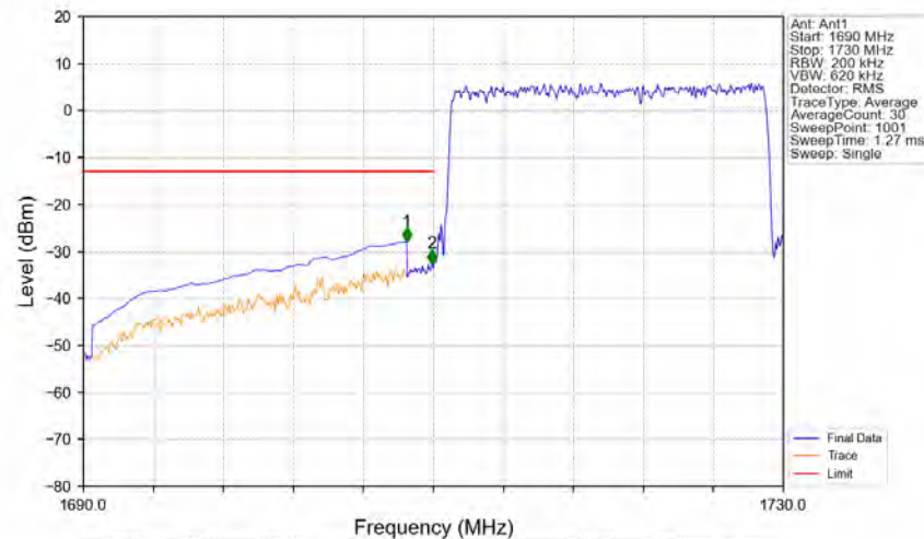
Band66_20MHz_QPSK_LCH_1720MHz_RB_100_0_NTNV
