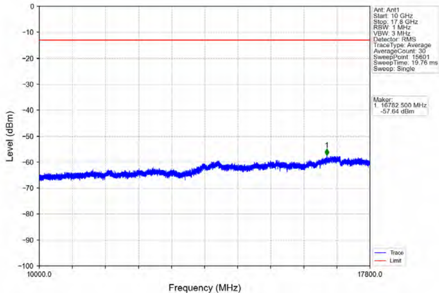
Band66_20MHz_16QAM_LCH_1720MHz_RB_100_0_NTNV
