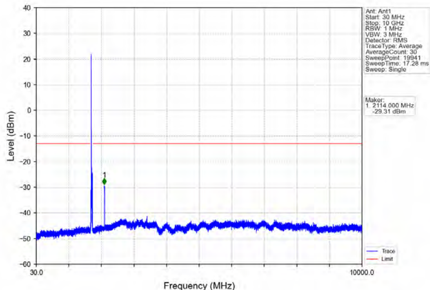
Band66_20MHz_16QAM_LCH_1720MHz_RB_1_0_NTNV
