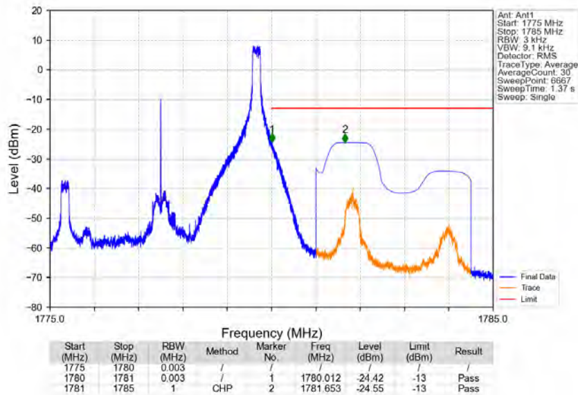
Band66_5MHz_QPSK_HCH_1777.5MHz_RB_1_24_NTNV
