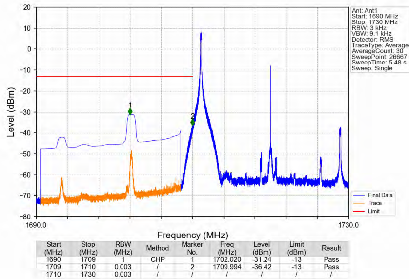
Band66_20MHz_16QAM_LCH_1720MHz_RB_1_0_NTNV
