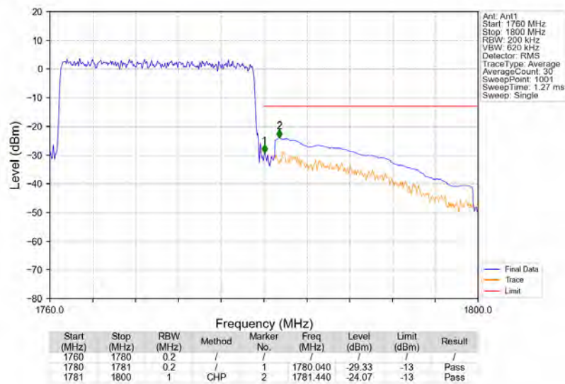
Band66 20MHz 64QAM HCH 1770MHz RB 100 0 NTNV
