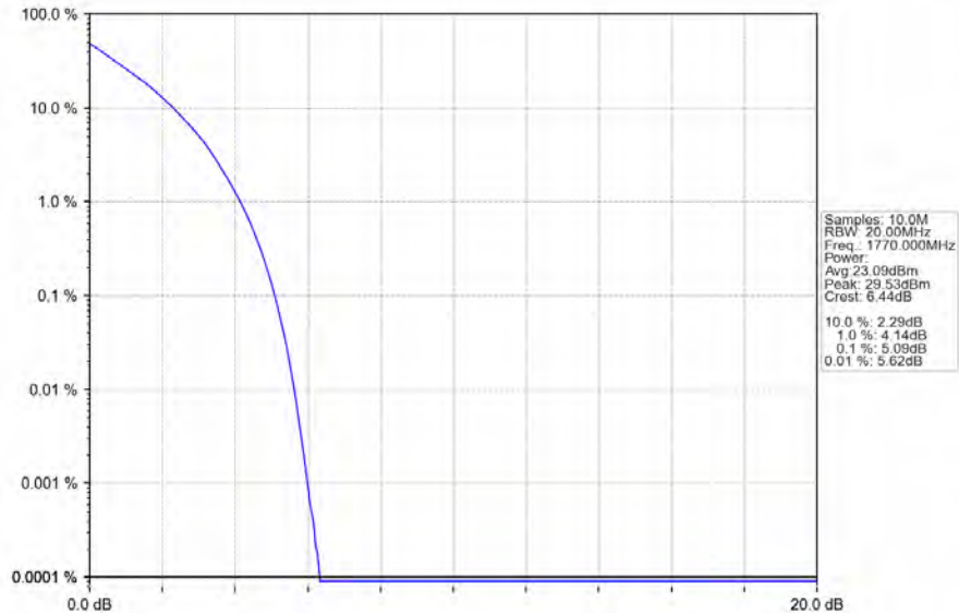
Band66_20MHz_QPSK_HCH_1770MHz_RB_100_0_NTNV
