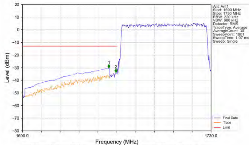
Band66_20MHz_16QAM_LCH_1720MHz_RB_100_0_NTNV
