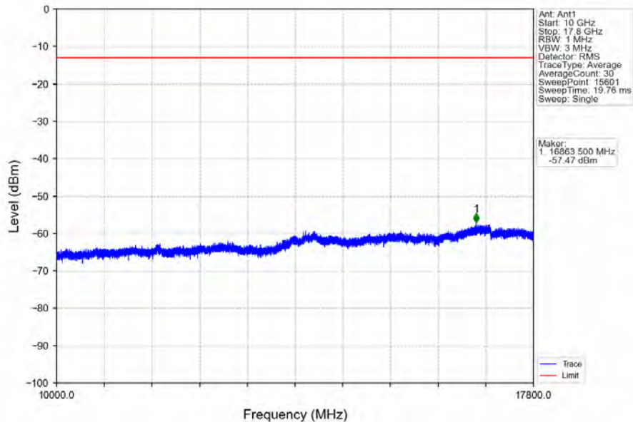
Band66_20MHz_QPSK_LCH_1720MHz_RB_100_0_NTNV
