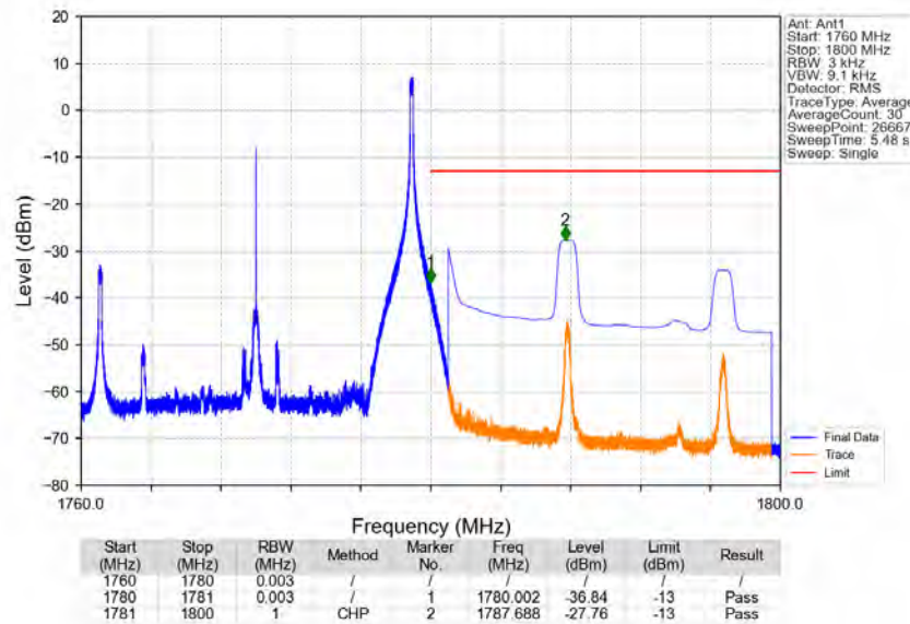
Band66_20MHz_16QAM_HCH_1770MHz_RB_1_99_NTNV
