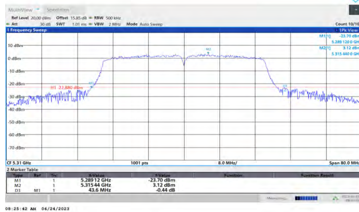
11N40MIMO_Ant2_5310
