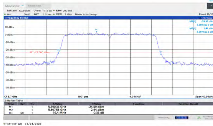
11N20MIMO_Ant2_5700
