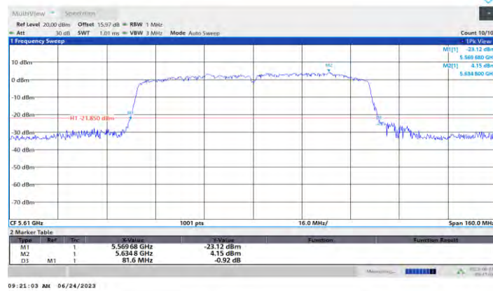
11AC80MIMO_Ant2_5610
