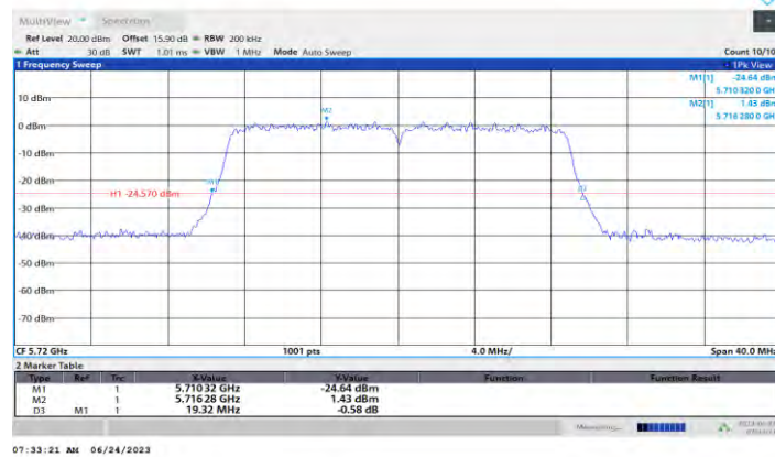
11N20MIMO_Ant1_5720
