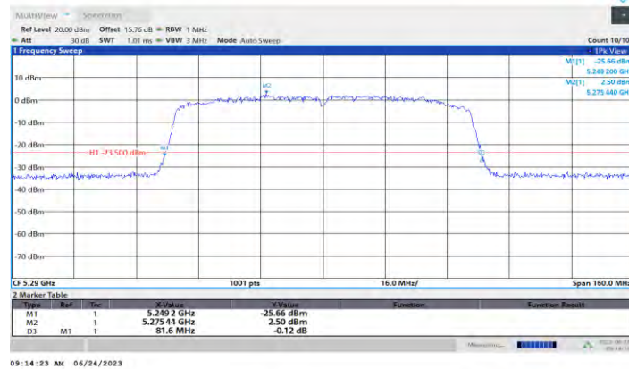
11AC80MIMO_Ant1_5290
