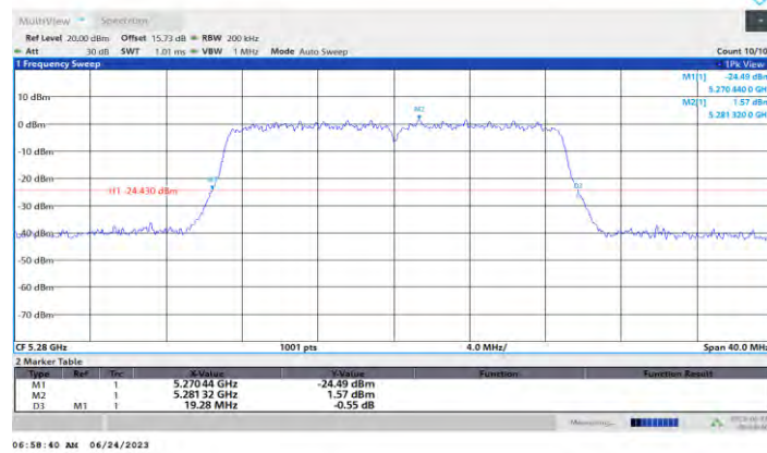
11N20MIMO_Ant1_5280
