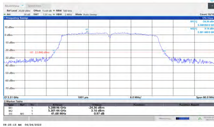
11N40MIMO_Ant1_5310
