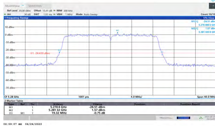
11N20MIMO_Ant2_5280
