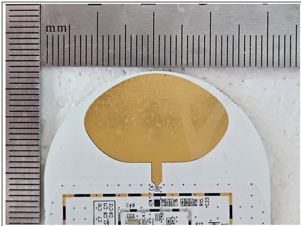
<UWB Antenna>
