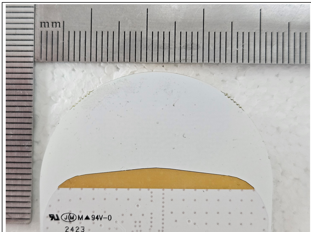
<UWB Antenna>
