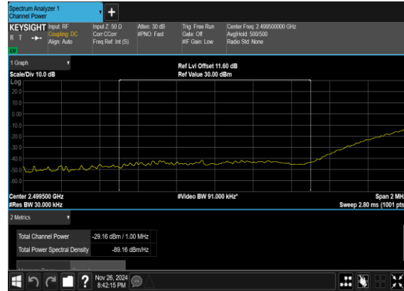
N7(50M)_CP-OFDM_QPSK _Edge_1RB_Left_Low_CH_chp_PASS
