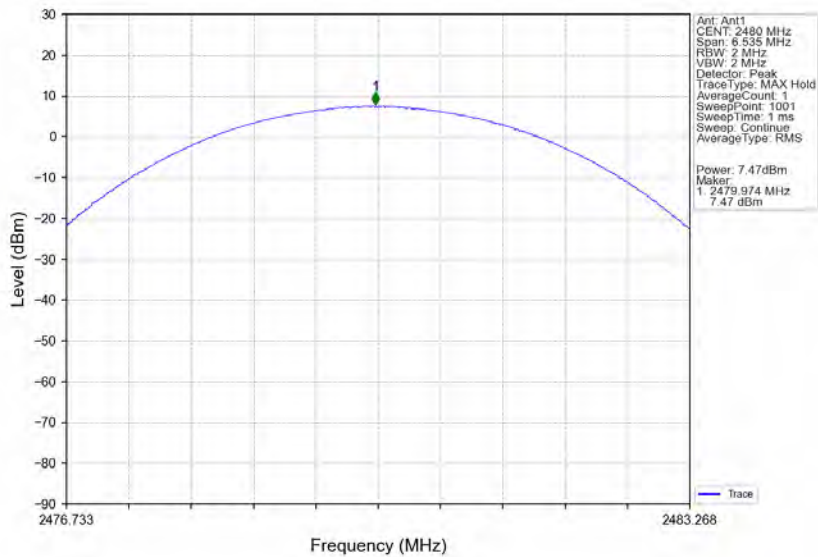
8DPSK 3DH5 HCH 2480MHz Ant1 NTNV
