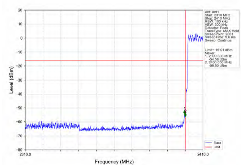
Pi/4DQPSK 2DH5 HOPP Ant1 NTV
