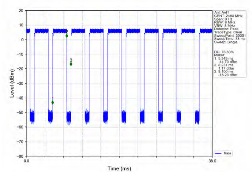
8DPSK 3DH5 HCH 2480MHz Ant1 NTN
