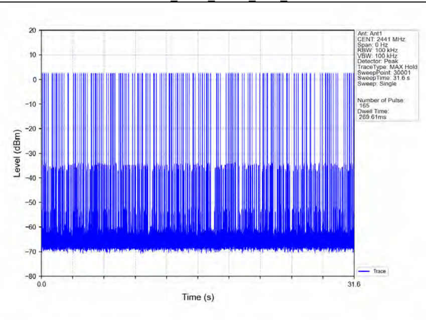
Pi/4DQPSK 2DH3 HOPP Ant1 NTN
