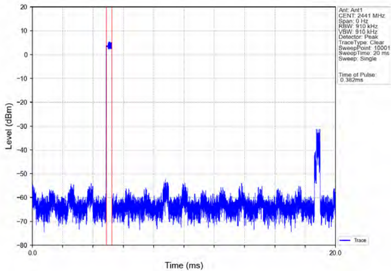
Pi/4DQPSK 2DH1 HOPP Ant1 NTV
