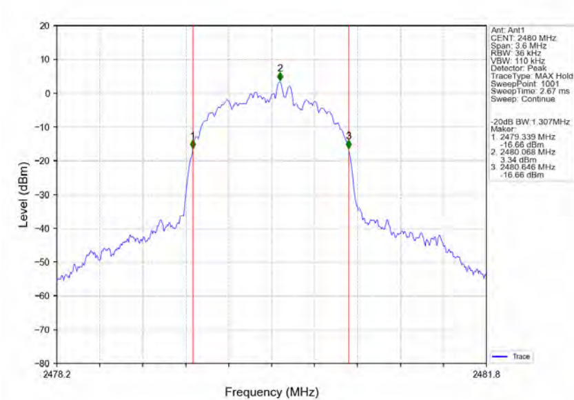
8DPSK 3DH5 HCH 2480MHz Ant1 NTVN
