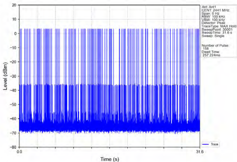
GFSK DH3 HOPP Ant1 NTN
