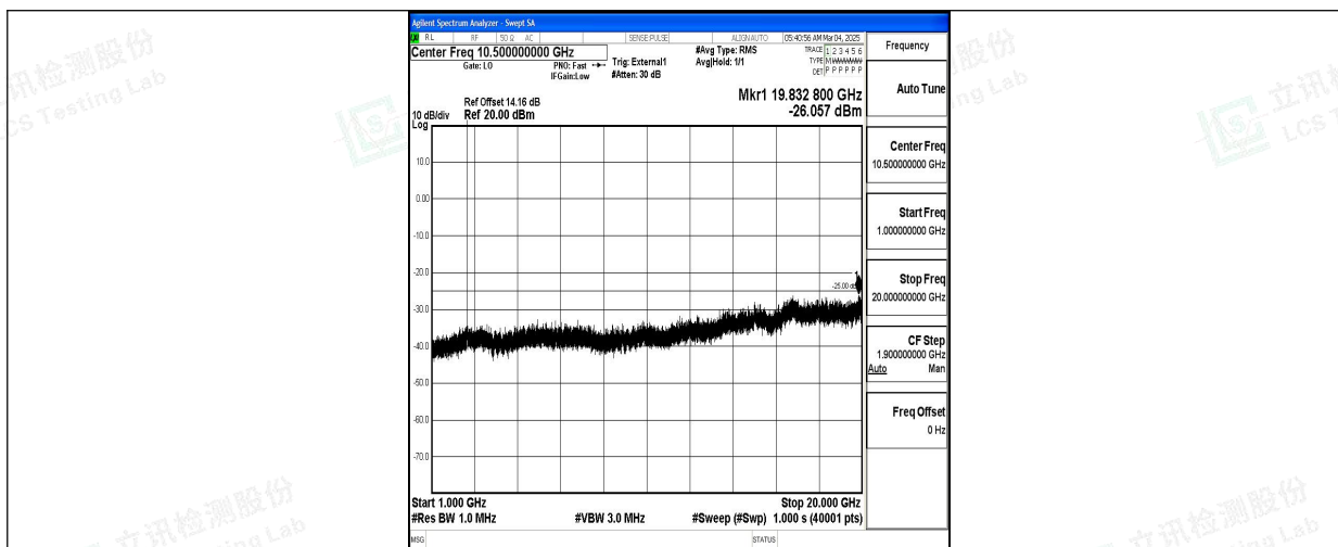
Band38 15MHz QPSK 37825 1RB#0 1000~20000 1000~20000
