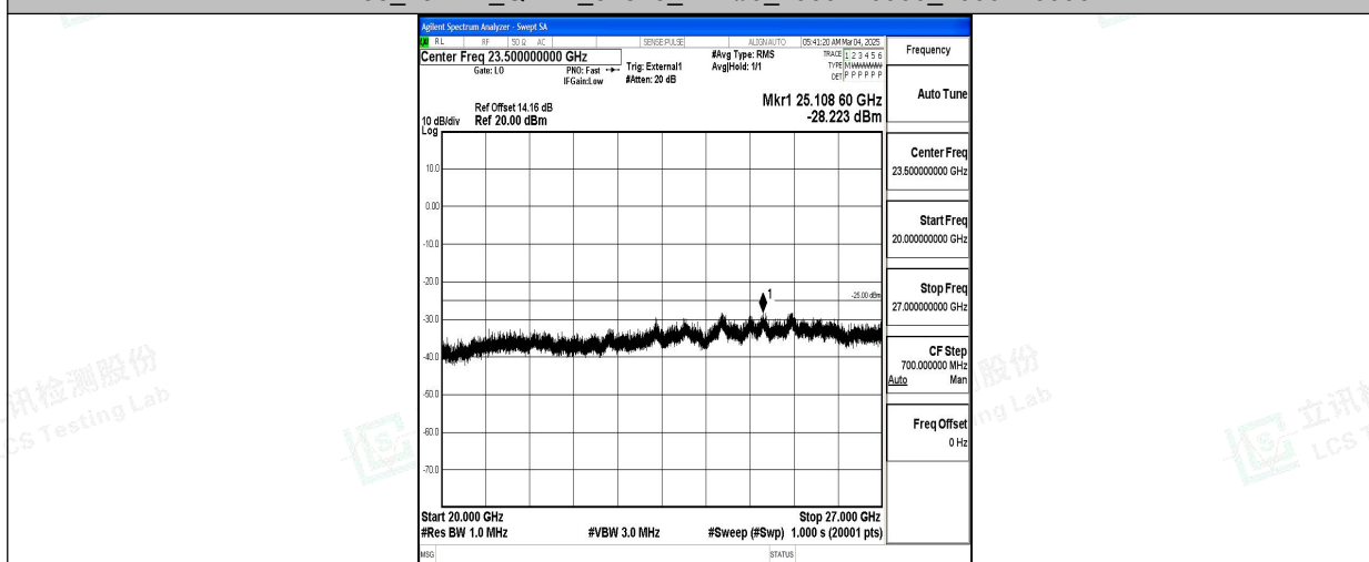
Band38 15MHz QPSK 37825 1RB#0 20000~27000 20000~27000
