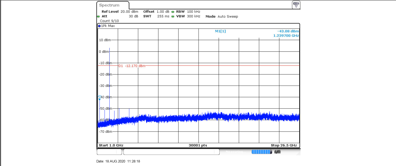
BLE Ant1 2480 1000~26500
