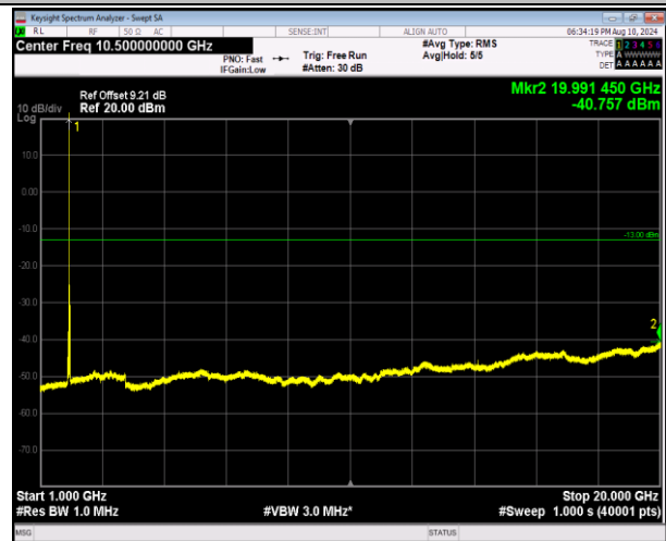
2-2-5MHz-20MHz-QPSK-QPSK-18808-18925-1RB#0-0RB# 0-1000~20000MHz-PASS
