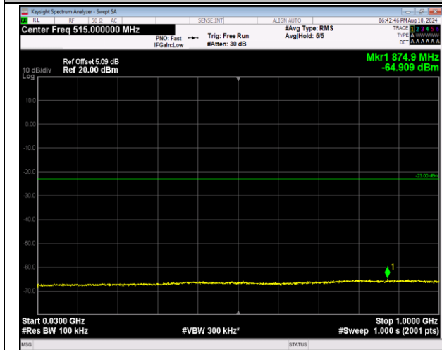
2-2-5MHz-20MHz-QPSK-QPSK-18983-19100-25RB#0-1 00RB#0-30~1000MHz-PASS
