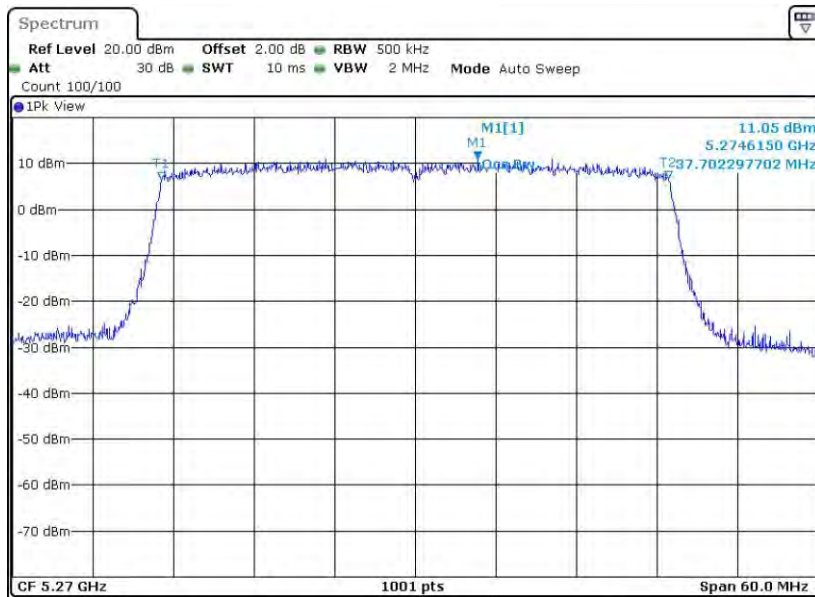
11AX40MIMO_Ant2_5270
