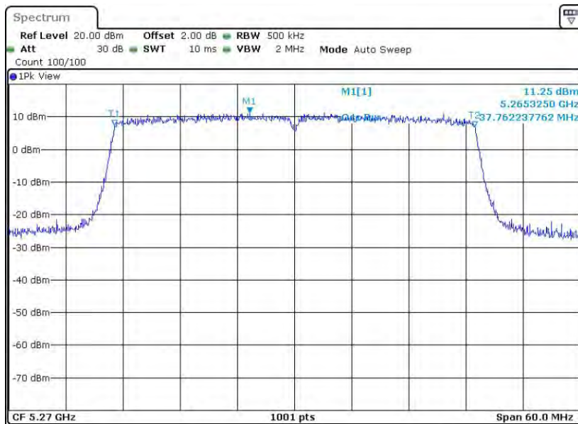
11AX40MIMO_Ant1_5270
