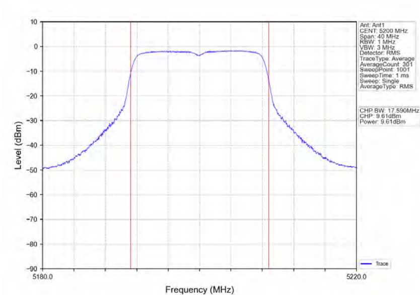
802.11a_MCH_5200MHz_Ant1_NTNV
