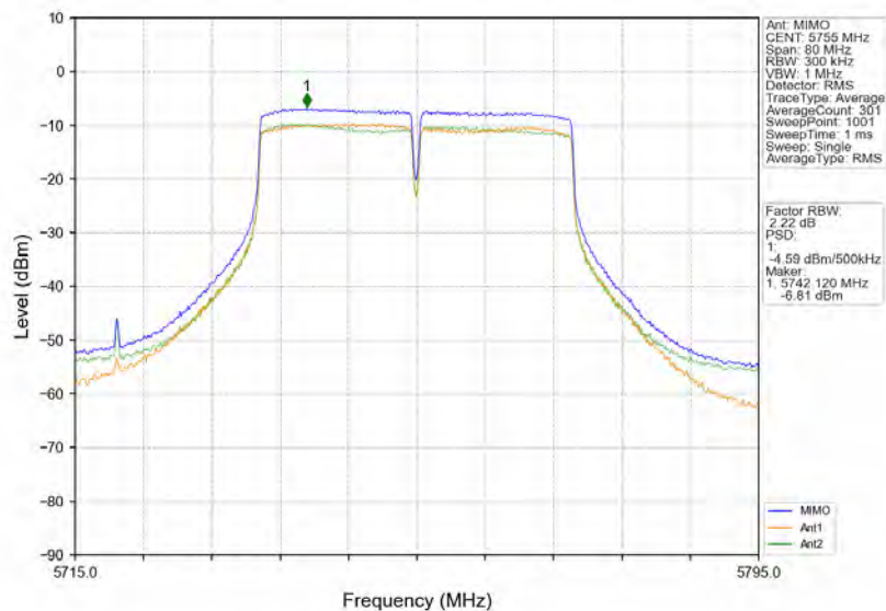
802.11n(HT40)_LCH_5755MHz_MIMO_NTNV
