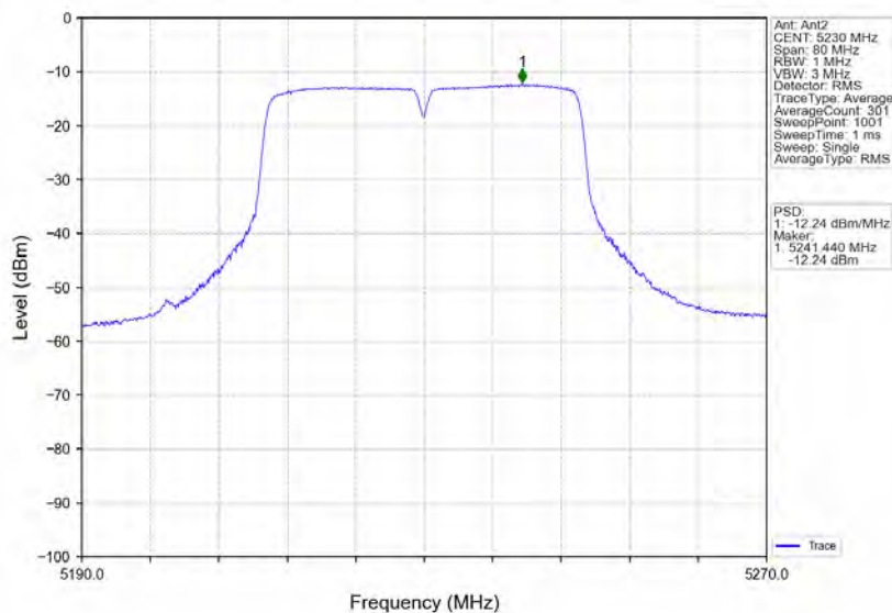
802.11n(HT40)_HCH_5230MHz_Ant2_NTNV
