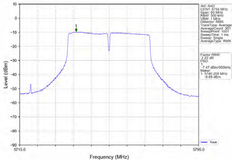
802.11n(HT40)_LCH_5755MHz_MIMO_NTNV
