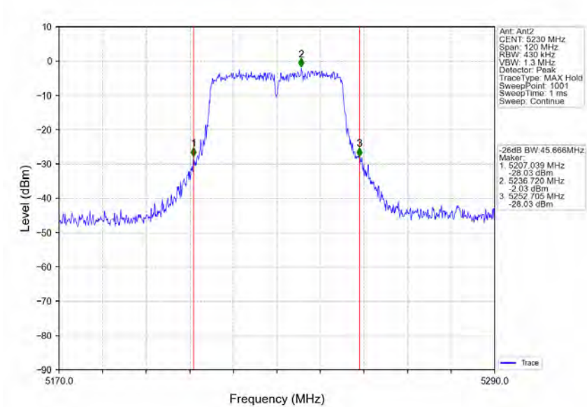
802.11n(HT40)_HCH_5230MHz_Ant2_NTNV
