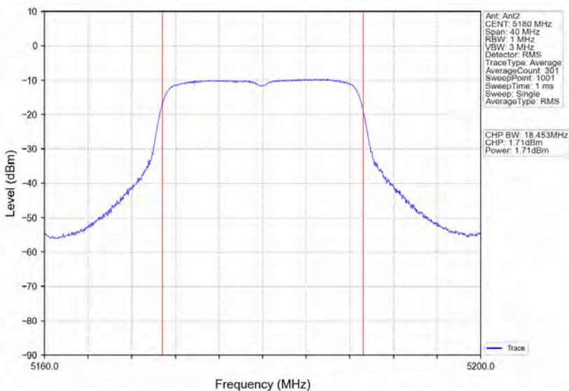
802.11n(HT20)_LCH_5180MHz_Ant2_NTNV
