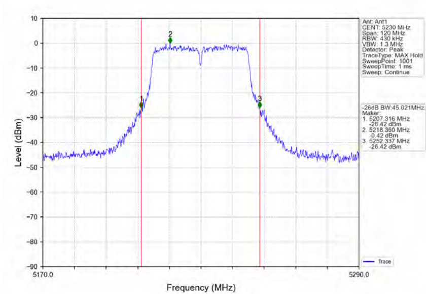
802.11n(HT40)_HCH_5230MHz_Ant1_NTNV
