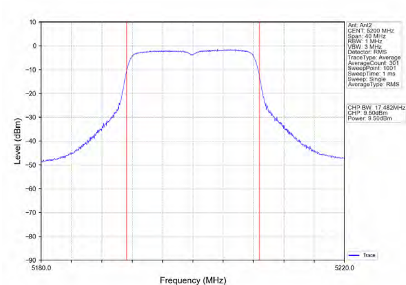
802.11a_MCH_5200MHz_Ant2_NTNV
