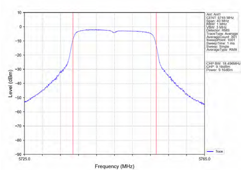
802.11n(HT20)_LCH_5745MHz_Ant1_NTNV
