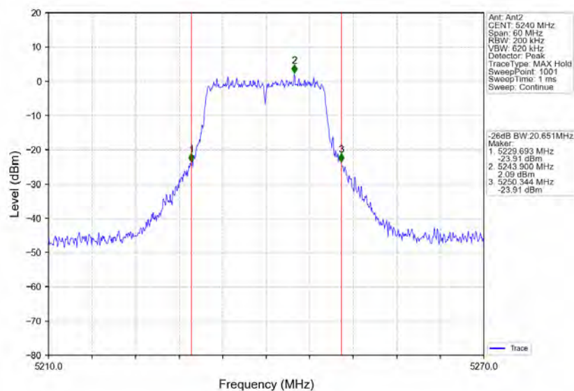
802.11a_HCH_5240MHz_Ant2_NTNV
