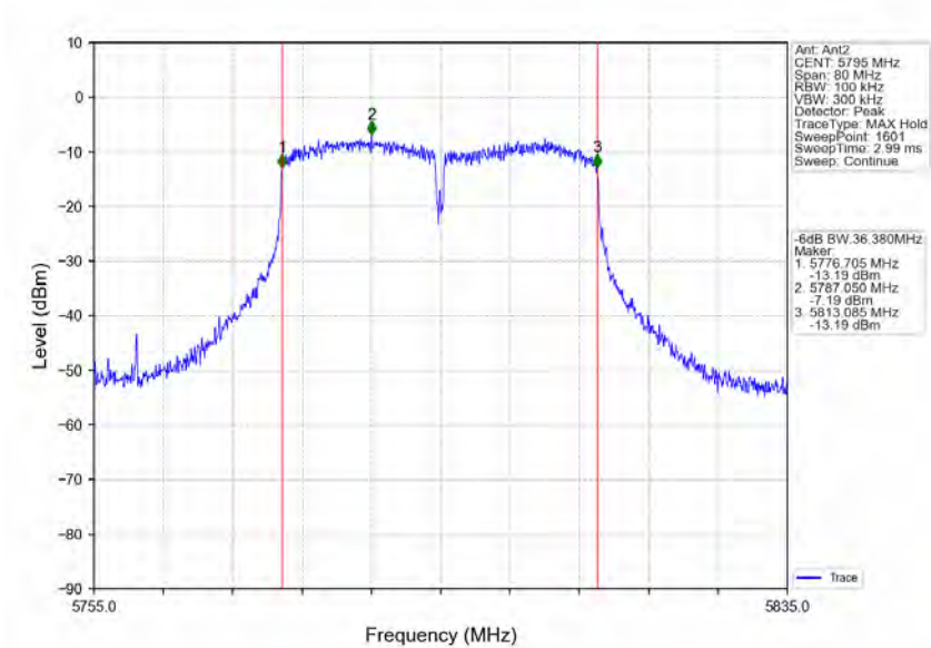
802.11n(HT40)_HCH_5795MHz_Ant2_NTNV
