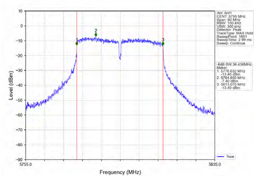
802.11n(HT40)_HCH_5795MHz_Ant1_NTNV
