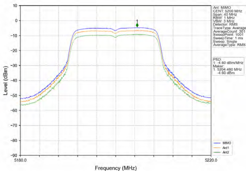
802.11n(HT20)_MCH_5200MHz_MIMO_NTNV
