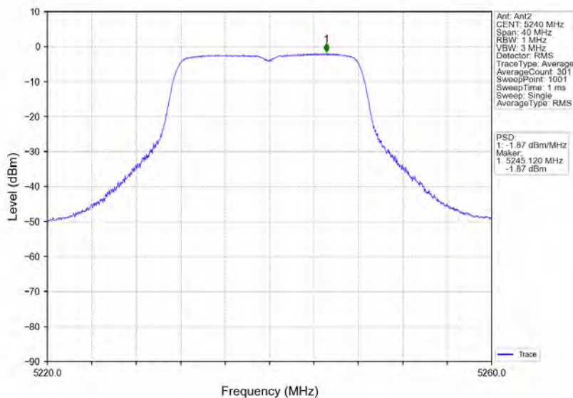
802.11a_HCH_5240MHz_Ant2_NTNV
