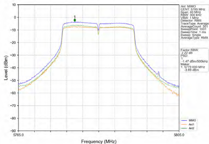
802.11n(HT20)_MCH_5785MHz_MIMO_NTNV
