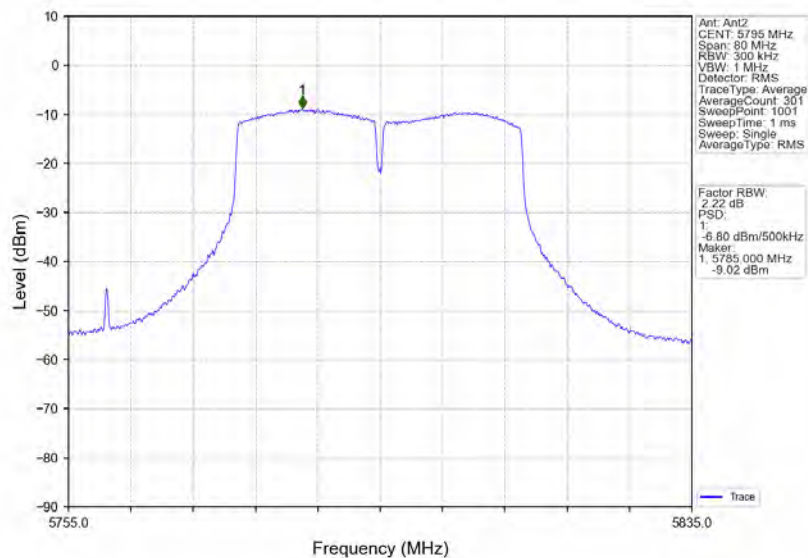
802.11n(HT40)_HCH_5795MHz_Ant2_NTNV
