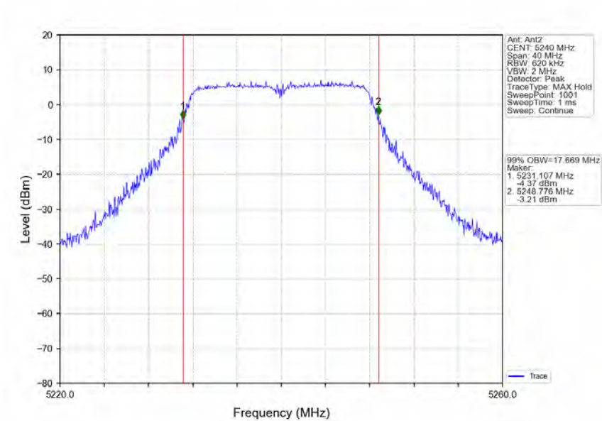
802.11a_HCH_5240MHz_Ant2_NTNV
