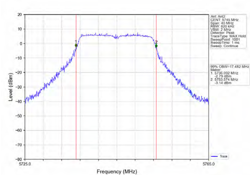
802.11a_LCH_5745MHz_Ant2_NTNV
