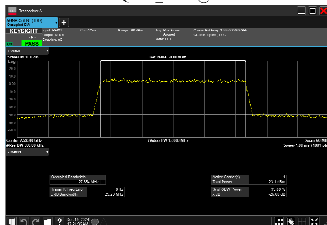
n38_30MHz_30kHz_2595MHz_CP-OFDM QPSK_RB78@0
