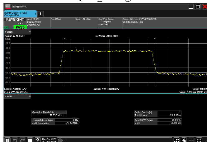
n38_30MHz_30kHz_2595MHz_CP-OFDM QPSK_RB78@0
