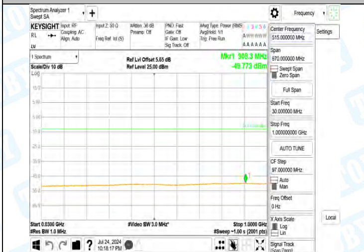
Band2-9538-3-30~1000MHz-PASS
