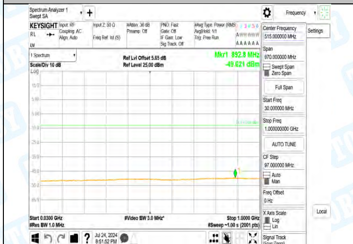
Band2-9538-3-30~1000MHz-PASS
