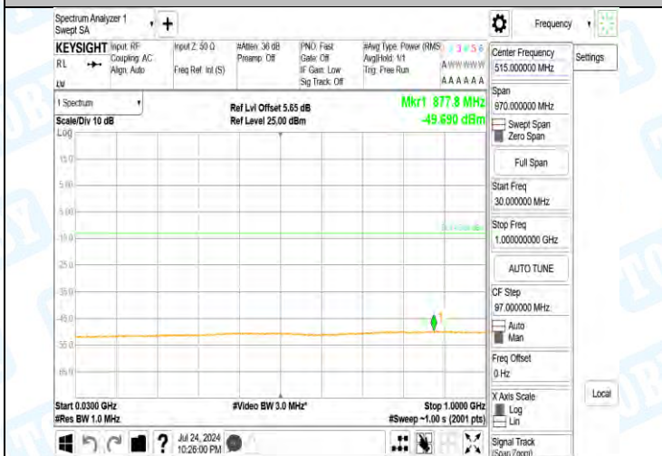
Band2-9538-5-30~1000MHz-PASS
