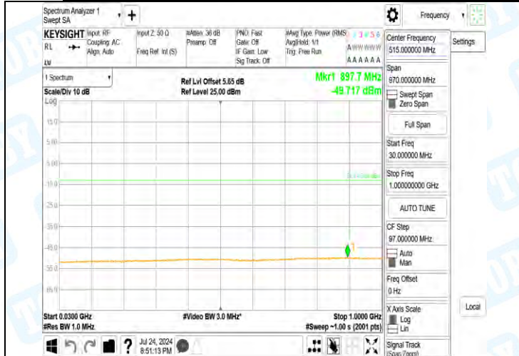
Band2-9400-3-30~1000MHz-PASS
