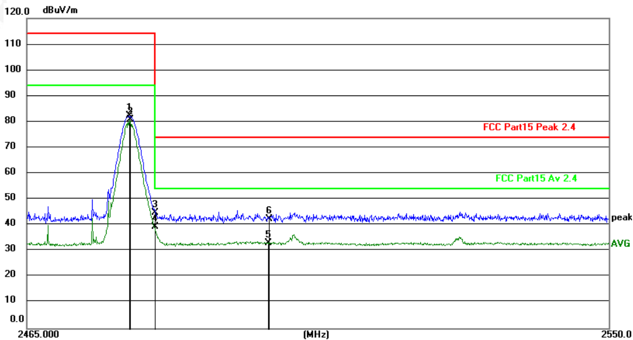
2480MHz Horizontal
