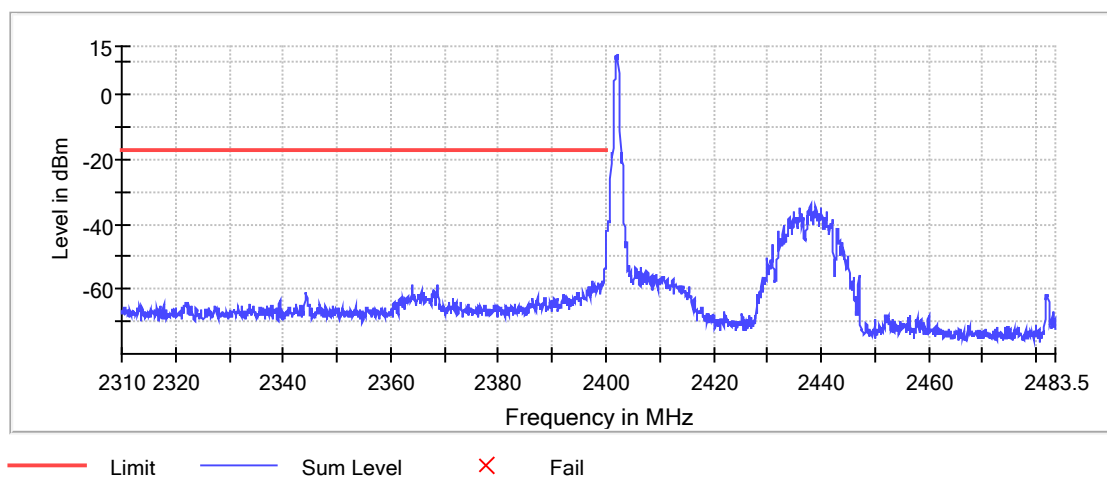
Band Edge
