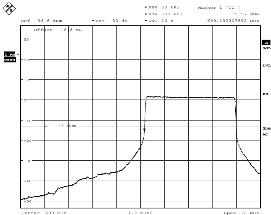
Diagram Ch 23035_QPSK_5MHZ
