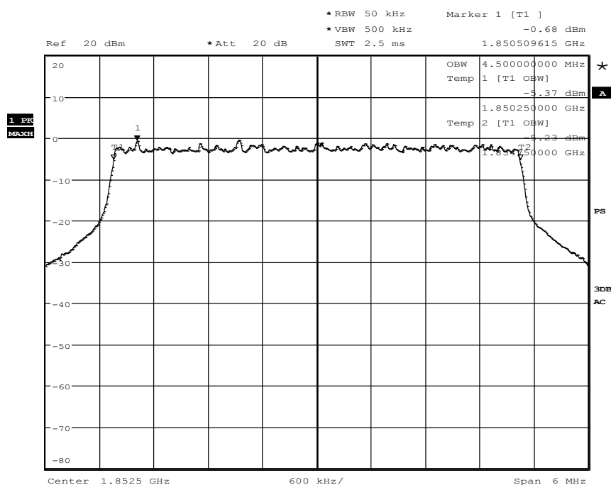
Diagram 35.208_OBW 5MHz Ch_19175
