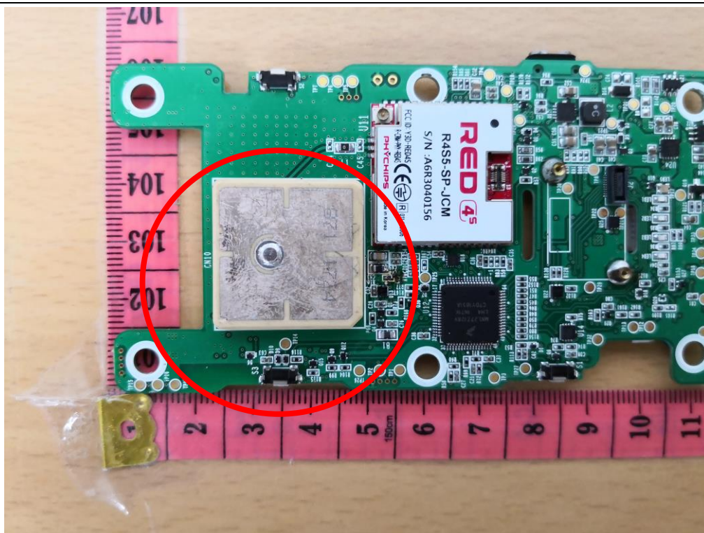
RFID Antenna
