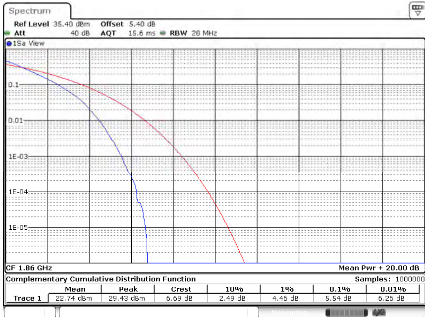
Band2-20MHz-QPSK-18700-100RB#0
