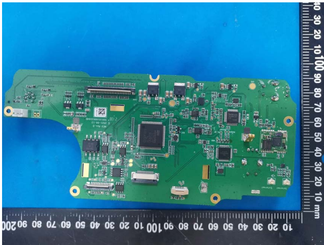
GNSS Module
