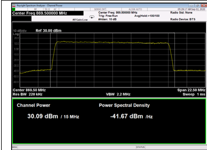
Figure 108: 256QAM 15MHz B.W.; 869.5MHz, 30kHz
