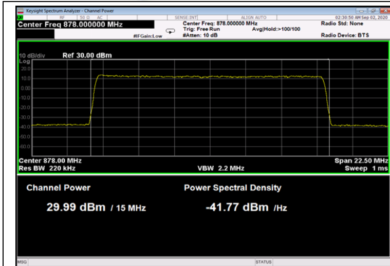
Figure 152: QPSK 15MHz B.W.; 878.0MHz, 15kHz
