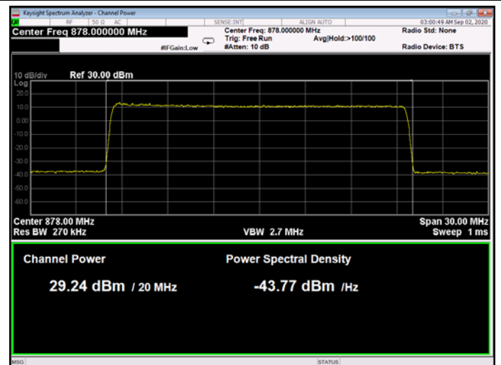
Figure 161: QPSK 20MHz B.W.; 878.0MHz, 15kHz
