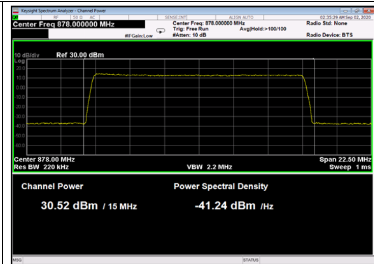
Figure 153: QPSK 15MHz B.W.; 878.0MHz, 30kHz
