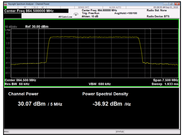
Figure 135: QPSK 5MHz B.W.; 864.5MHz, 30kHz
