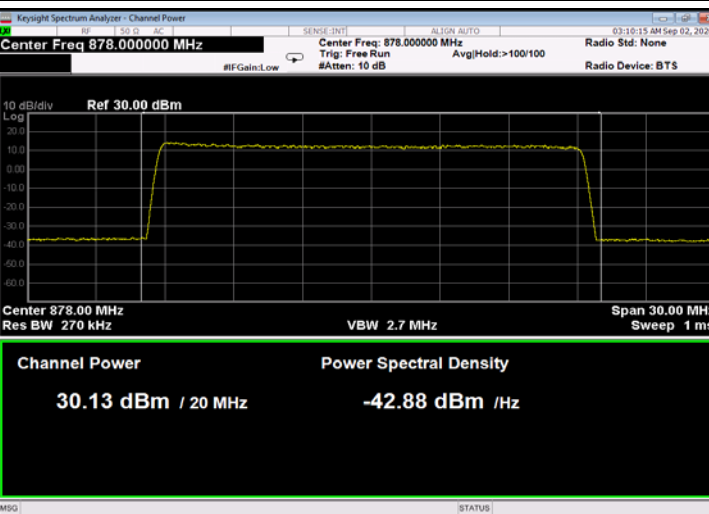
Figure 162: QPSK 20MHz B.W.; 878.0MHz, 30kHz
