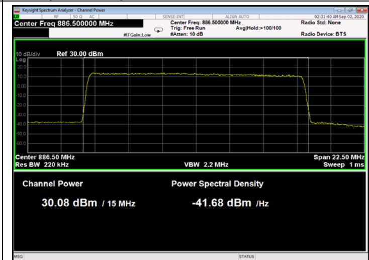
Figure 155: QPSK 15MHz B.W.; 886.5MHz, 15kHz
