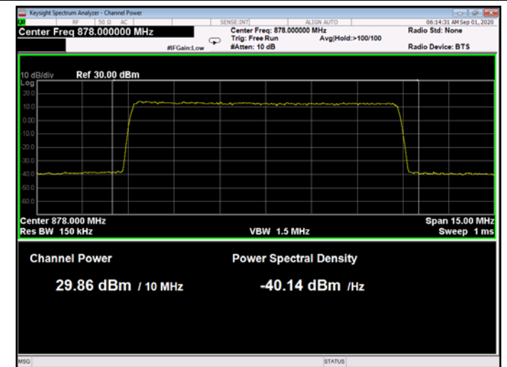
Figure 144: QPSK 10MHz B.W.; 878.0MHz, 30kHz
