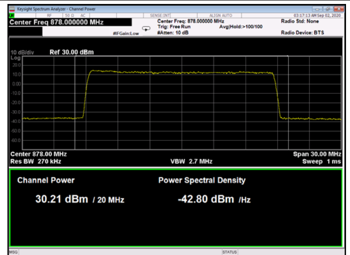
Figure 163: QPSK 20MHz B.W.; 878.0MHz, 60kHz
