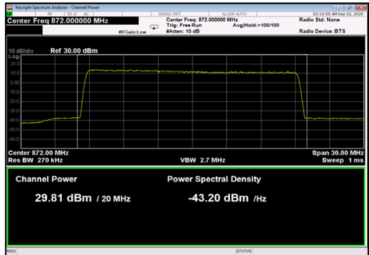
Figure 159: QPSK 20MHz B.W.; 872.0MHz, 30kHz
