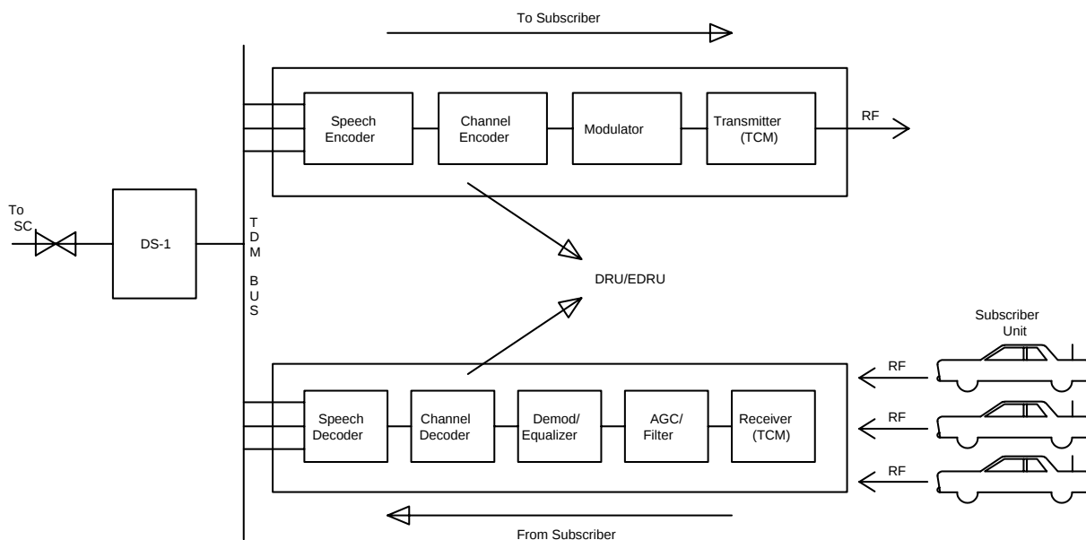
Figure 2-1. TDMA - DRU/EDRU To/From Subscriber
