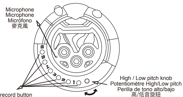
6 Phrase record button 6 Bouton d'enregistrement de phrases 6 Botón de grabación de frases 6段語音錄製按鍵
