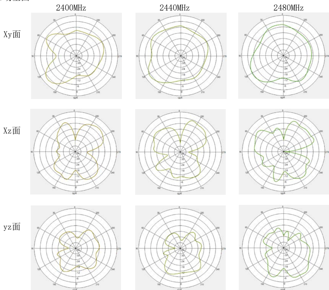
2D场型图
