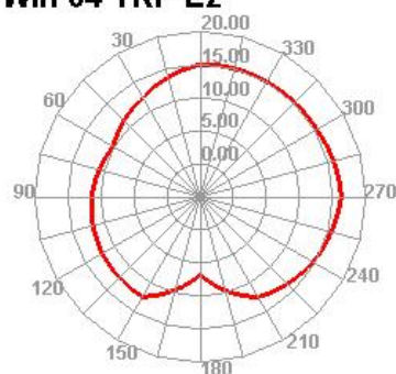
Wifi 64 TRP E2
