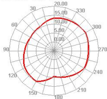
Wifi 36 TRP E2
