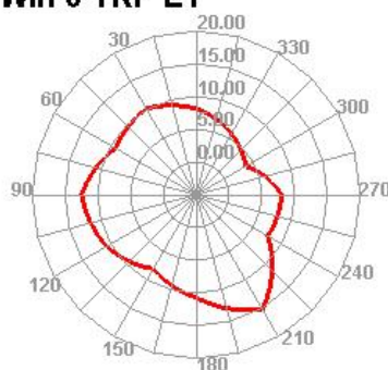
Wifi 6 TRP E1
