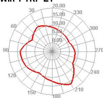
Wifi 1 TRP E1
