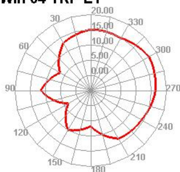
Wifi 64 TRP E1
