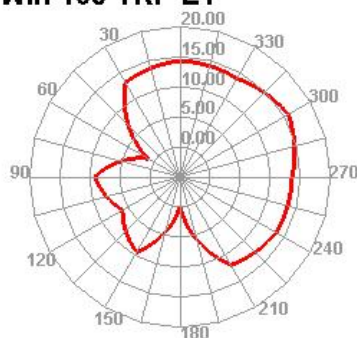
Wifi 165 TRP E1
