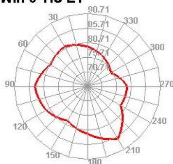
Wifi 6 TIS E1
