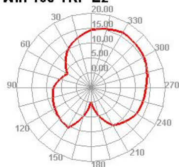
Wifi 165 TRP E2
