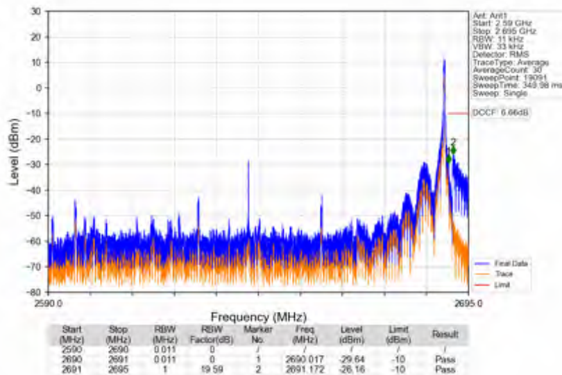
n41 30kHz SISO NTNv 100MHz DFT-s-OFDM QPSK 2640MHz Edge 1RB Right
