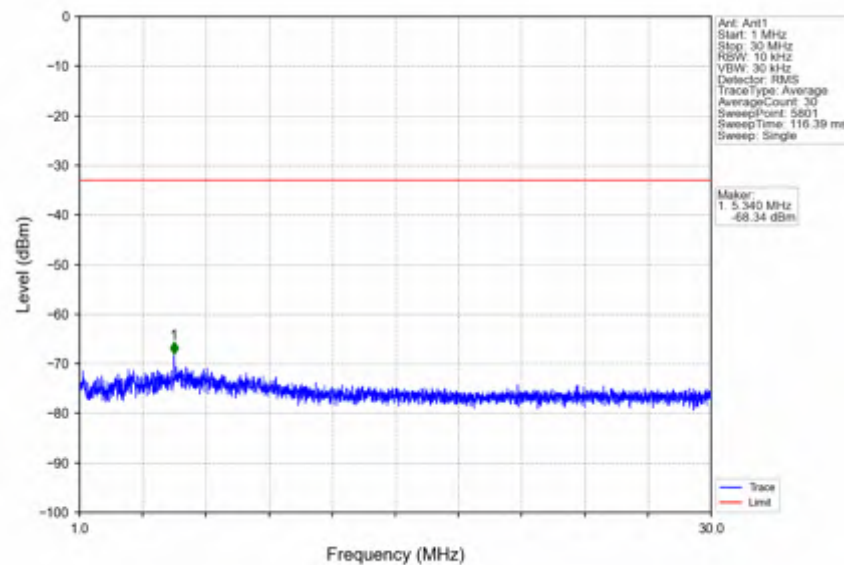
n41_30kHz_SISO_NTNV_90MHz_CP-OFDM_QPSK_2541MHz_Inner_1RB_Left
