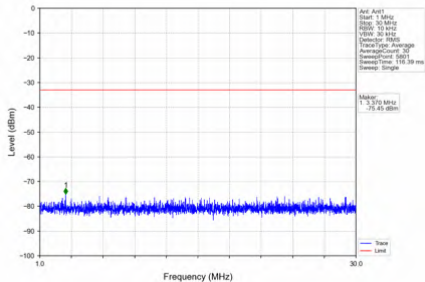
n66_15kHz_SISO_NTV_5MHz_CP-OFDM_QPSK_1712.5MHz_Outer_Full
