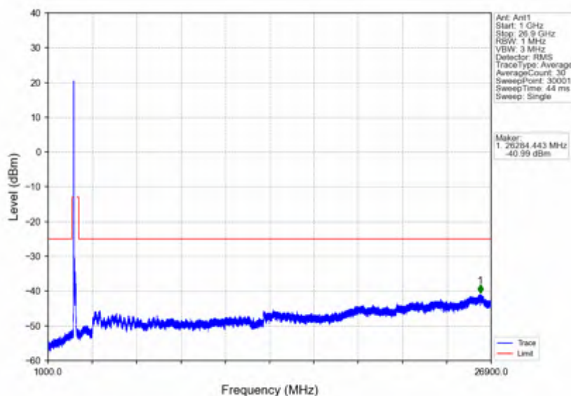
n41 30kHz SISO NTNV 100MHz CP-OFDM QPSK 2592.99MHz Edge 1RB Left
