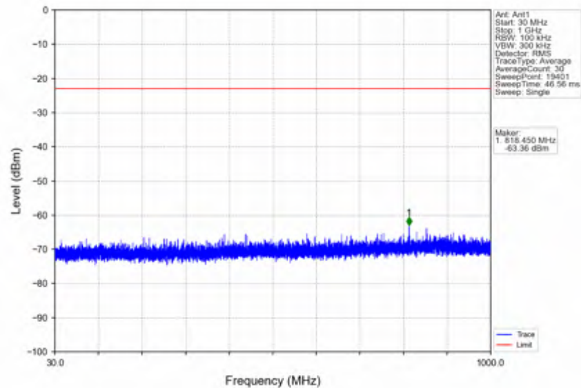
n66_15kHz_SISO_NTNV_10MHz_CP-OFDM QPSK_1775MHz_Inner_1RB_Right
