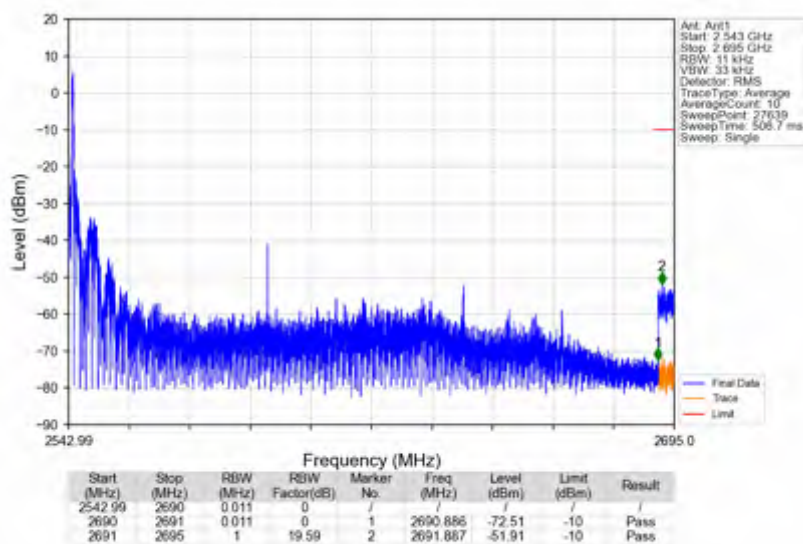
n41 30kHz SISO NTNV 100MHz CP-OFDM QPSK 2592.99MHz Edge 1RB Left
