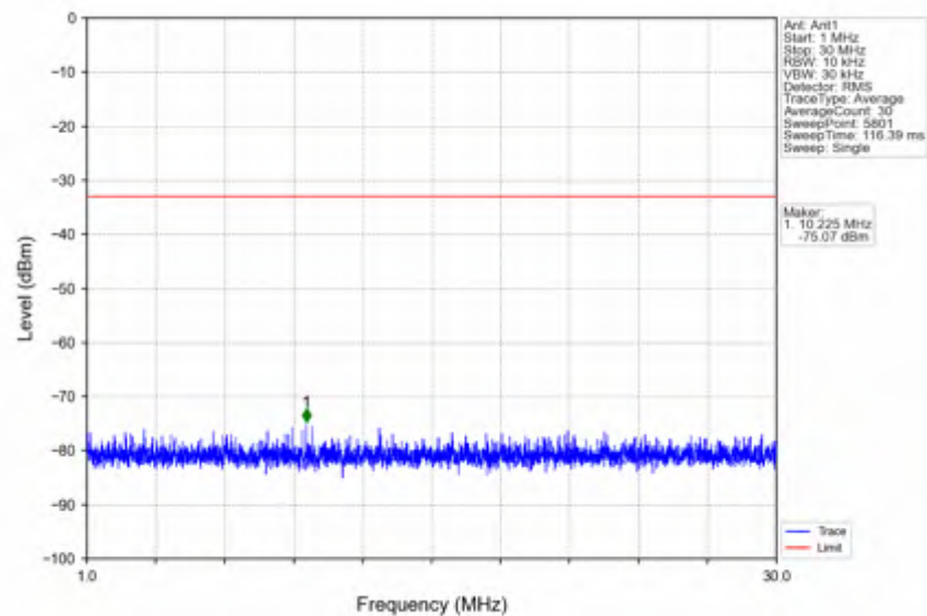
n66_15kHz_SISO_NTNV_10MHz_DFT-s-OFDM_PI/2_BPSK_1775MHz_Inner_1RB_Right
