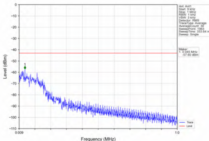
n66_15kHz_SISO_NTNV_10MHz_CP-OFDM QPSK_1775MHz_Inner_1RB_Right
