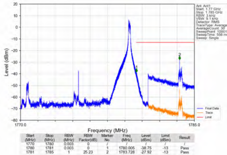
n66_15kHz_SISO_NTNV_10MHz_DFT-s-OFDM PI/2 BPSK_1775MHz_Inner_1RB_Right
