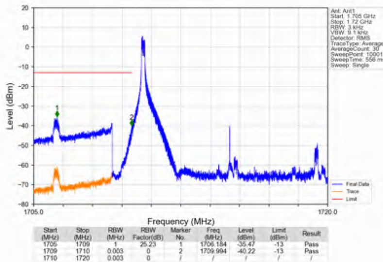
n66_15kHz_SISO_NTNV_10MHz_DFT-s-OFDM QPSK_1715MHz_Inner_1RB_Left
