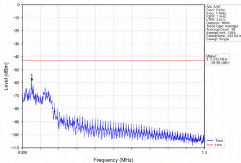
n66_15kHz_SISO_NTNV_10MHz_DFT-s-OFDM PI/2 BPSK_1775MHz_Inner_1RB_Right
