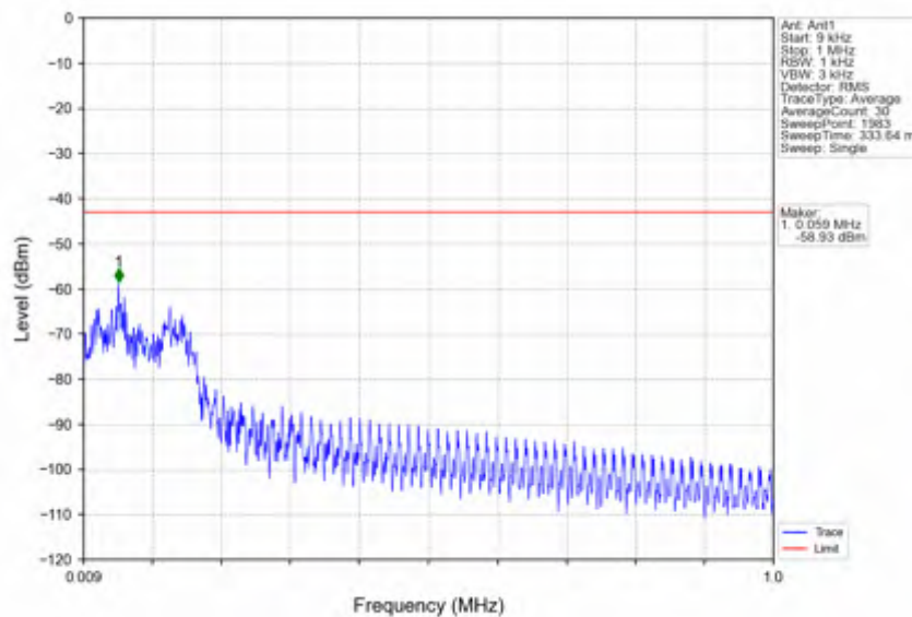
n66 15kHz SISO NTNV 10MHz DFT-s-OFDM PI/2 BPSK 1715MHz Inner 1RB Left
