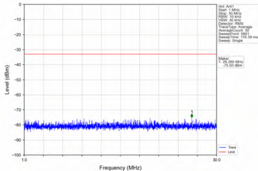
n66_15kHz_SISO_NTNV_5MHz_CP-OFDM QPSK_1712.5MHz_Inner_1RB_Left
