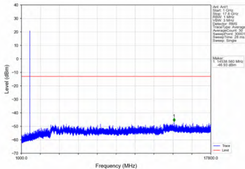
n66 15kHz SISO NTN 5MHz CP-OFDM QPSK 1745MHz Edge 1RB Left
