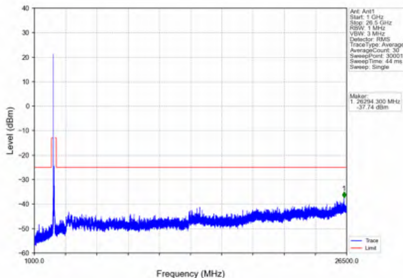
n41 30kHz SISO NTNv 100MHz DFT-s-OFDM QPSK 2640MHz Edge 1RB Right
