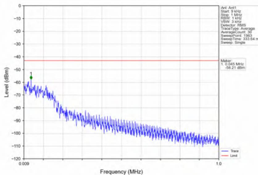
n66_15kHz_SISO_NTNV_5MHz_CP-OFDM QPSK_1712.5MHz_Inner_1RB_Left
