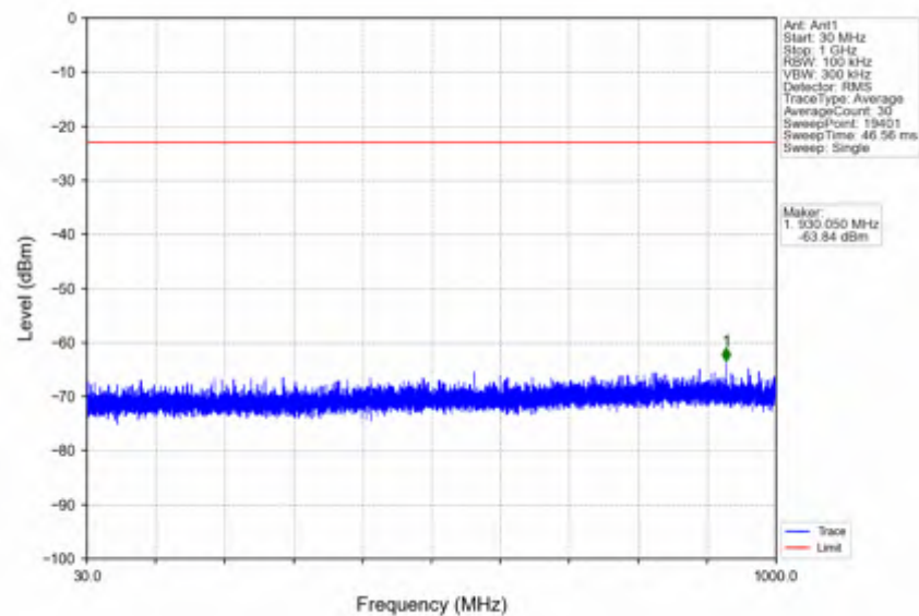
n66_15kHz_SISO_NTNV_10MHz_DFT-s-OFDM_PI/2_BPSK_1775MHz_Inner_1RB_Right
