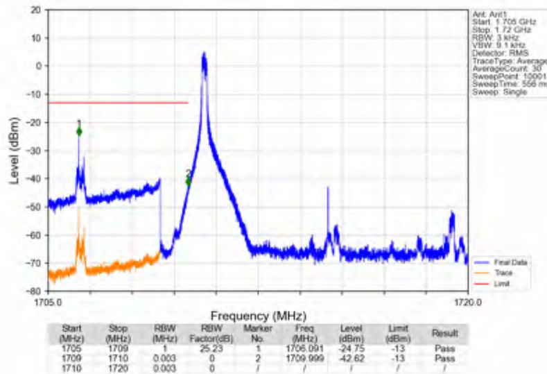
n66_15kHz_SISO_NTNV_10MHz_DFT-s-OFDM_PI/2_BPSK_1715MHz_Inner_1RB_Left
