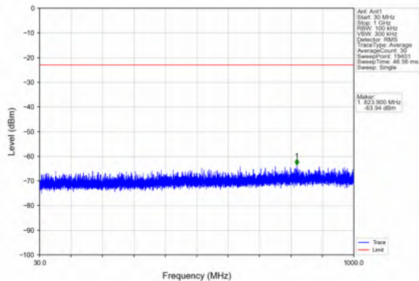
n66 15kHz SISO NTN 5MHz CP-OFDM QPSK 1745MHz Edge 1RB Left
