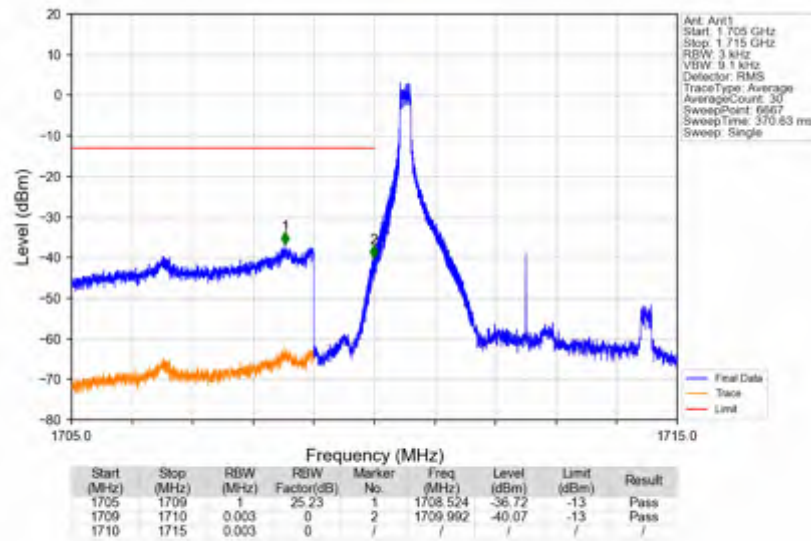
n66_15kHz_SISO_NTNV_5MHz_CP-OFDM QPSK_1712.5MHz_Inner_1RB_Left
