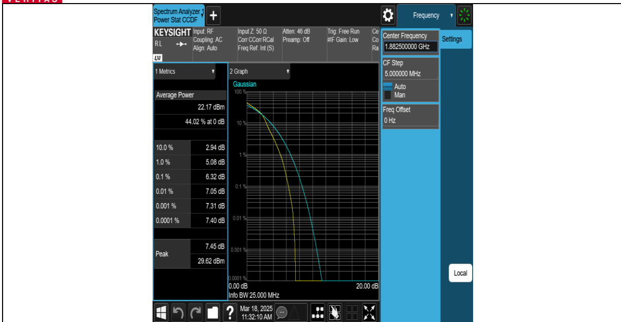
Band25-20MHz-16QAM-26365-27RB#0-PASS
